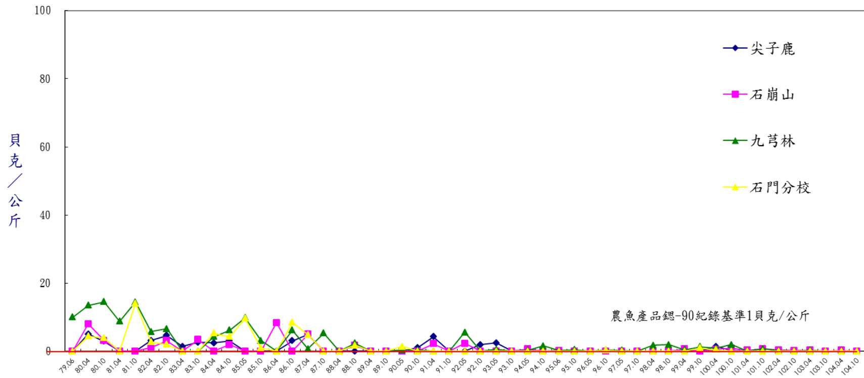
圖16 核能一廠茶葉鋇-90活度歷年分析結果
