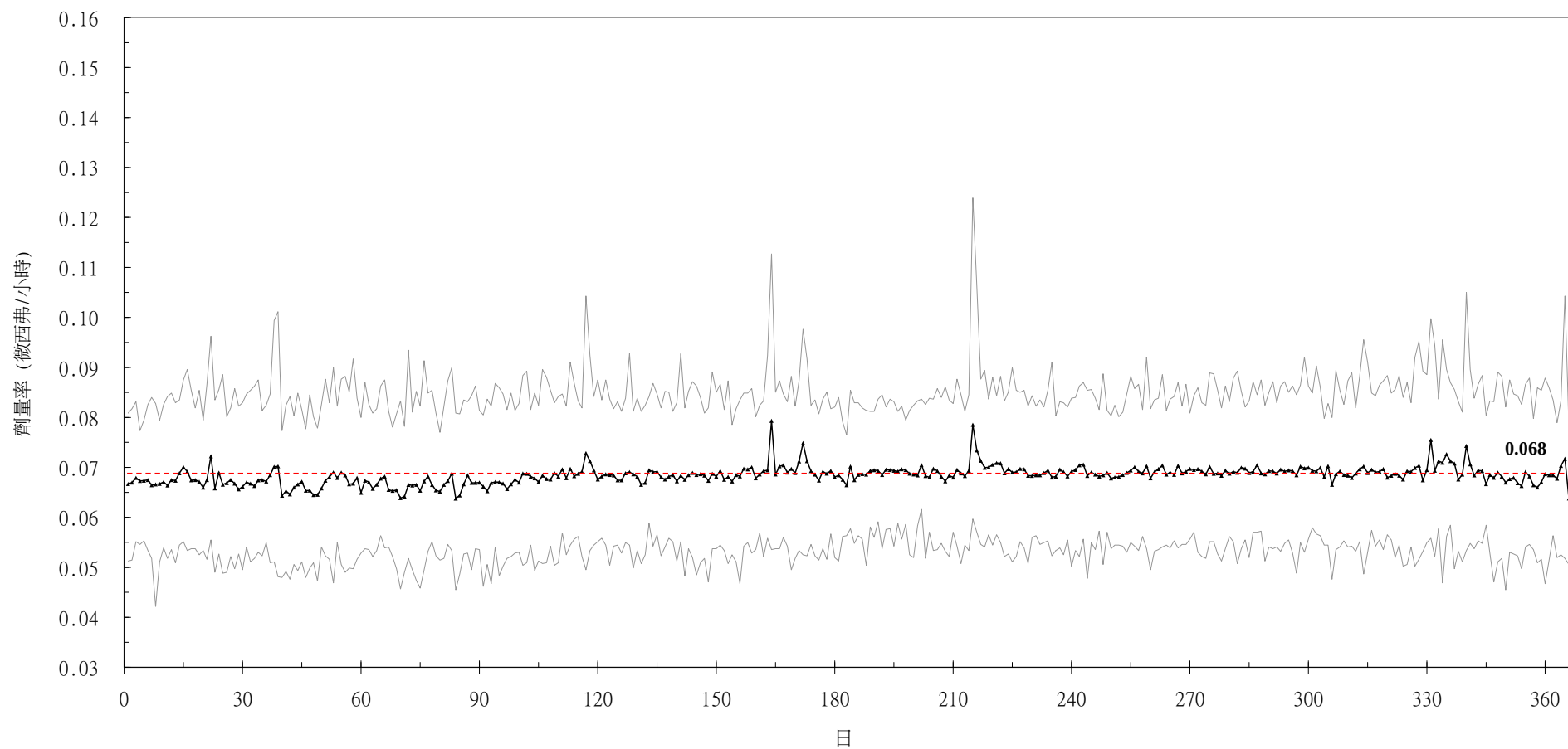
圖4 101年連續輻射偵測劑量率變動圖(原科中心)
