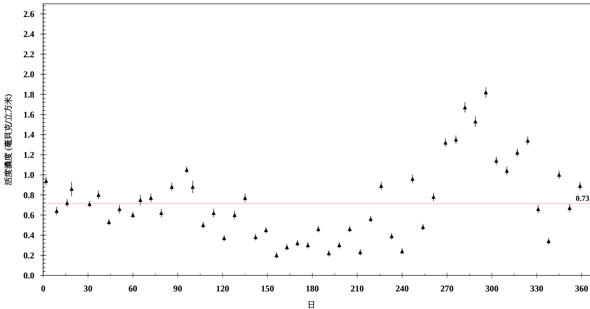
圖6 101年空浮微粒活度濃度變動圖(原科中心)
