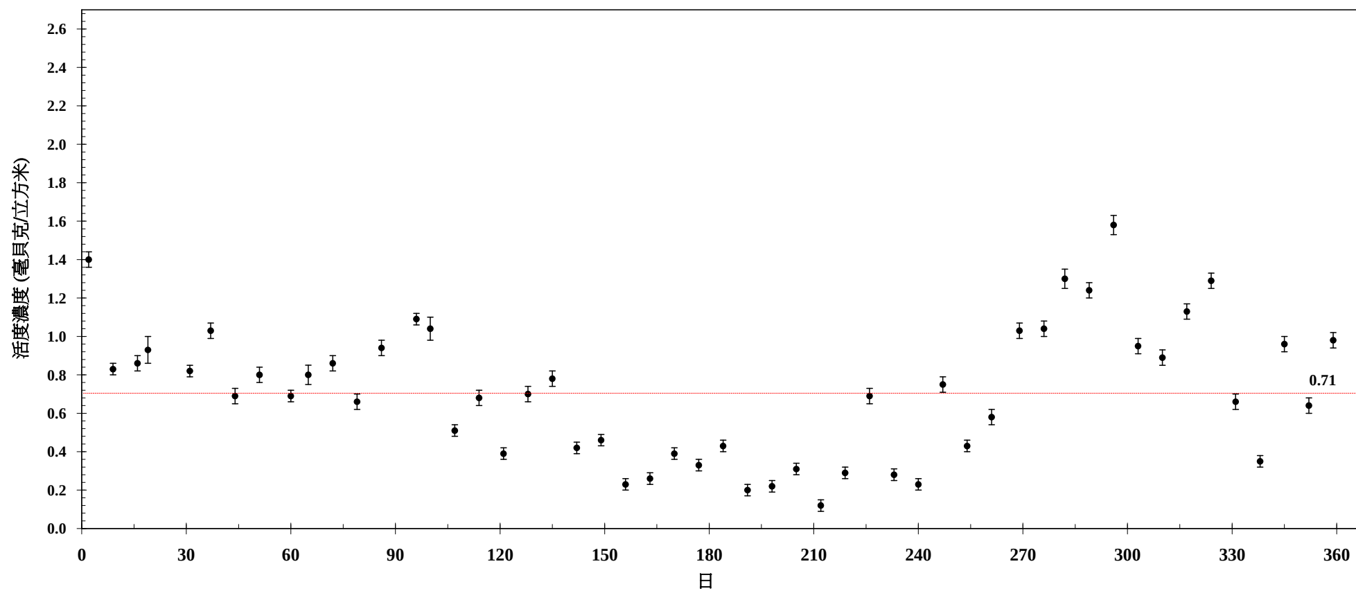
圖7 101年空浮微粒活度濃度變動圖(速器館側)
