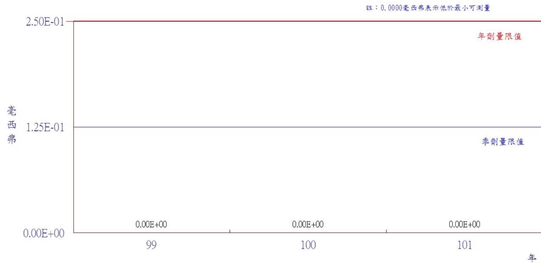
圖5 蘭嶼貯存場101年民眾最大個人全身劑量
