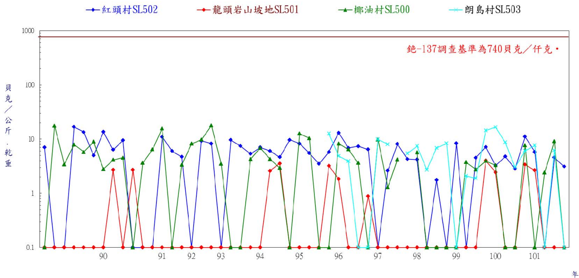
圖3 蘭嶼貯存場土壤鈉-137加馬能譜分析結果
