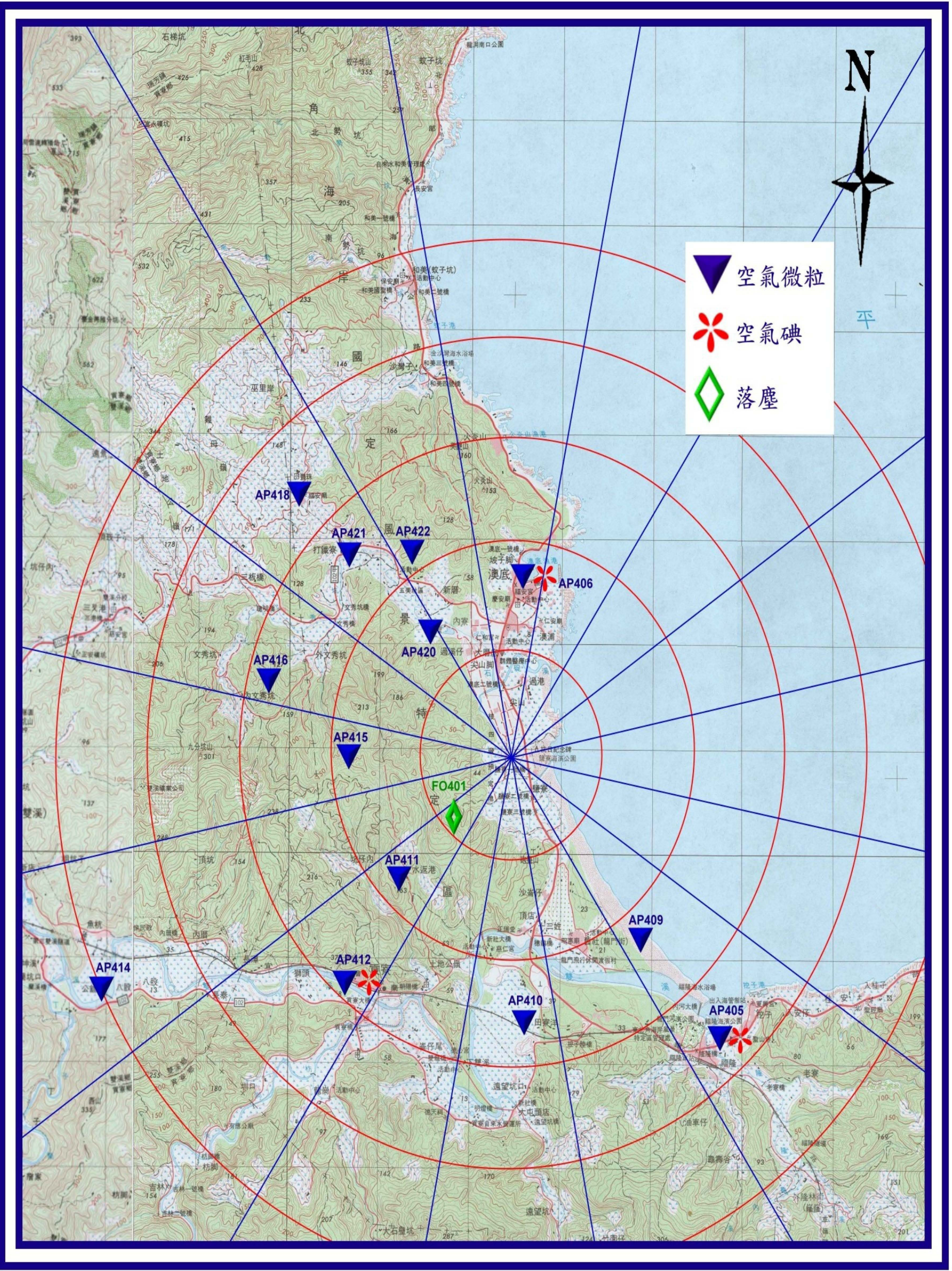
圖4 核能四廠空氣微粒取樣站分佈圖(5公里內)
