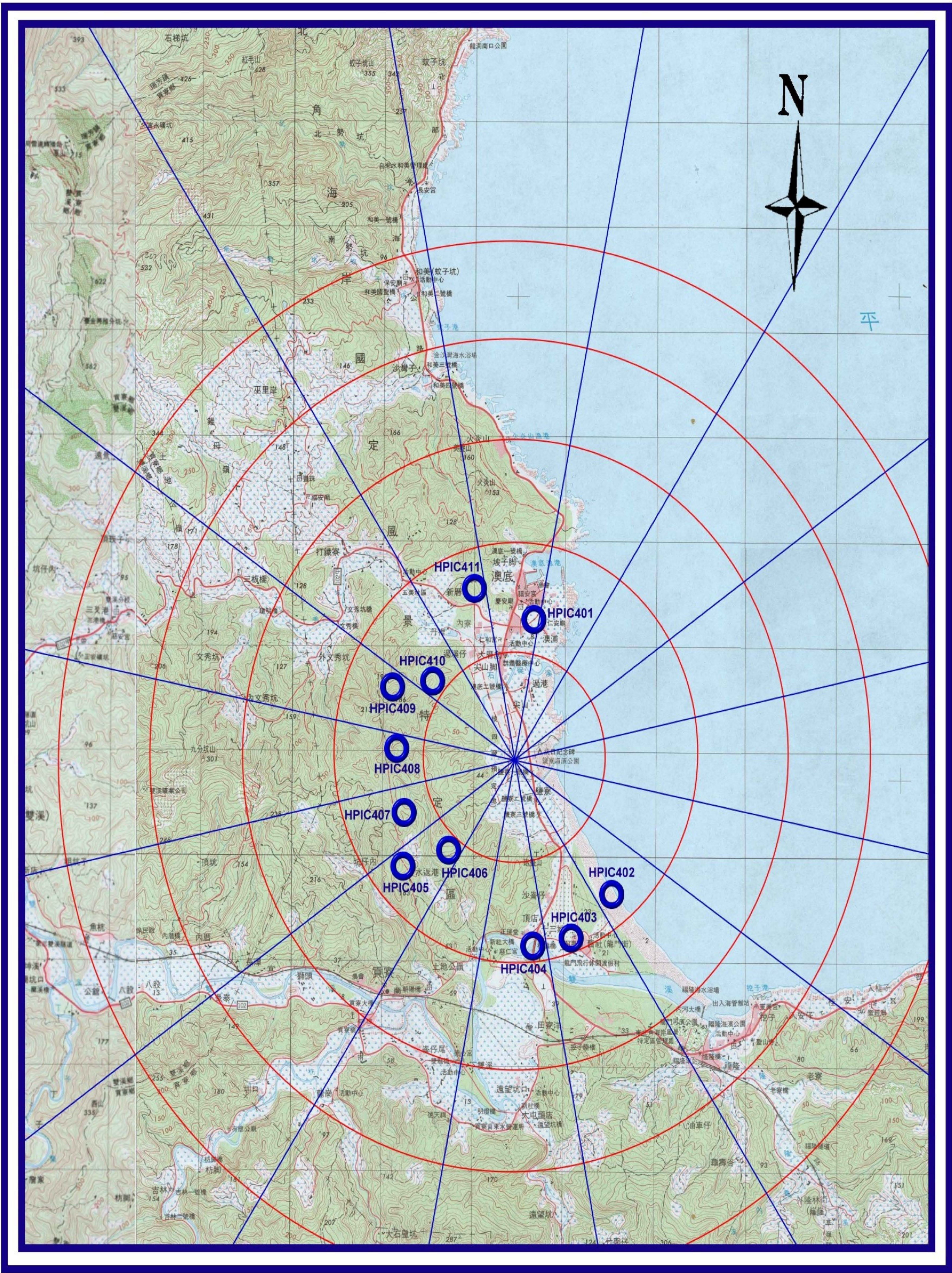
圖3 核能四廠高壓游離腔監測站分佈圖
