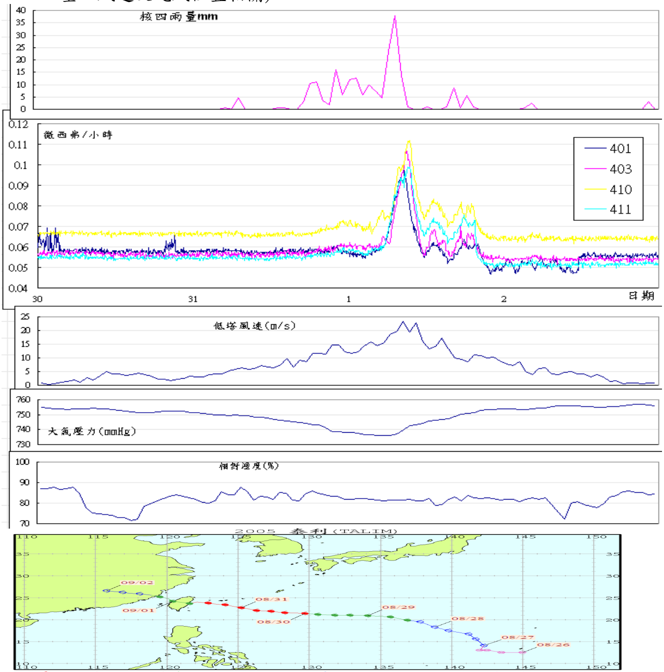
泰利颱風(94. 08. 30至09. 02)侵颱期間劑量率、降雨量、風速及颱風路徑變化
