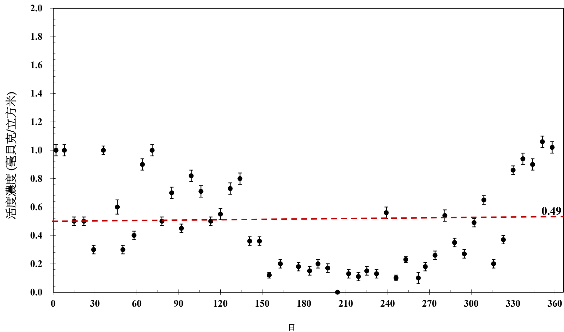
圖7 113年空浮微粒活度濃度變動圖(加速器館)
