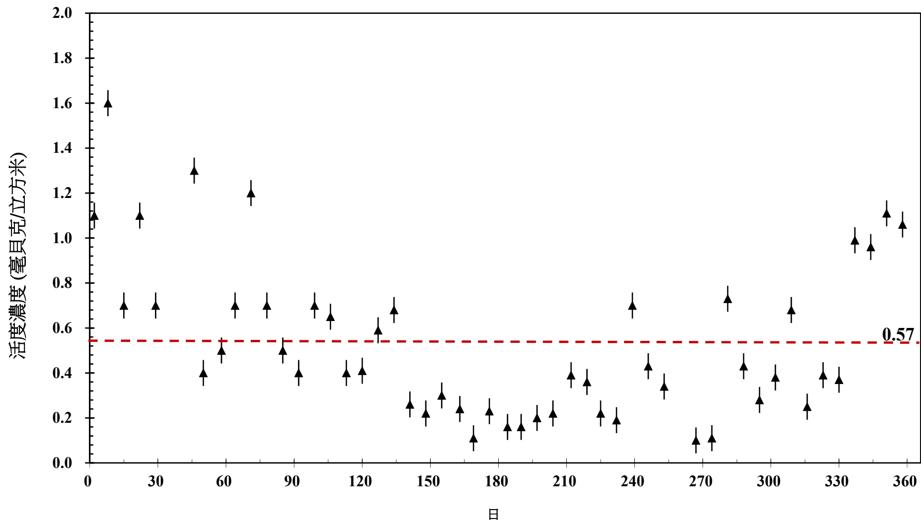
圖6 113年空浮微粒活度濃度變動圖(李存敏館)
