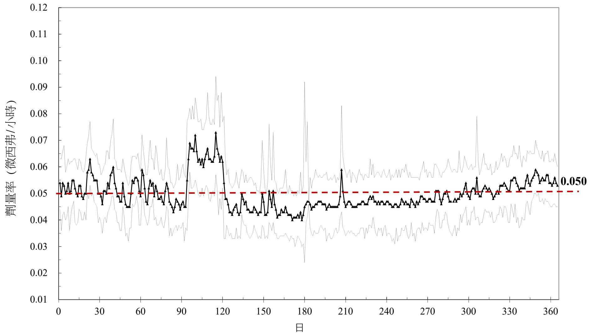
圖 4 113 年連續輻射偵測劑量率變動圖(李存敏館)
