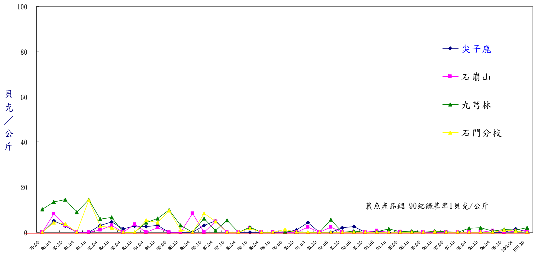
圖16 核能一廠茶葉銇-90活度歷年分析結果
