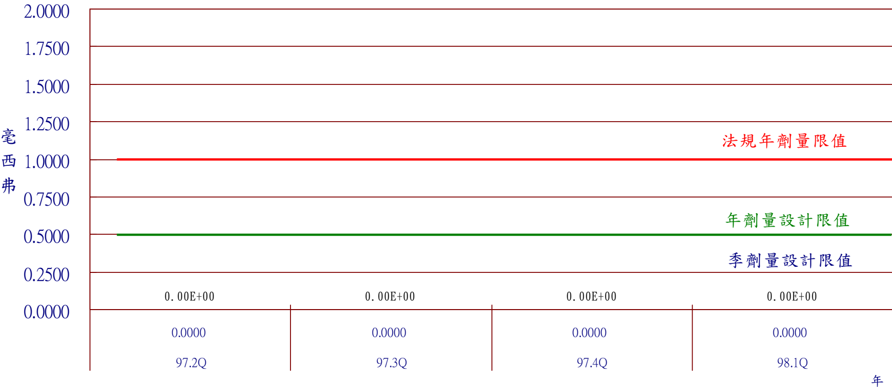
圖17 核能三廠98年第1季民眾最大個人全身劑量
