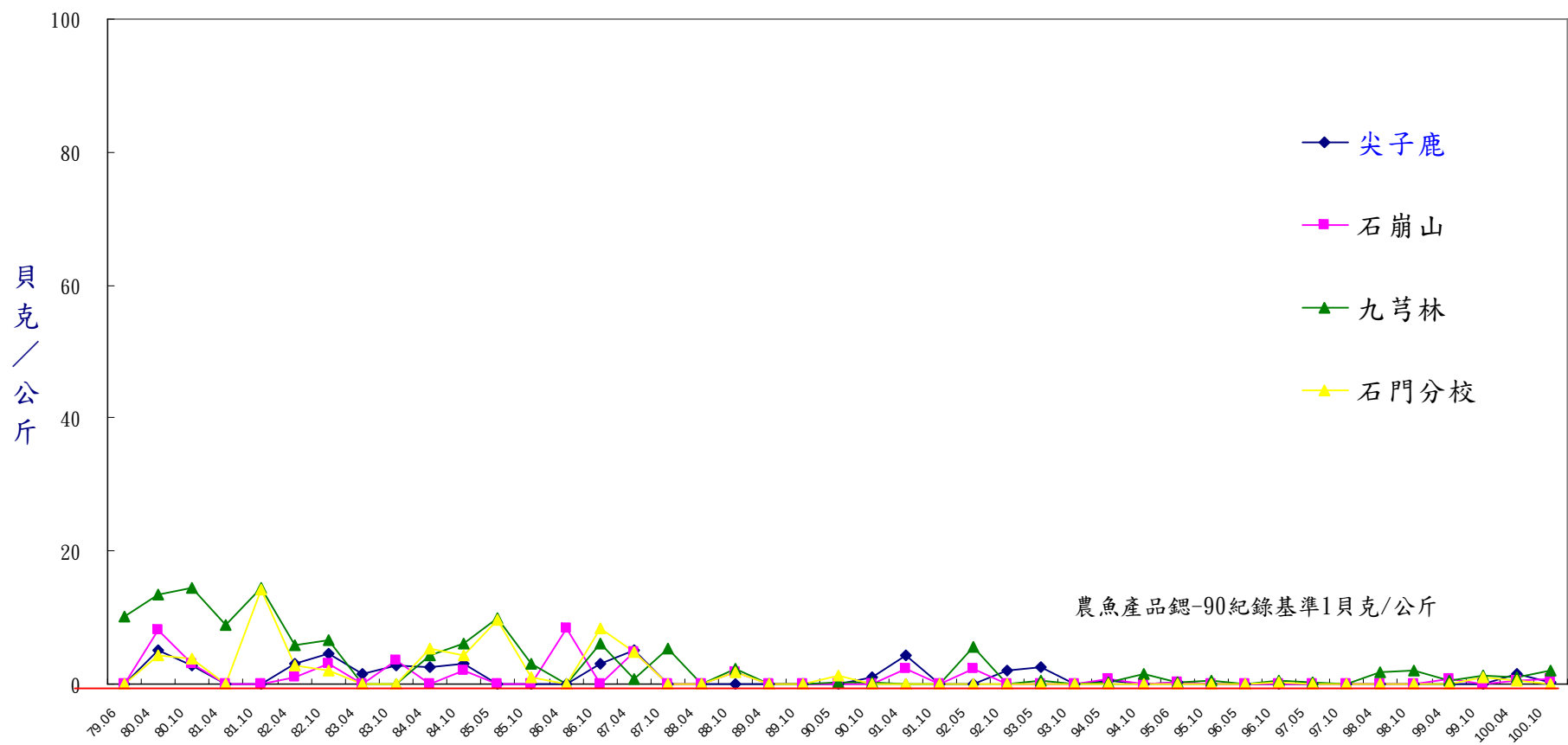
圖16 核能一廠茶葉 90 Sr活度歷年分析結果
