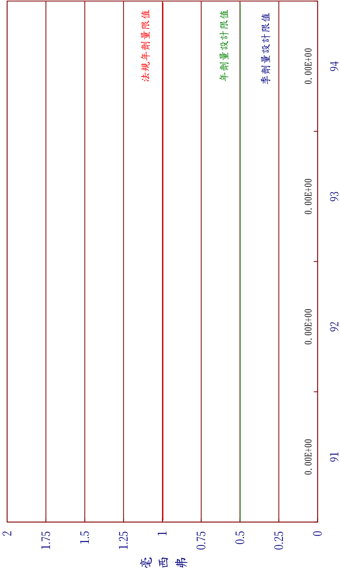
圖19 核能三廠94年民眾最大個人全身劑量
