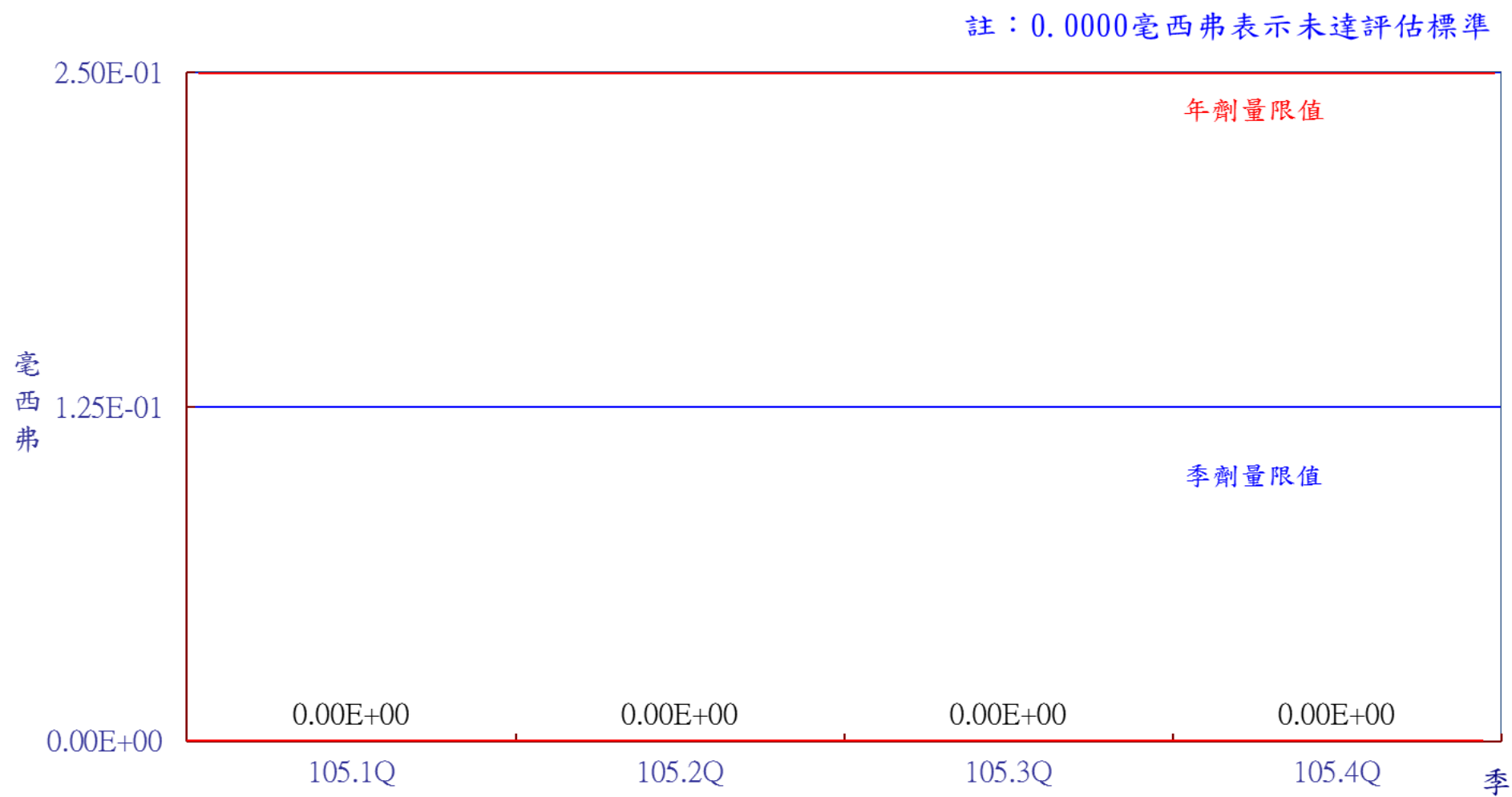
圖5 蘭嶼貯存場105年第4季民眾最大個人全身劑量
