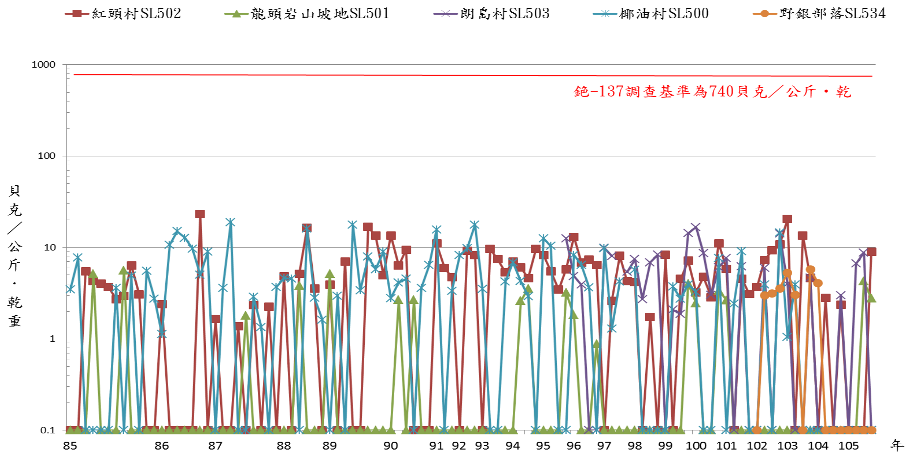
圖3 蘭嶼貯存場土壤鉍-137加馬能譜分析結果
