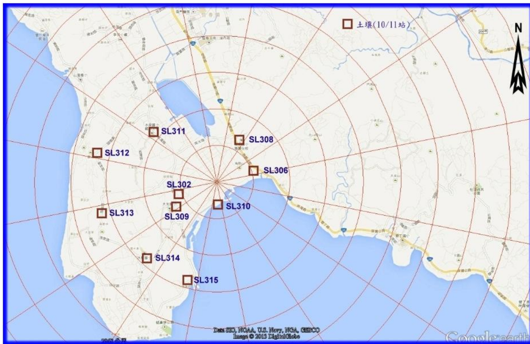
圖 9 核能三廠土壤取樣站分佈圖(5 公里內)
