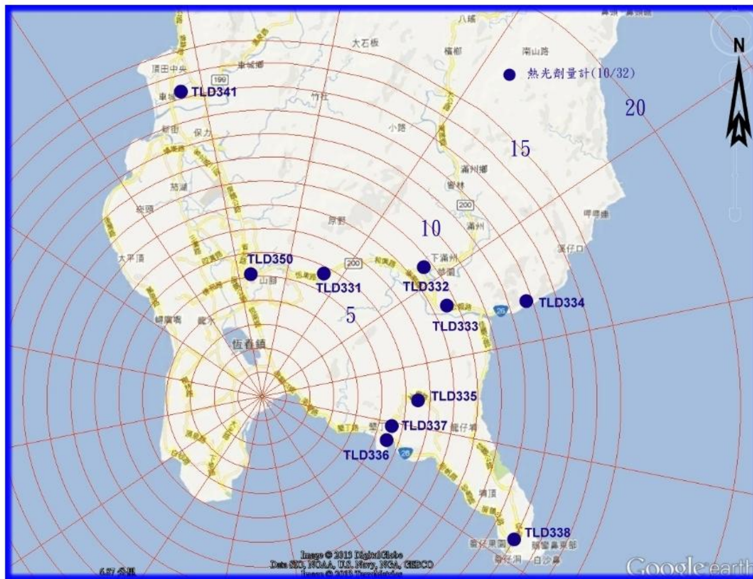
圖 2 核能三廠熱發光劑量計監測站分佈圖(5 公里外)
