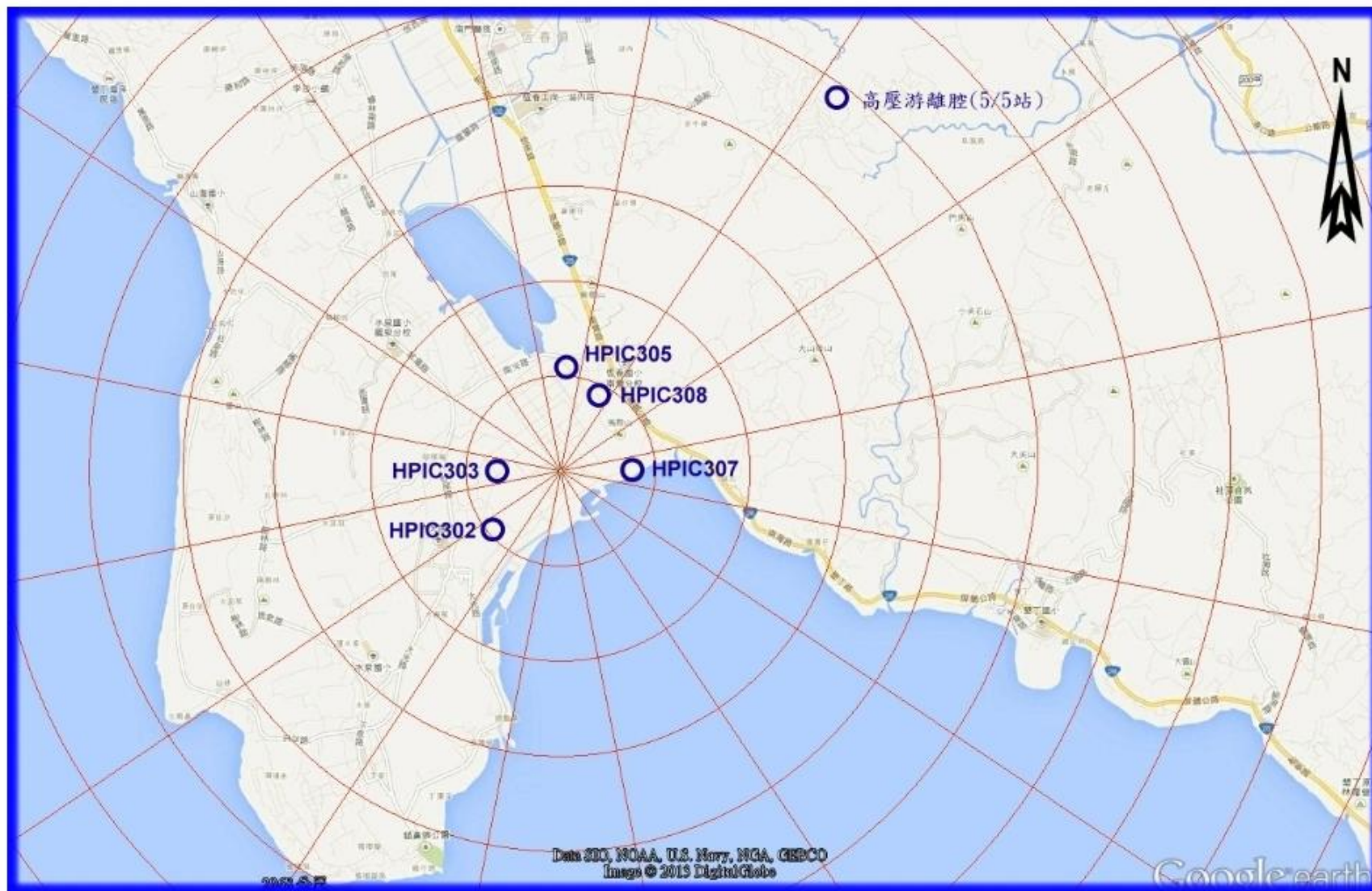
圖 3 核能三廠高壓游離腔監測站分佈圖
