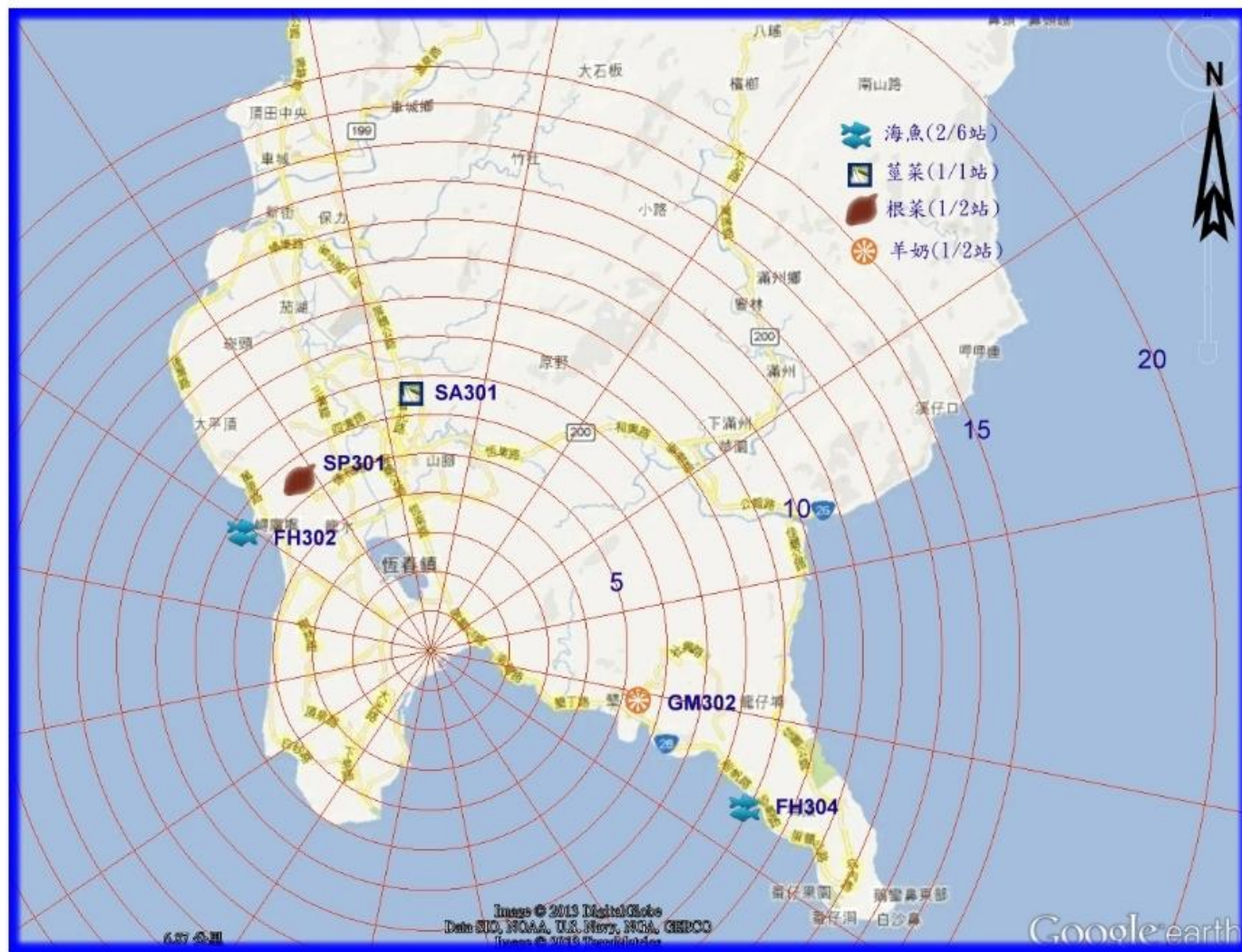
圖 8 核能三廠各類生物樣取樣站分佈圖(5 公里外)
