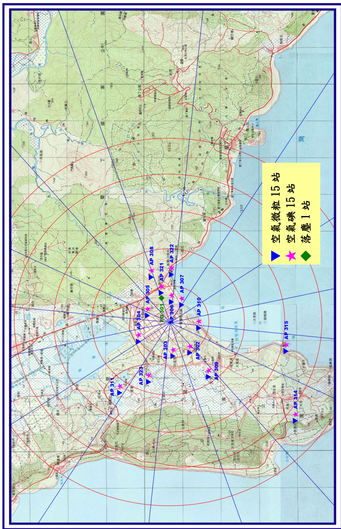
圖 4 核能三廠空氣微粒取樣站分佈圖
