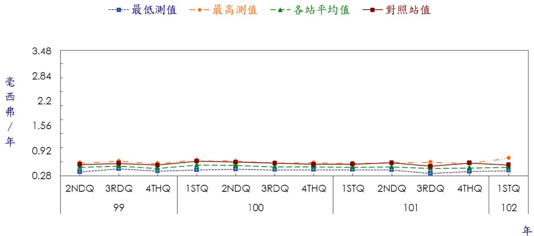
圖14 核能三廠環境熱發光劑量計監測結果
