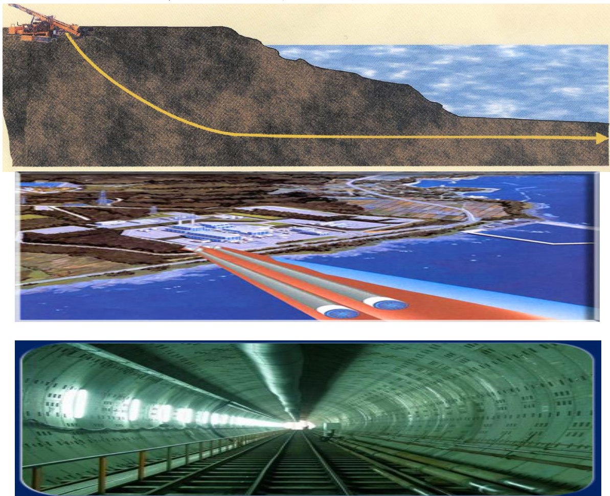
核能四廠出水口潛盾隧道設計及完工圖
