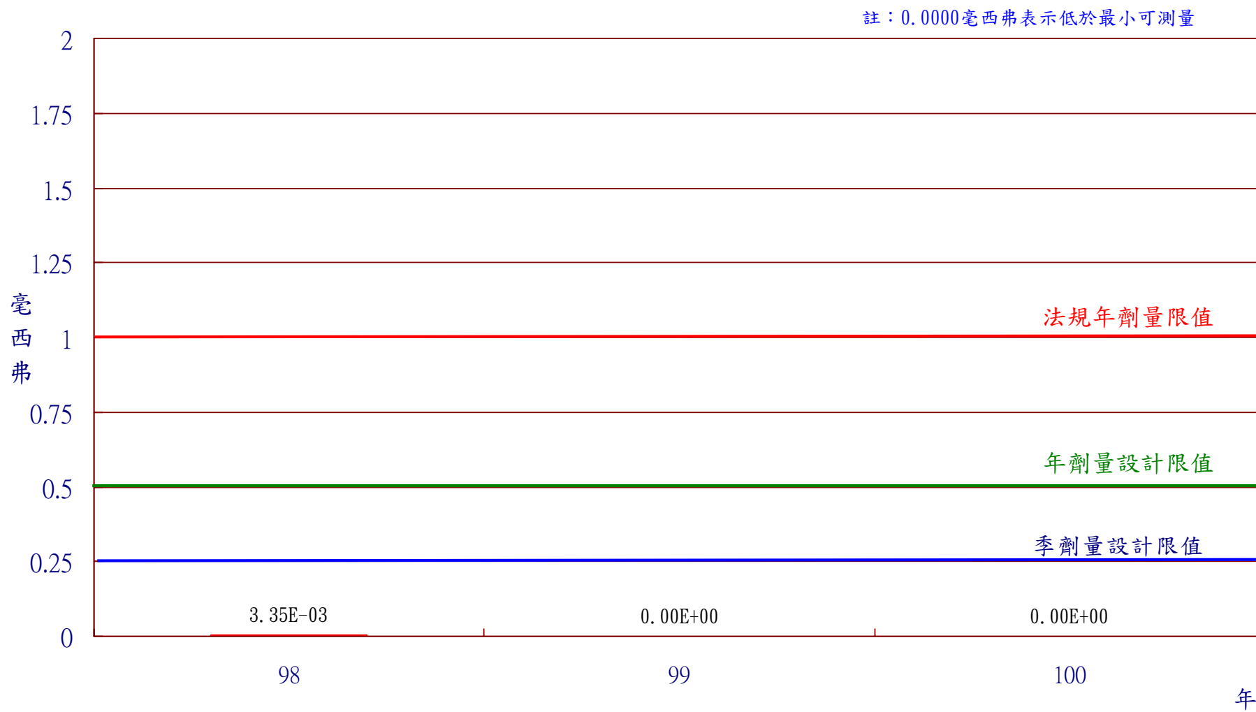
圖16 核能二廠100年民眾最大個人全身劑量
