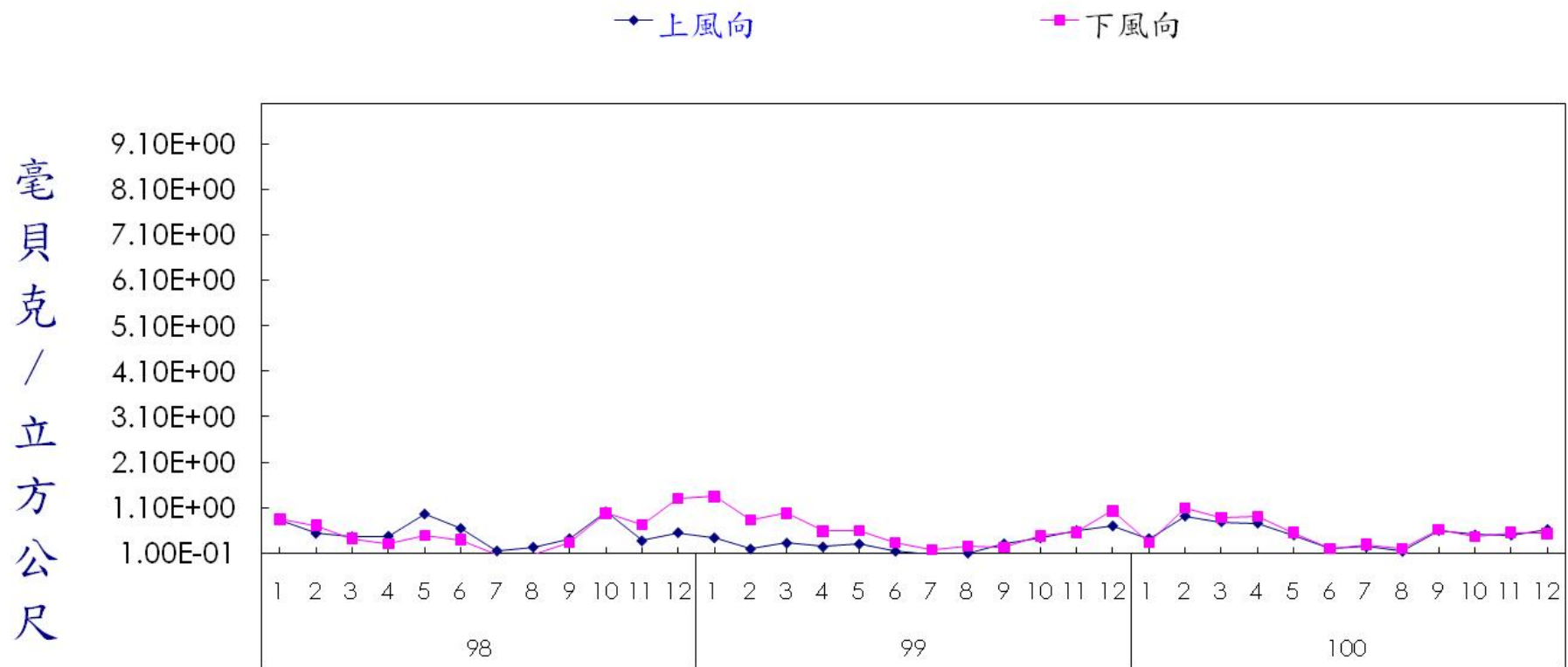
圖 14 核能二廠上下風向空氣微粒總貝他活度監測結果 年
