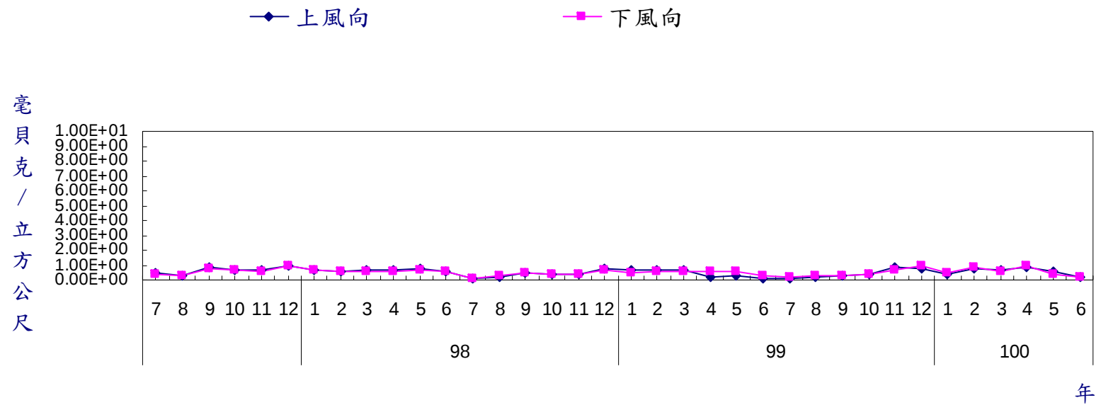
圖 15 核能三廠上下風向空氣微粒總貝他活度監測結果
