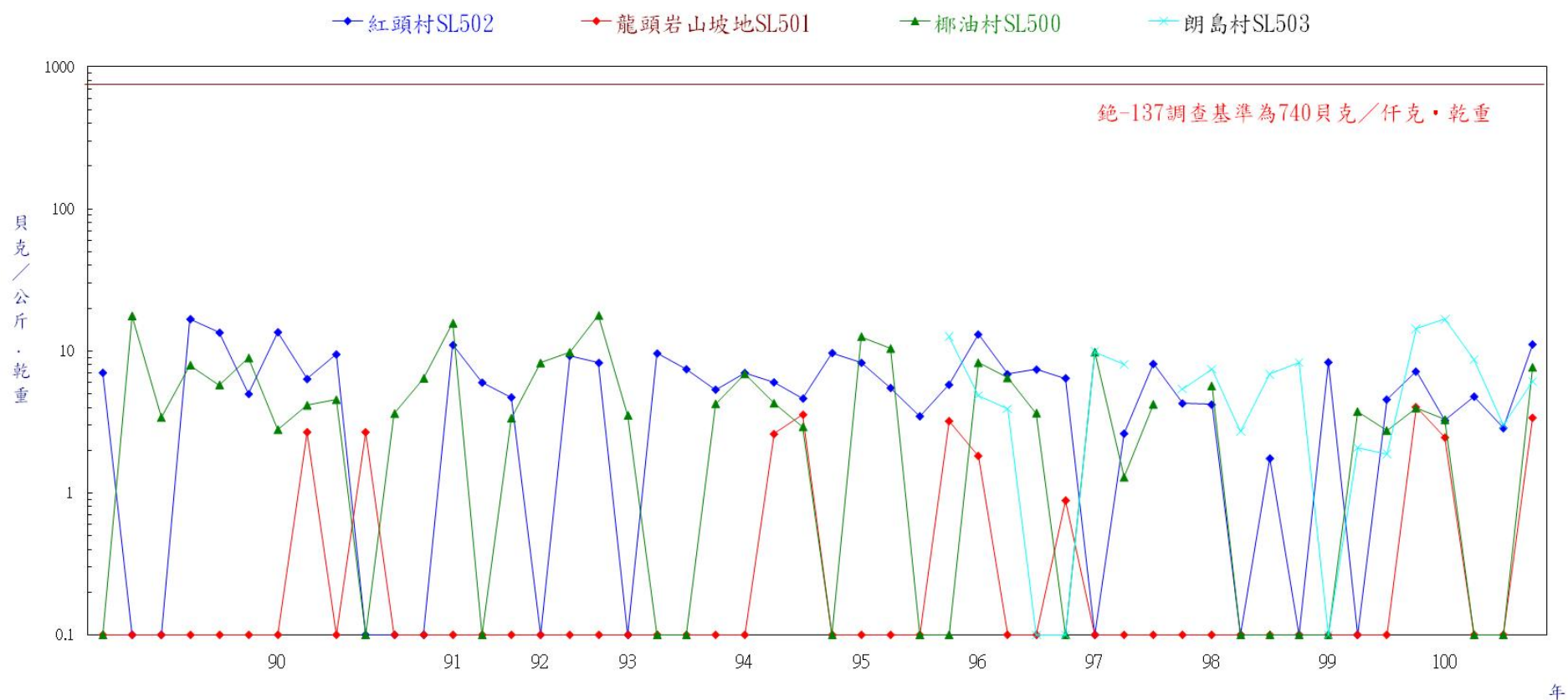
圖3 蘭嶼貯存場土壤鈷-137加馬能譜分析結果
