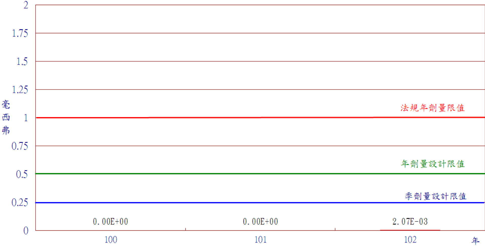
圖16 核能二廠102年民眾最大個人全身劑量
