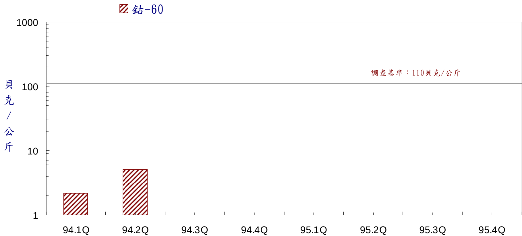
圖 15 核能二廠出水口附近排水涵管下方岸沙加馬能譜監測結果
