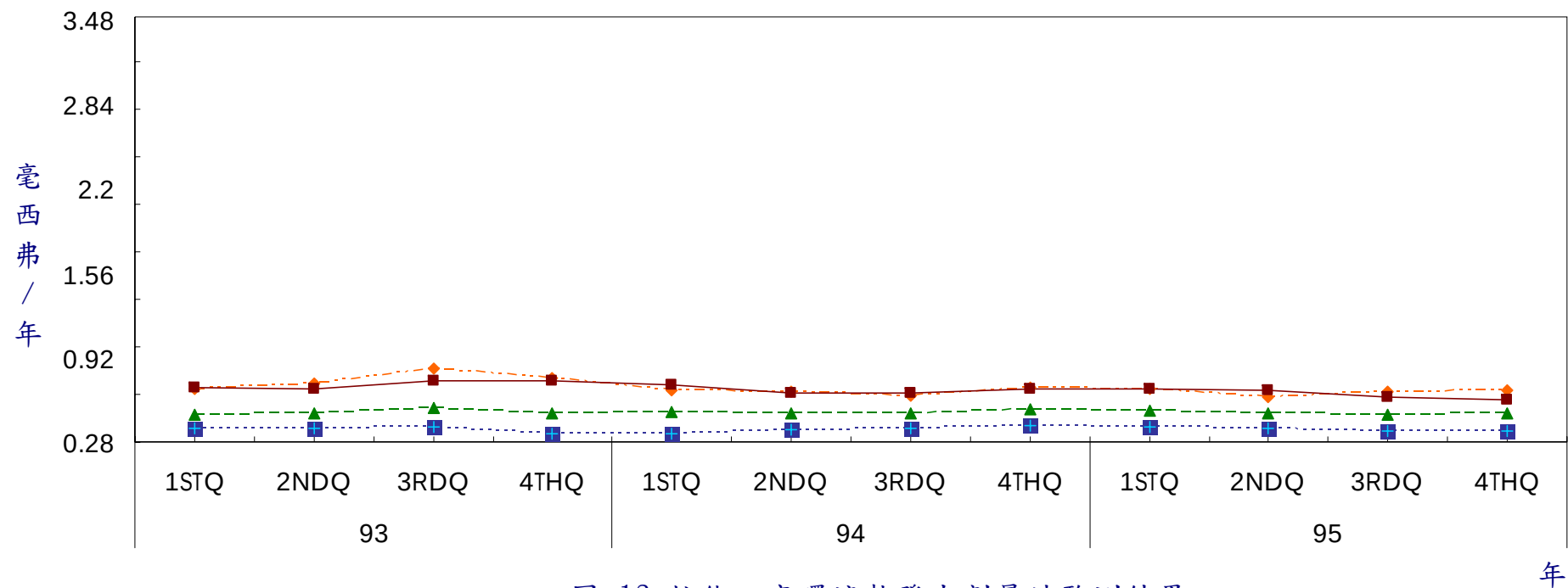
圖 13 核能二廠環境熱發光劑量計監測結果
