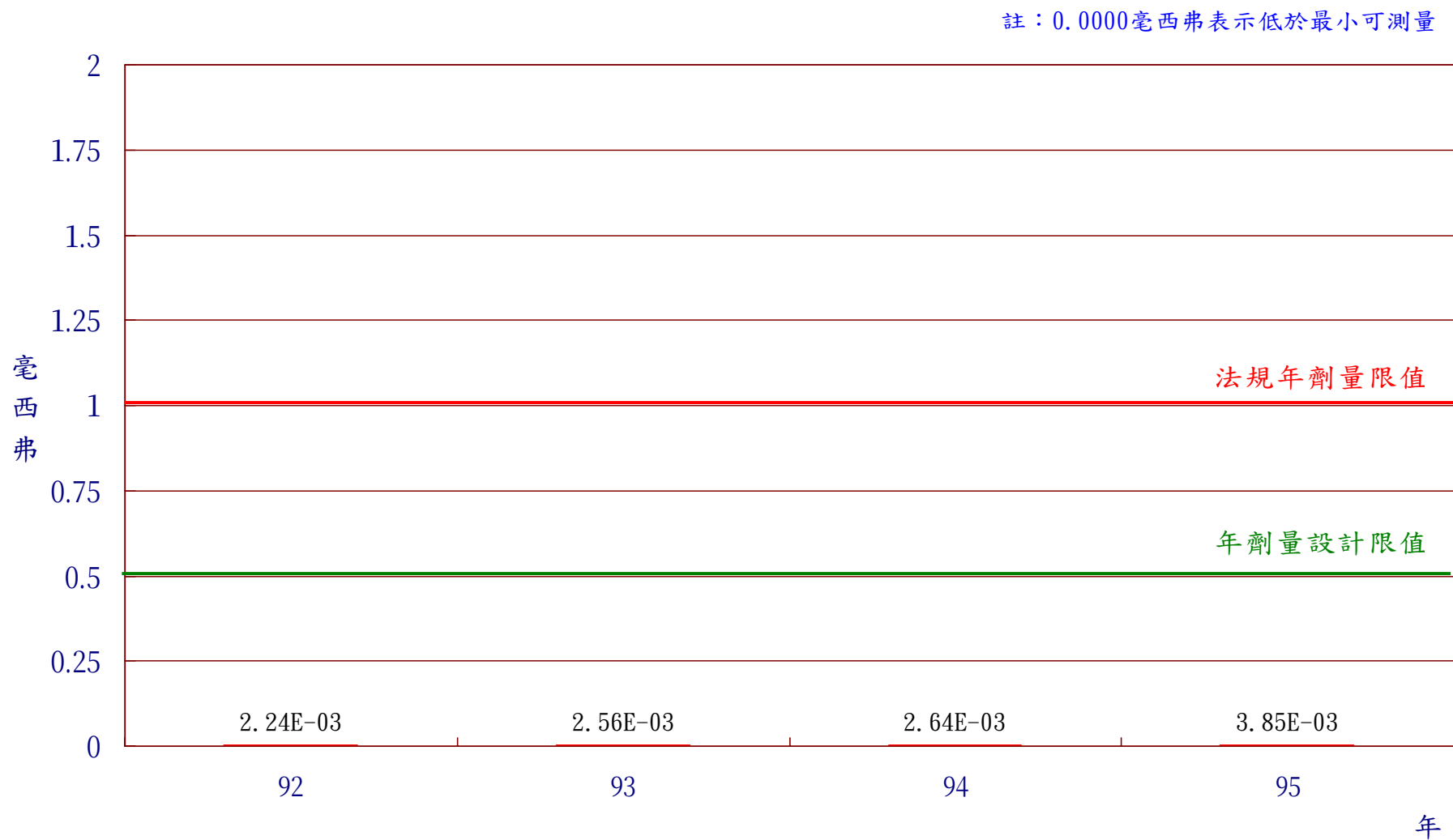
圖16 核能二廠95年民眾最大個人全身劑量
