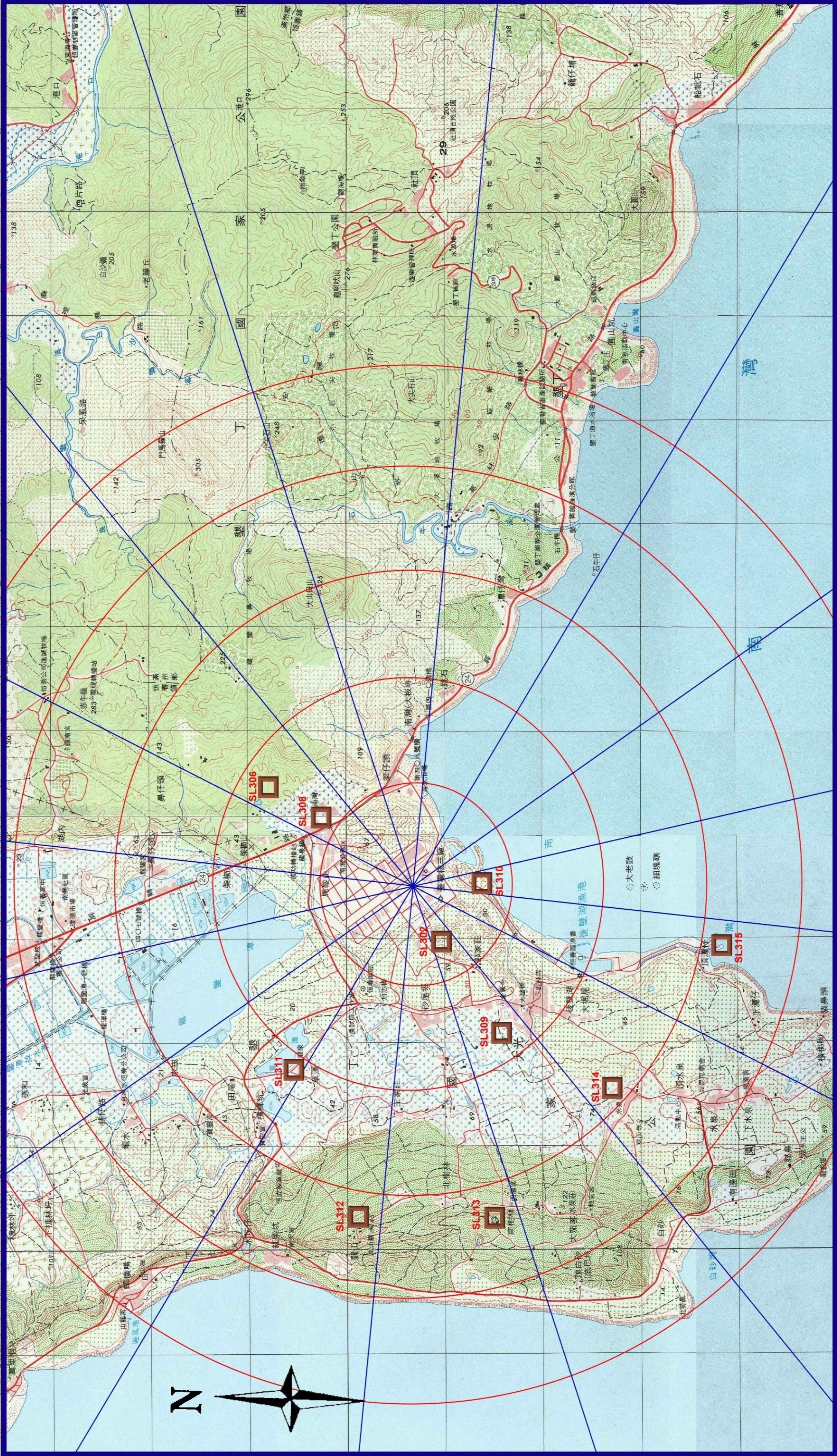
圖10 核能三廠土壤取樣站分佈圖(5公里內)
