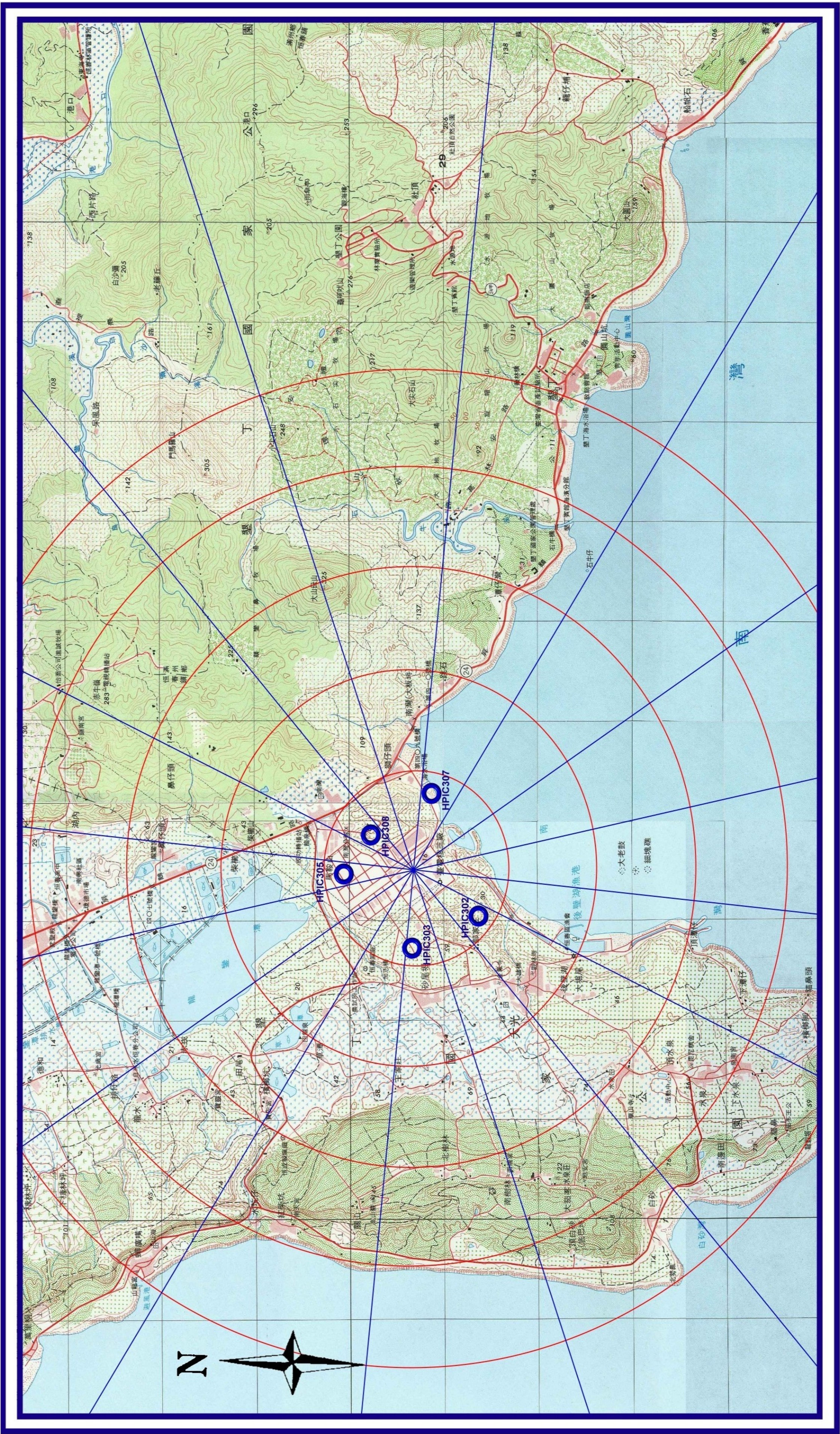
圖3 核能三廠高壓游離腔監測站分佈圖
