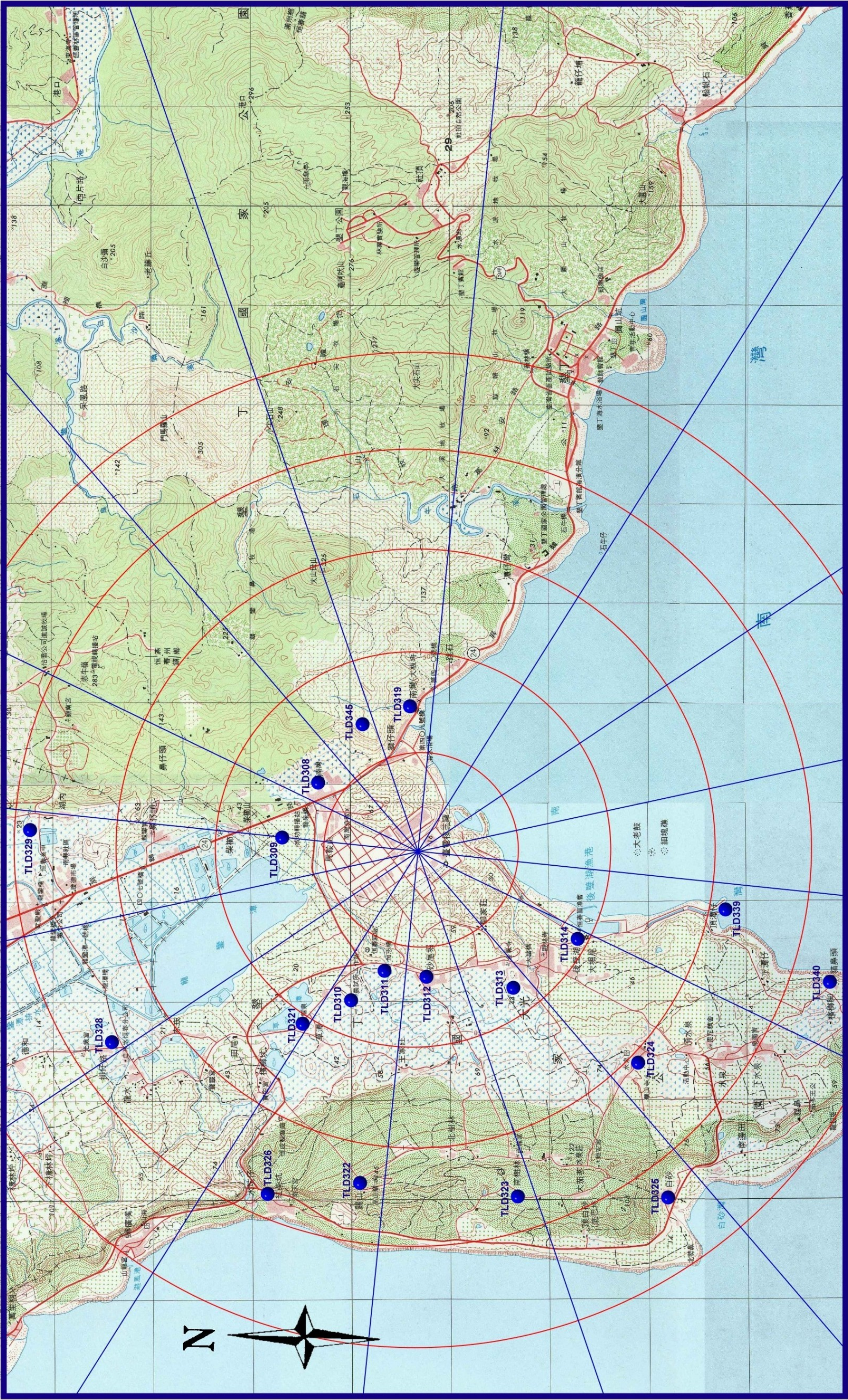
圖1 核能三廠熱發光劑量計監測站分佈圖(5公里內)
