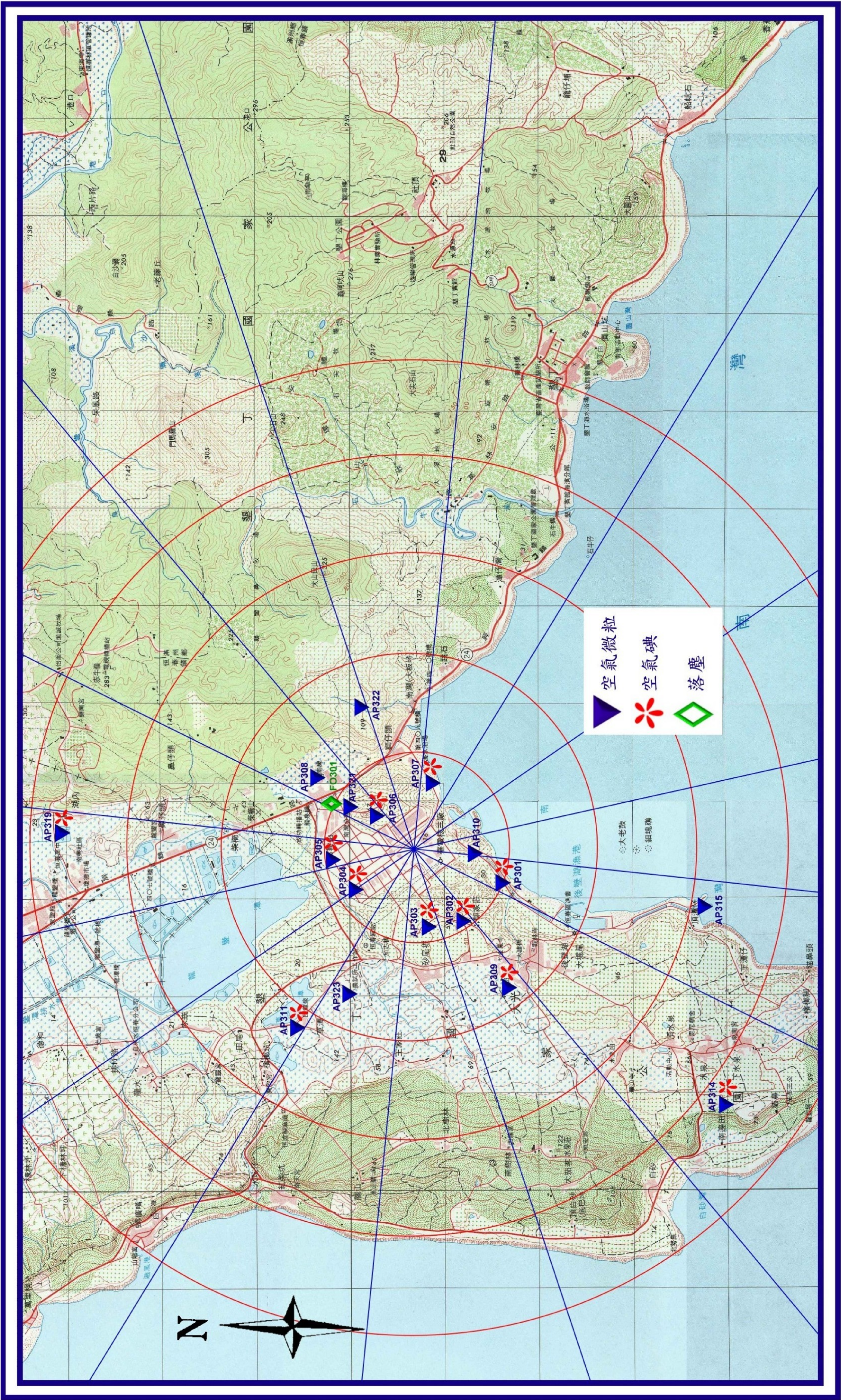
圖4 核能三廠空氣微粒取樣站分佈圖(5公里內)
