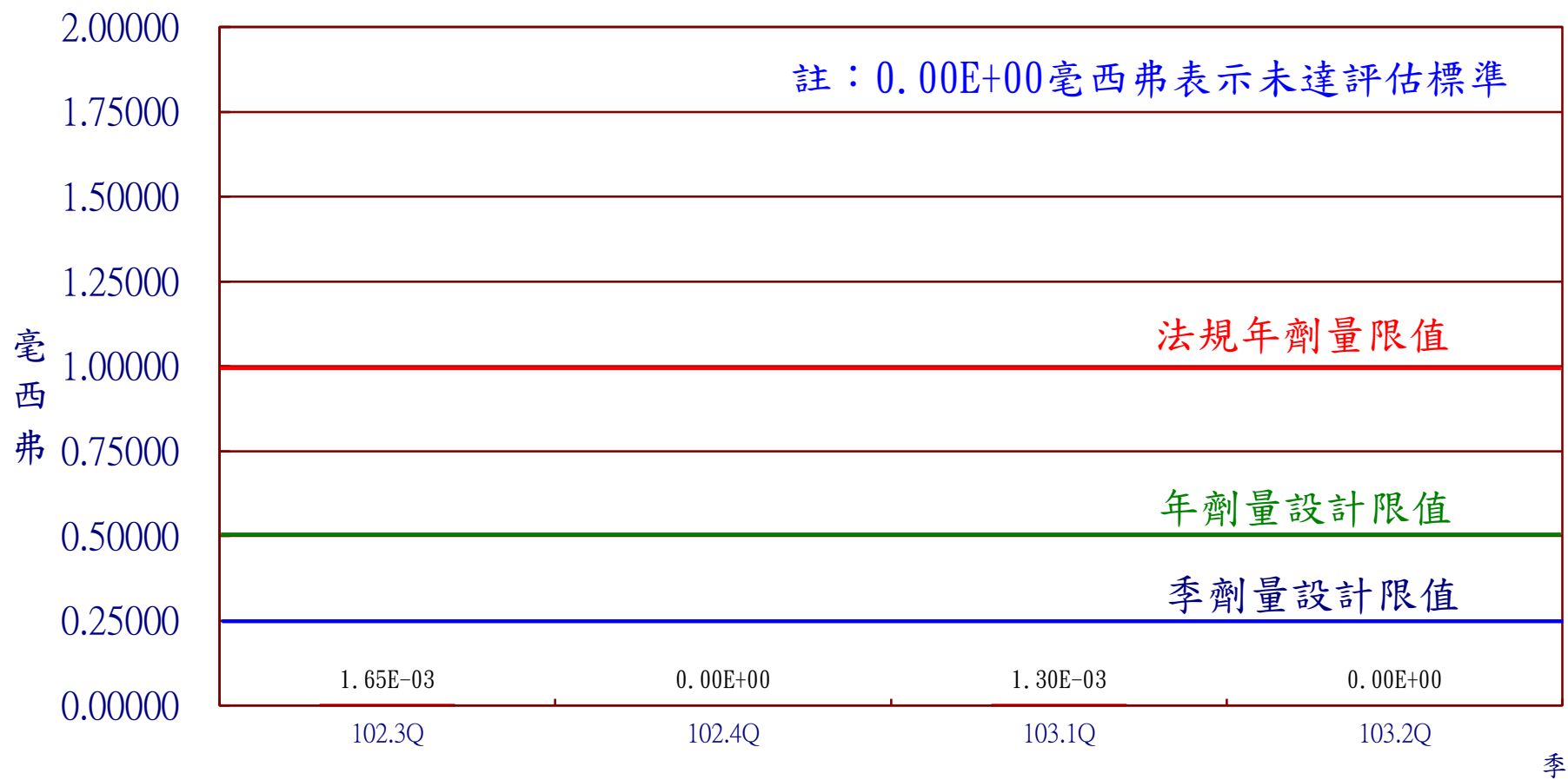
圖18 核能一廠103年第2季民眾最大個人全身劑量
