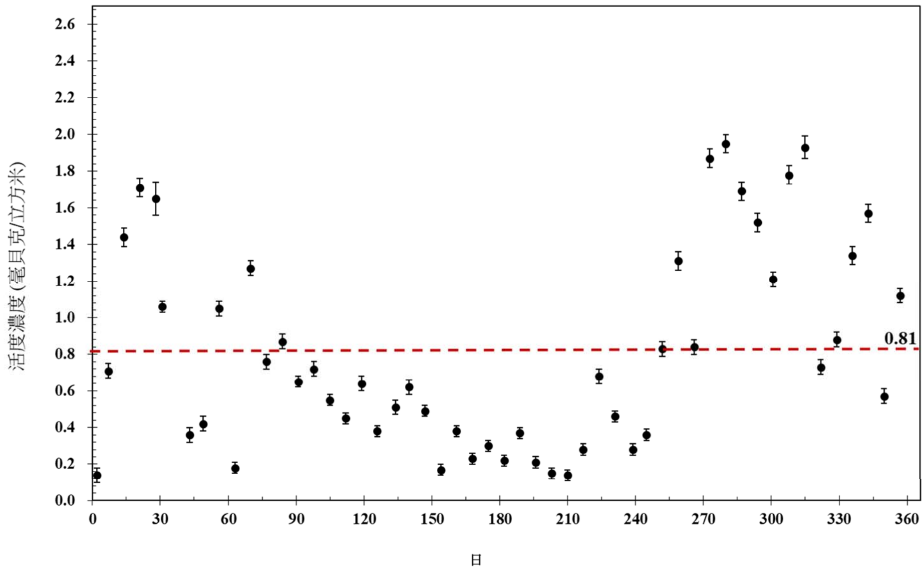
圖7 108年空浮微粒活度濃度變動圖(加速器館)
