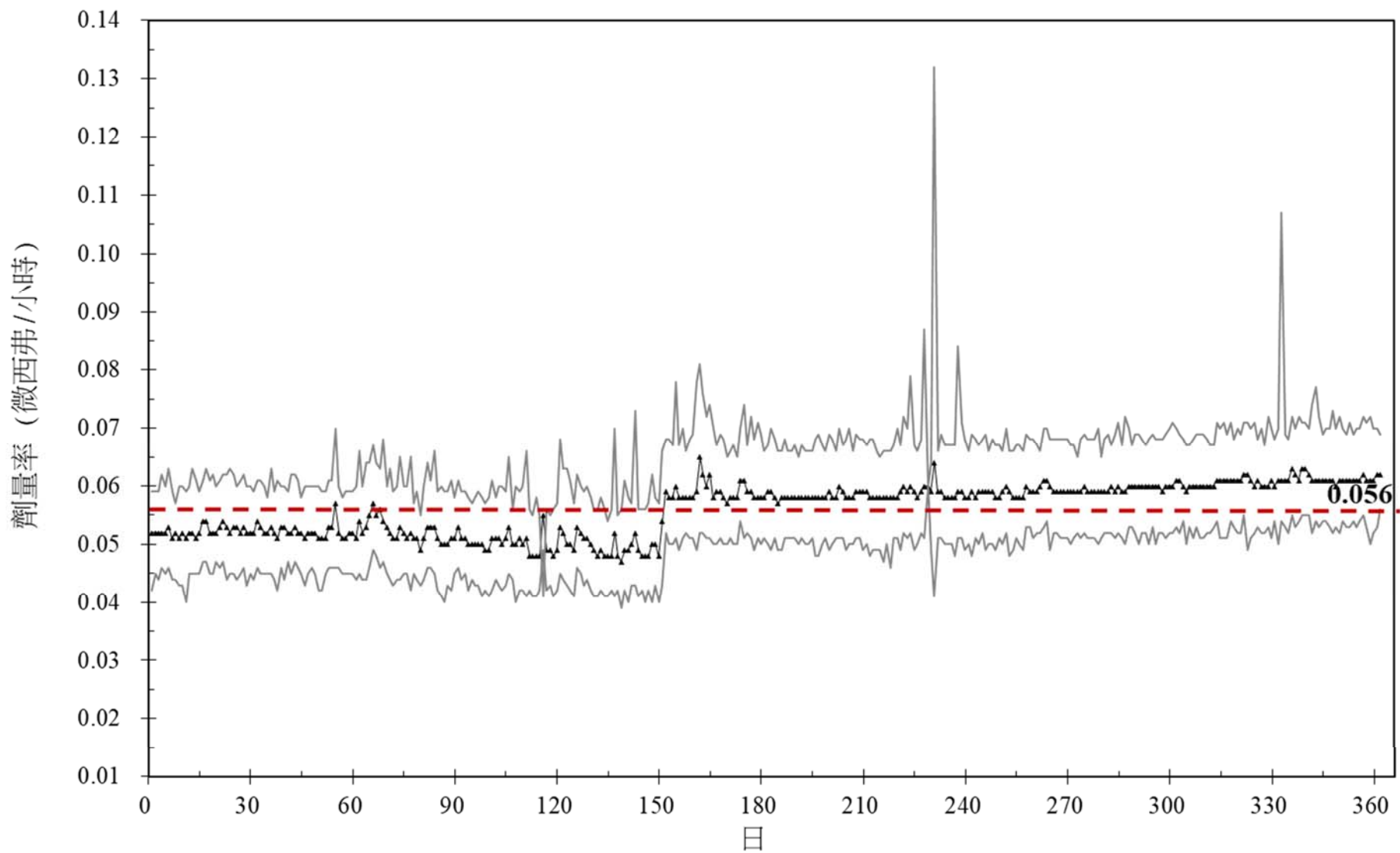
圖5 108年連續輻射偵測劑量率變動圖(加速器館)
