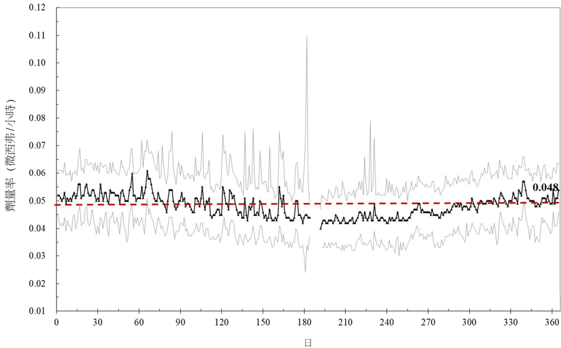
圖 4 108 年連續輻射偵測劑量率變動圖(李存敏館)
