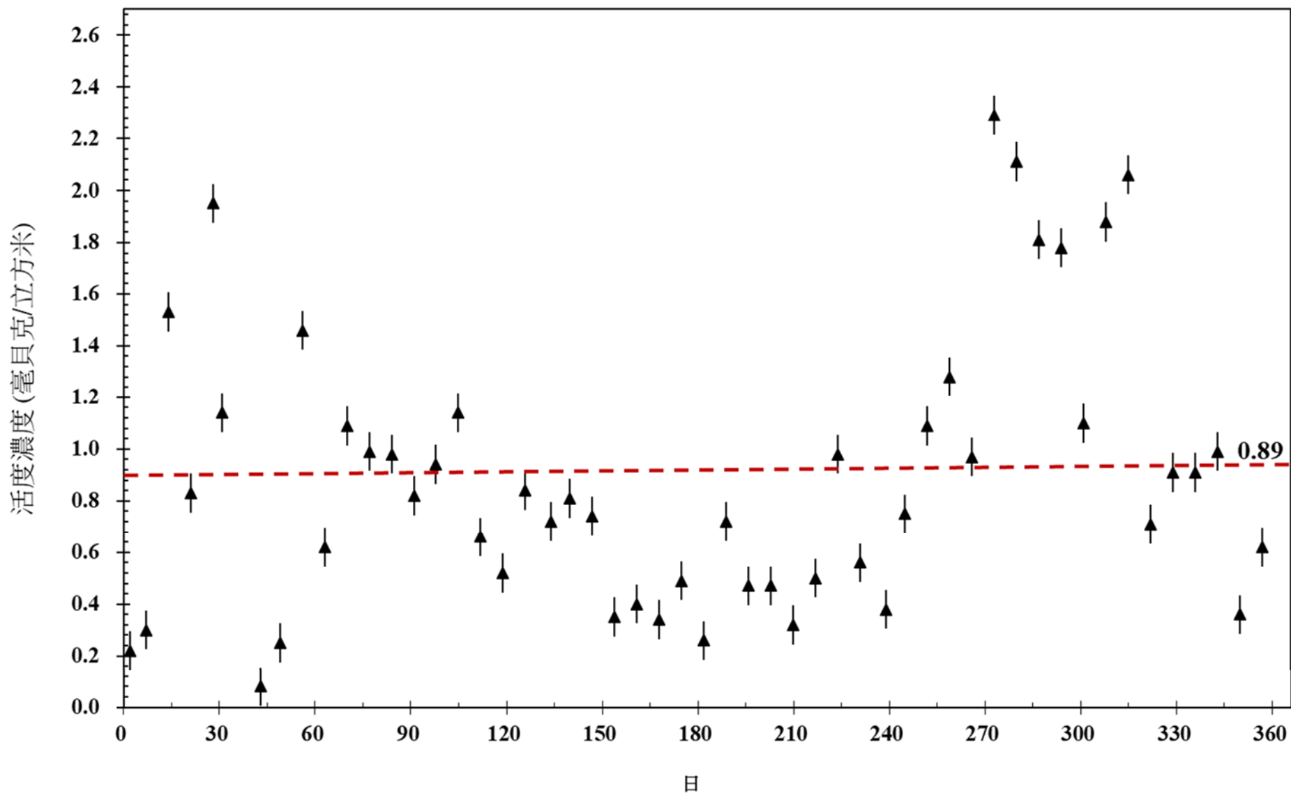
圖6 108年空浮微粒活度濃度變動圖(李存敏館)
