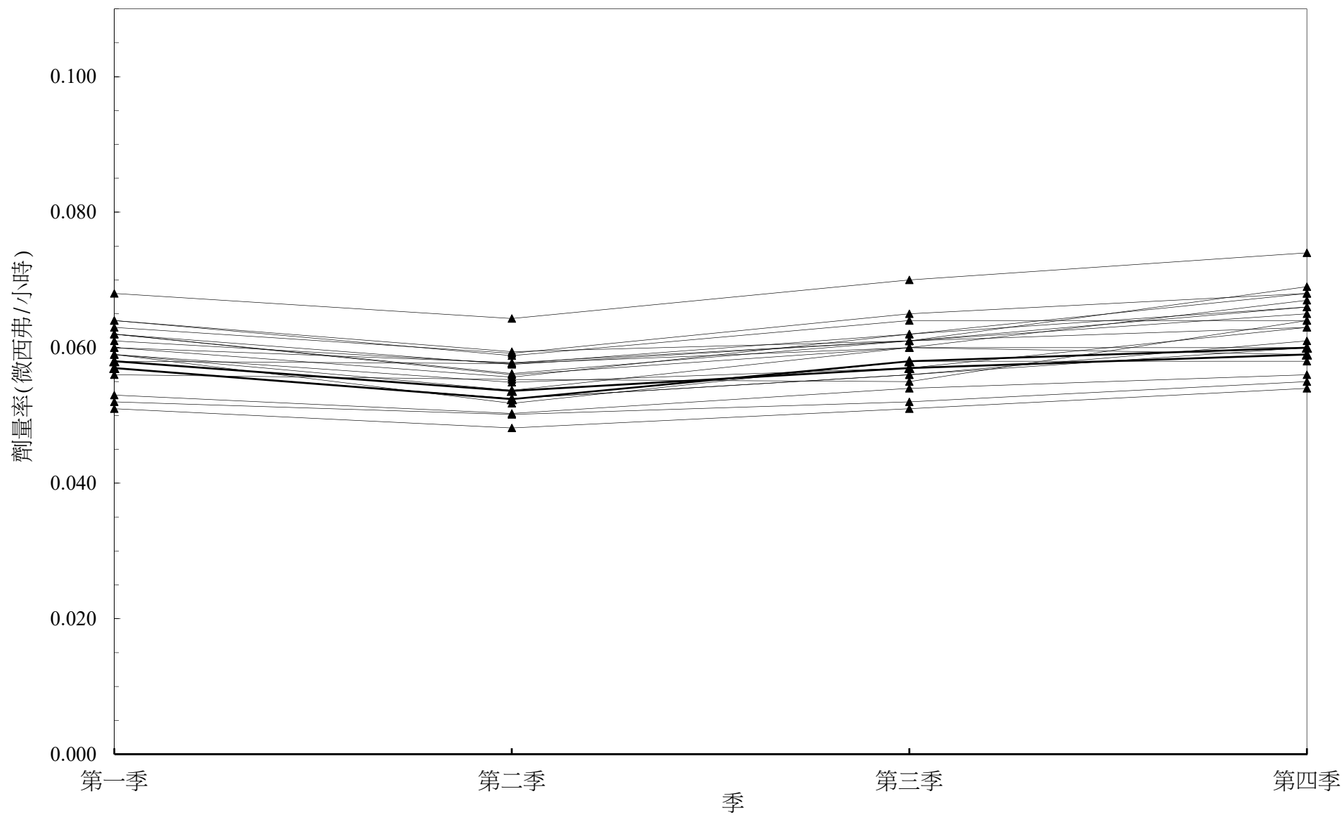
圖2 108年熱發光劑量計偵測站劑量率變動圖
