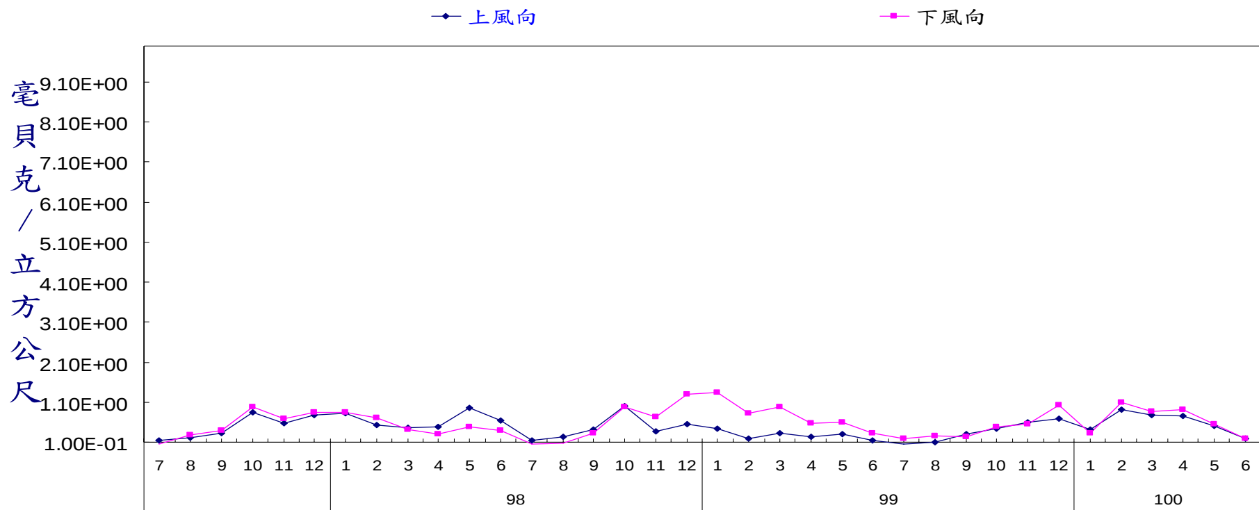
圖 14 核能二廠上下風向空氣微粒總貝他活度監測結果 年
