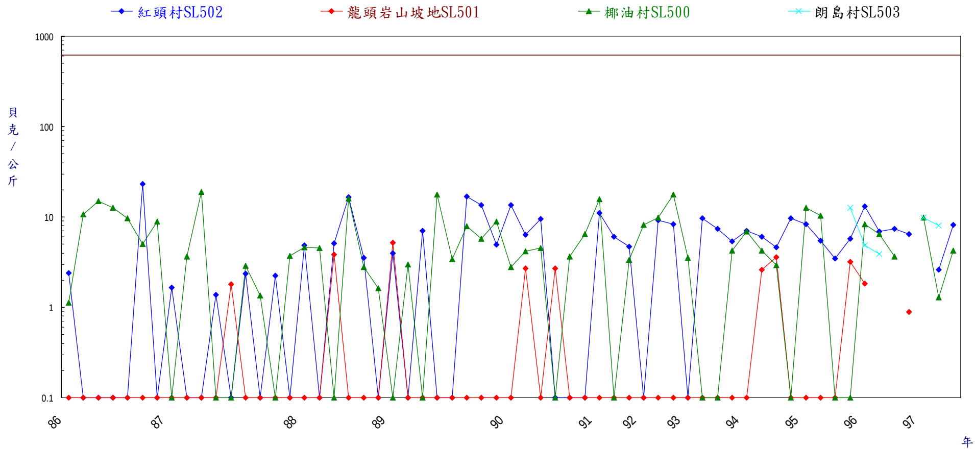
圖3 蘭嶼貯存場土壤銫-137加馬能譜分析結果
