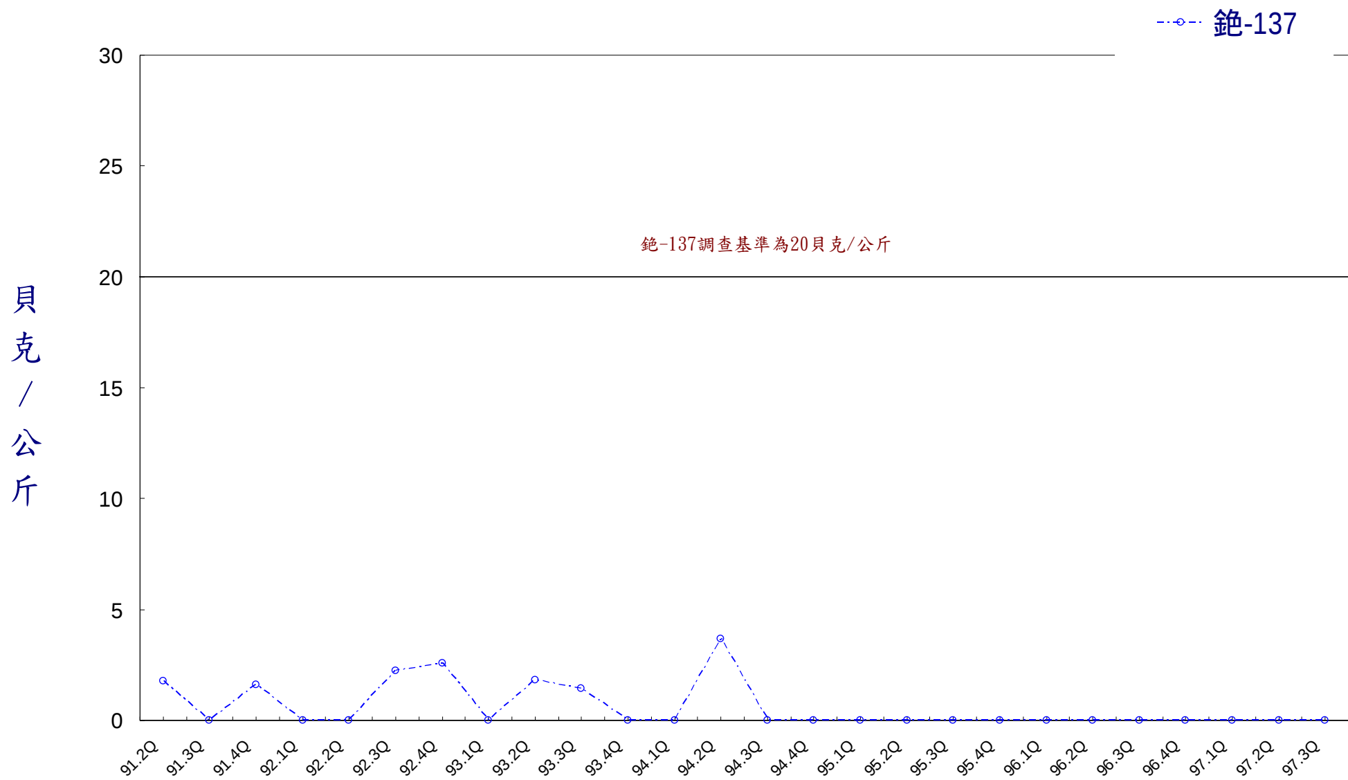
圖4 蘭嶼貯存場排水口岸沙加馬能譜分析結果
