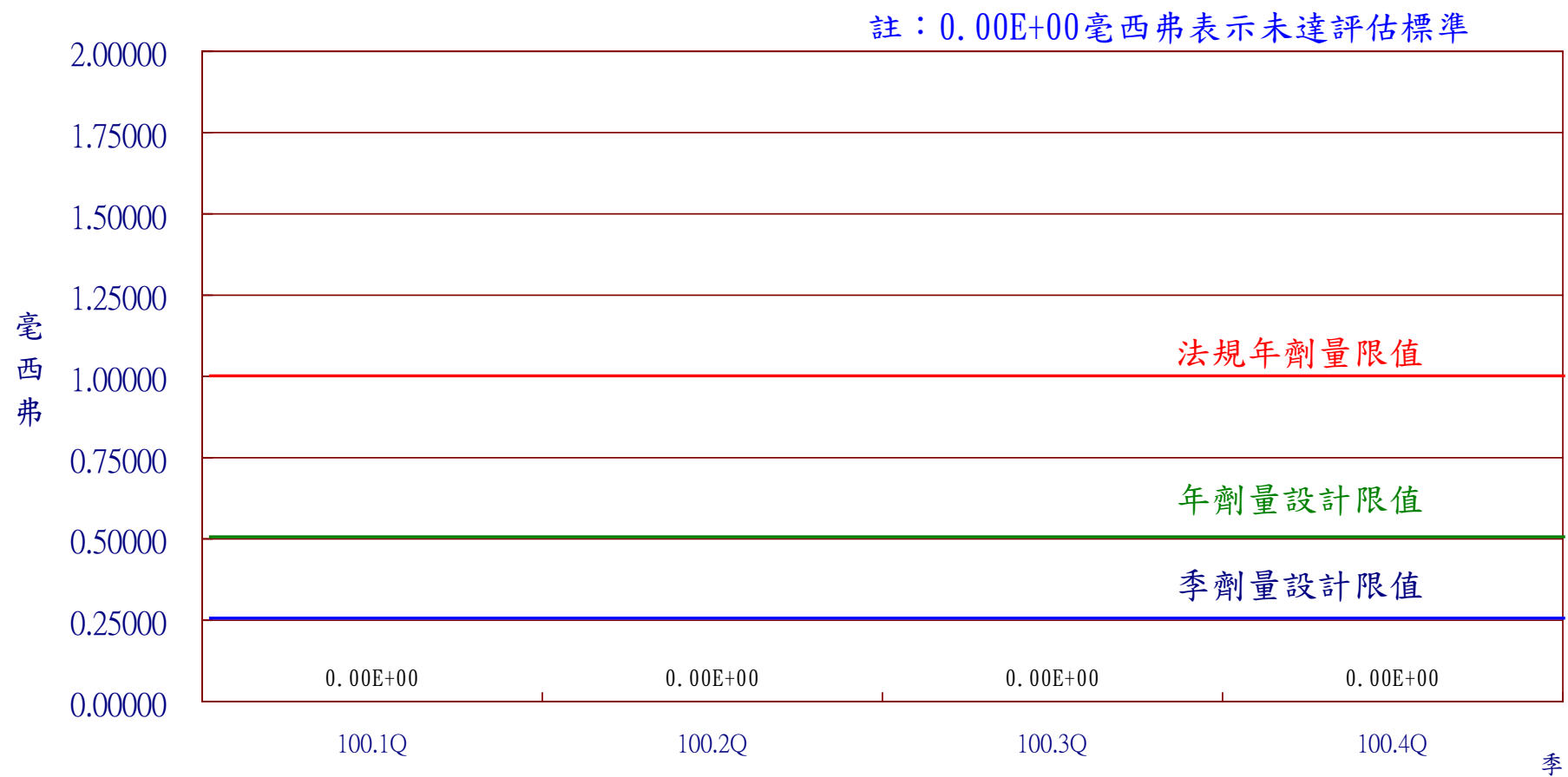
圖16 核能二廠100年第4季民眾最大個人全身劑量
