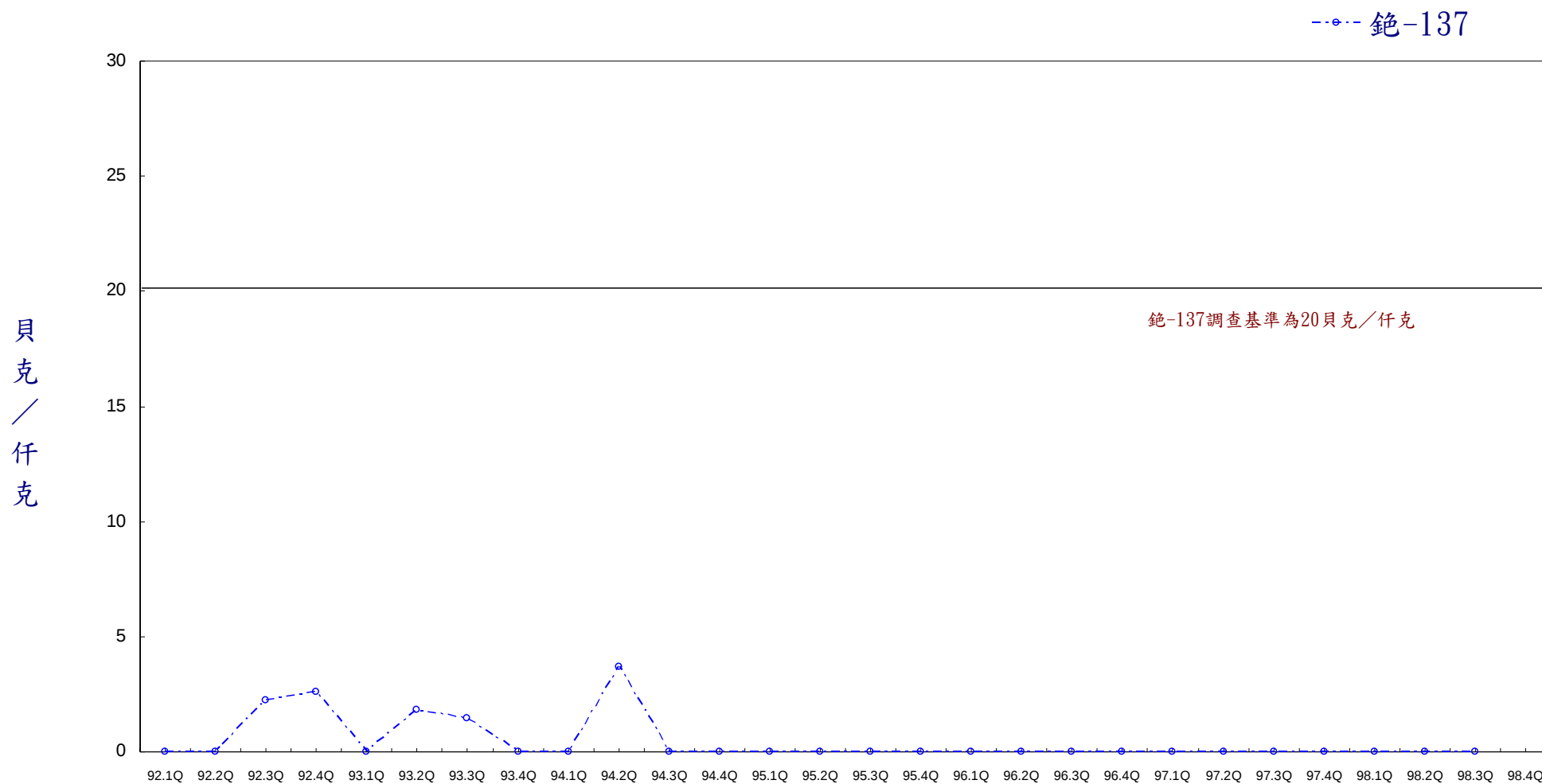
圖4 蘭嶼貯存場排水口岸砂加馬能譜分析結果
