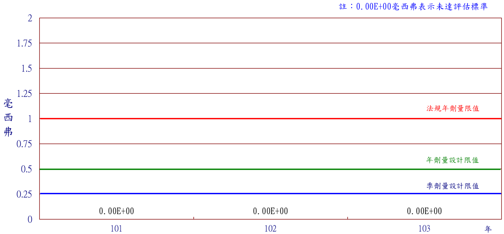
圖17 核能三廠103年民眾最大個人全身劑量
