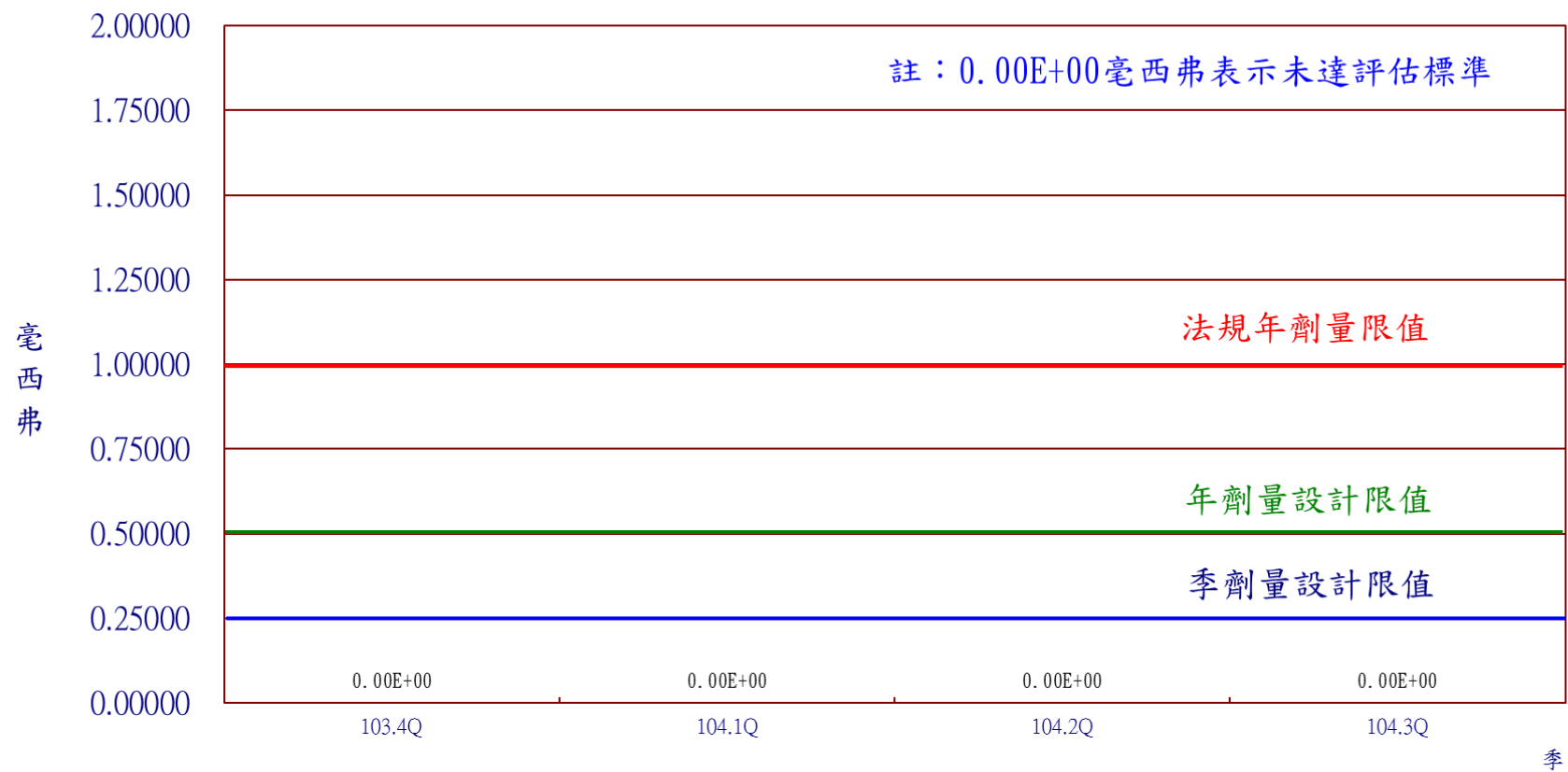
圖18 核能一廠104年第3季民眾最大個人全身劑量
