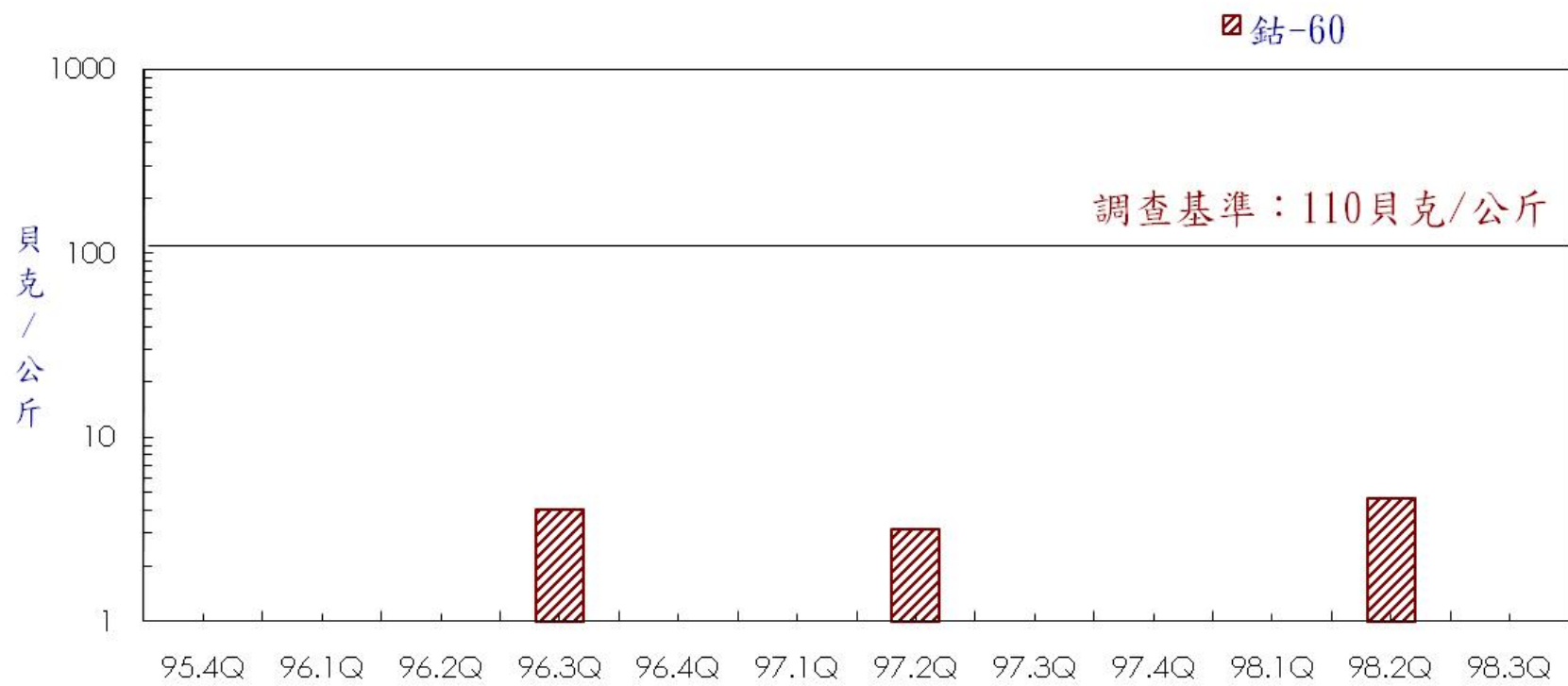
圖15 核能二廠出水口附近排水涵管下方岸沙加馬能譜監測結果
