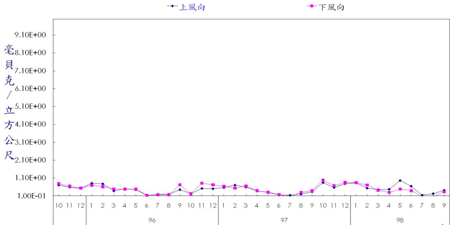
圖 14 核能二廠上下風向空氣微粒總貝他活度監測結果 年
