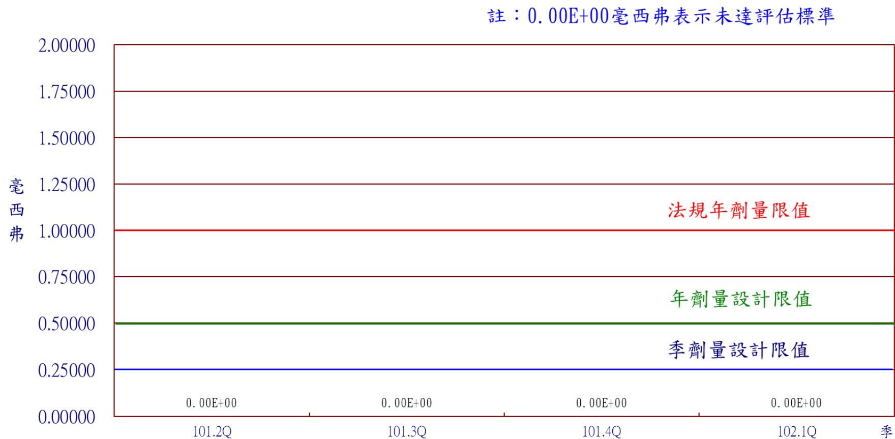
圖16 核能二廠102年第1季民眾最大個人全身劑量
