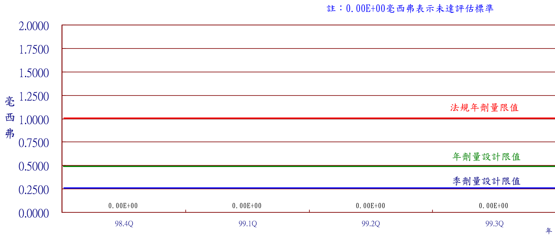
圖17 核能三廠99年第3季民眾最大個人全身劑量
