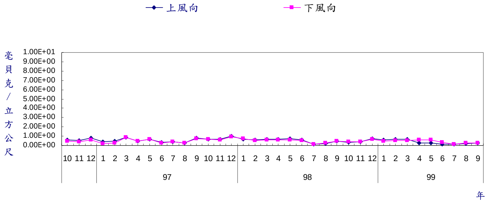
圖 15 核能三廠上下風向空氣微粒總貝他活度監測結果
