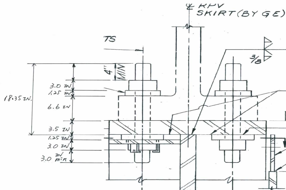
圖3 錨定螺栓結構尺寸(右側代表內圈)
