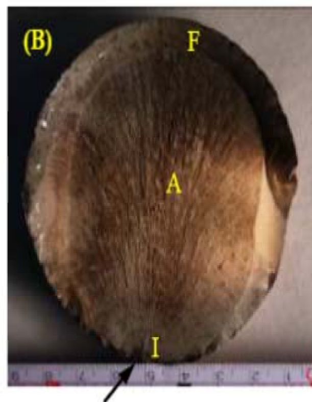
(圖4為A2螺栓斷面照片，(A)為原始形貌，(B)為清理後形貌；I為破斷起裂源，A為龜裂成長區，F為最終拉斷區)
