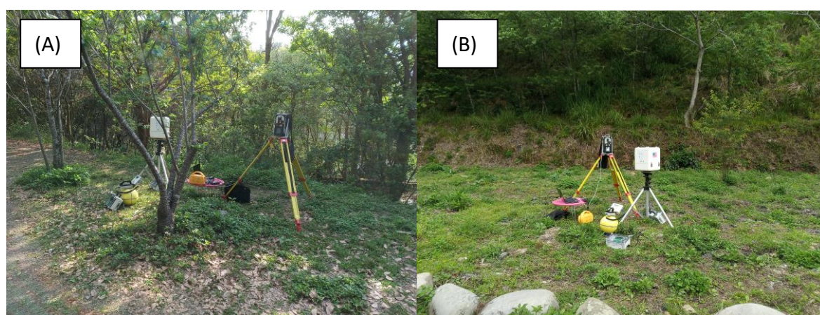
圖 4.2.5 省道 20、27 號沿途量測儀器架設與量測情形(A)台 27 縣近 18.5km 路標(B) 櫻花公園。
