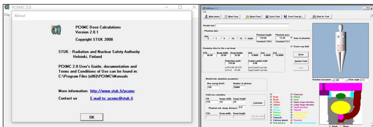
圖 4.2.17 劑量評估軟體-PCXMC 軟體版本及操作介面
