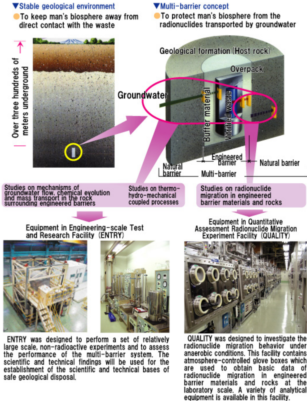
圖 43- 高放射性廢棄物深地層處置示意圖
