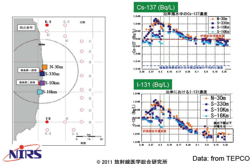
圖25- 日本福島沿岸海水中銫和碘隨時間變化的活度濃度分佈情形
