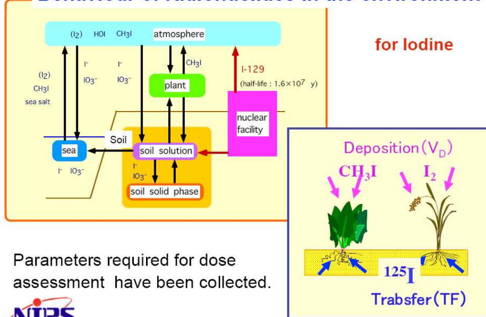
圖19- 放射性碘進入環境之過程
