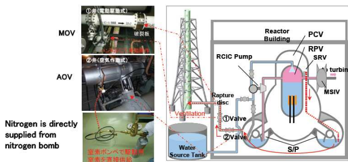
圖13- 圍阻體排氣
