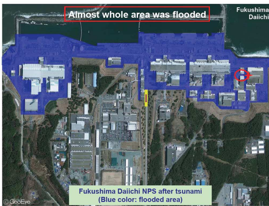
圖06-海嘯襲擊日本福島第一核電廠造成淹水情形（圖上藍色區域所示）
