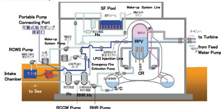
圖12- 利用可攜式泵進行爐心注水(反應爐喪失冷卻能力狀況)
