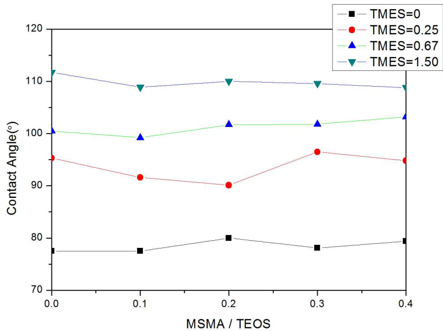
圖 14：TMESm3 與接觸角之關係
