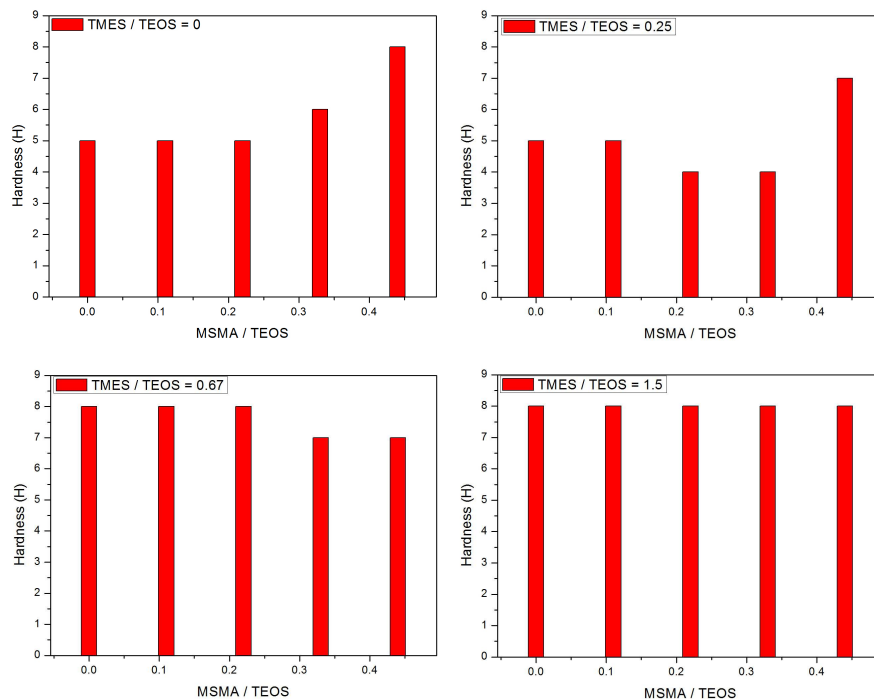
圖 15：矽烷比例對薄膜硬度之影響
