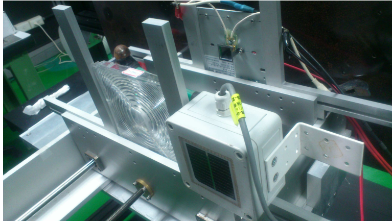
圖 3：HCPV 發電單一模組效率測量
