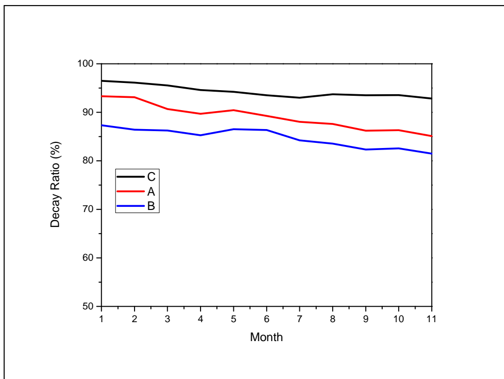
圖 5： HCPV 模組發電效能分析
