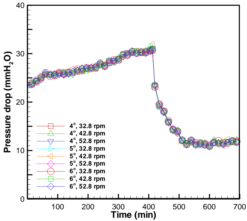
圖 18 細砂粒徑 1~2 mm 下各滾筒傾斜角與滾筒轉速之壓降
