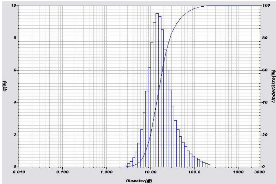
圖 28 細砂 1~2 mm，滾筒傾斜角 4°下之粒徑分析( D_{50}=12.71 \mu\text{m} )
