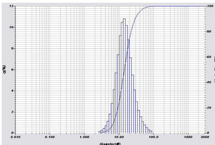
圖 23 細砂 0.2~0.5 mm，滾筒傾斜角 5°下之粒徑分析( D_{50}=12.52 \mu\text{m} )
