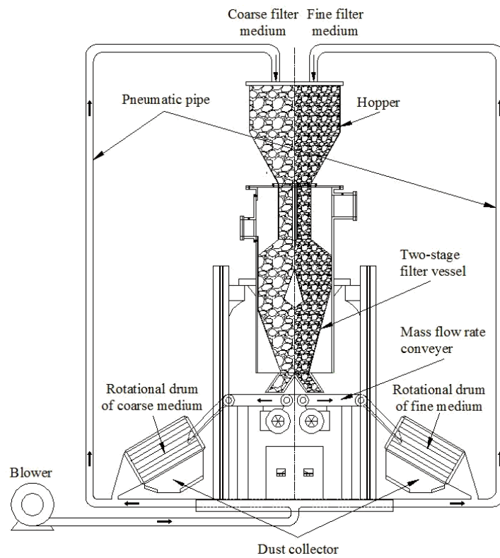
圖 4(b) 雙濾材再生循環系統與過濾器本體
