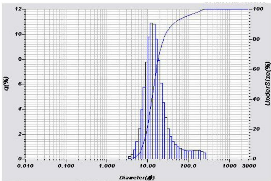
圖 29 細砂 1~2 mm，滾筒傾斜角 5°下之粒徑分析( D_{50}=12.75 \mu\text{m} )
