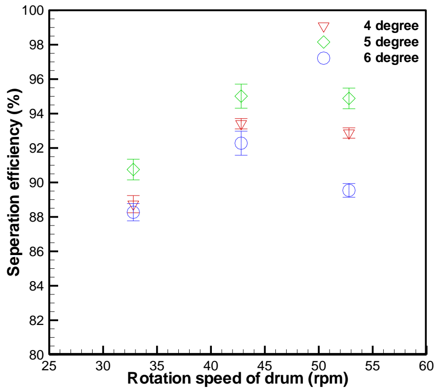
圖 15 細砂 1~2 mm 之分離效率
