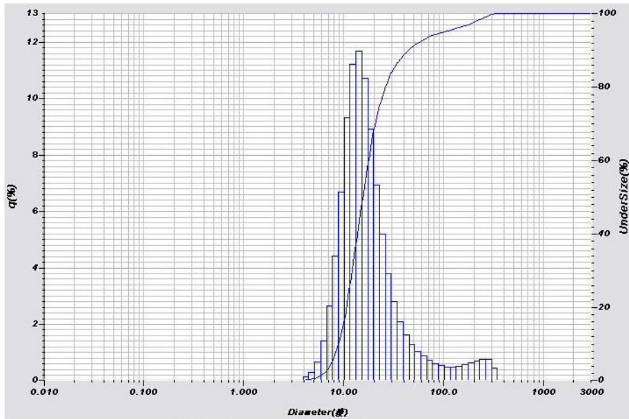
圖 26 細砂 0.5~1 mm，滾筒傾斜角 5°下之粒徑分析(D 50 =12.57 μm)
