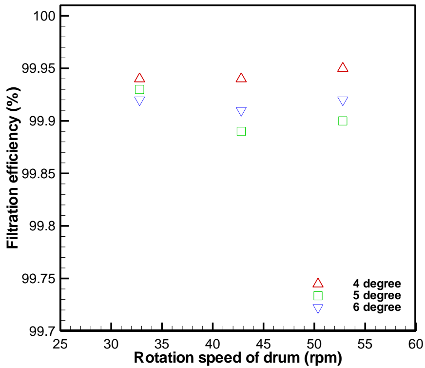
圖 20 細砂濾材 0.5~1 mm 之過濾效率
