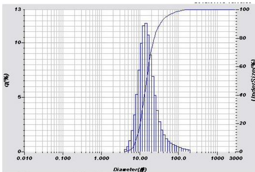
圖 22 細砂 0.2~0.5 mm，滾筒傾斜角 4°下之粒徑分析( D_{50}=12.55 \mu\text{m} )
