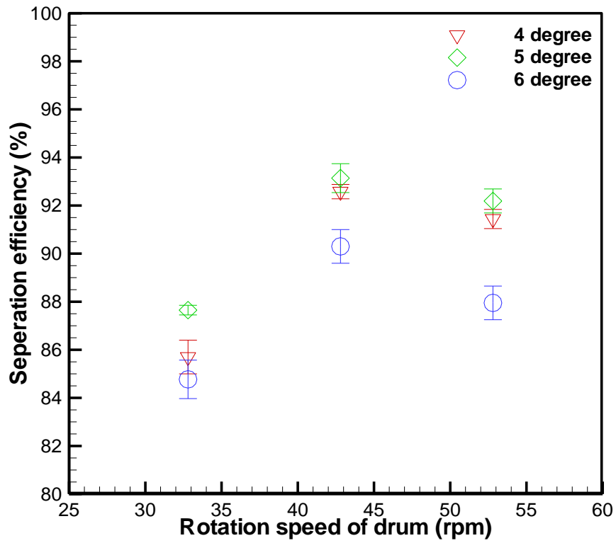
圖 13 細砂 0.2~0.5 mm 之分離效率
