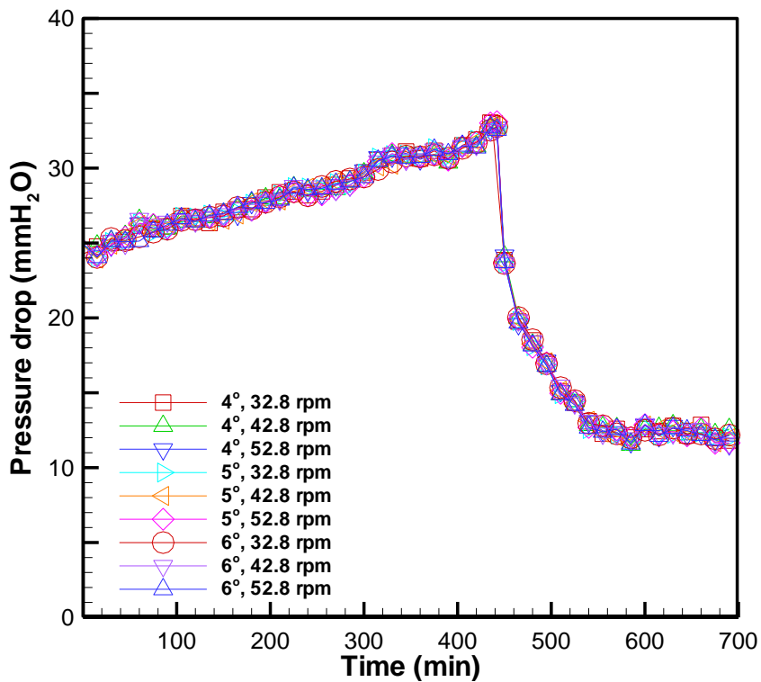
圖 17 細砂粒徑 0.5~1 mm 下各滾筒傾斜角與滾筒轉速之壓降
