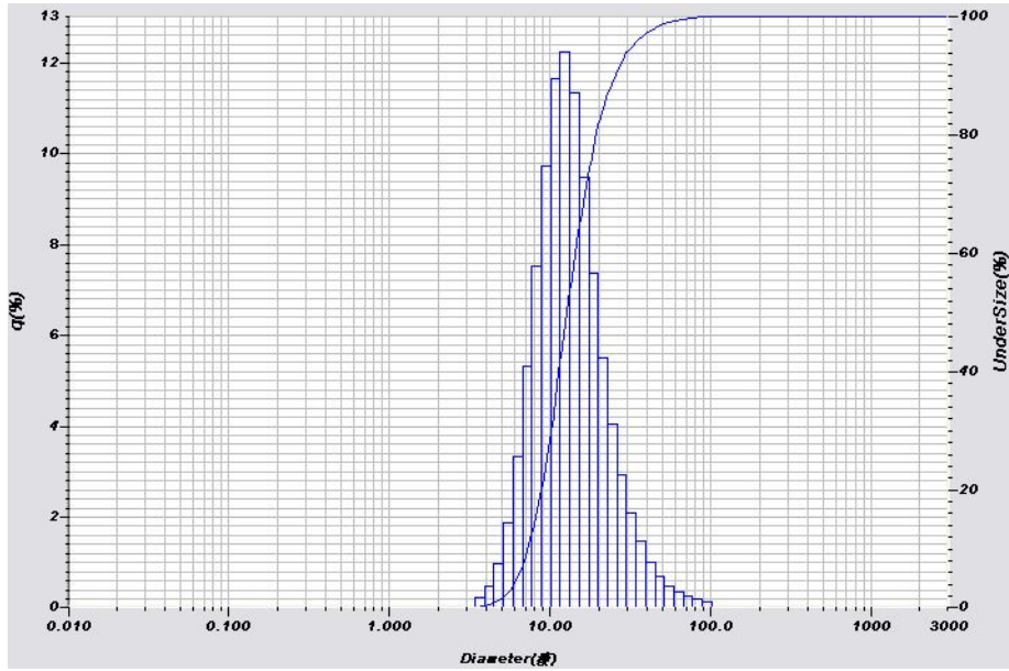
圖 24 細砂 0.2~0.5 mm，滾筒傾斜角 6°下之粒徑分析(D 50 =12.55 μm)
