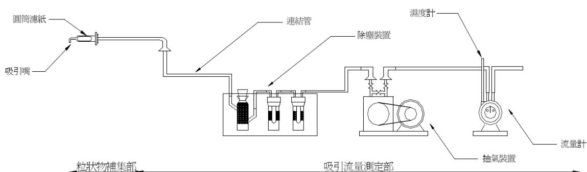
圖 9 採樣裝置
