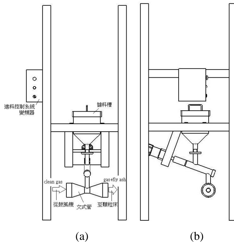
圖 6 粉塵供應器(a)前視圖(b)側視圖
