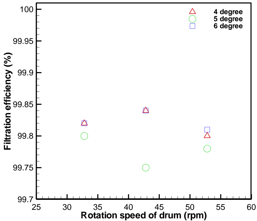
圖 21 細砂濾材 1~2 mm 之過濾效率
