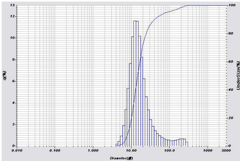
圖 27 細砂 0.5~1 mm，滾筒傾斜角 6°下之粒徑分析(D 50 =12.63 μm)
