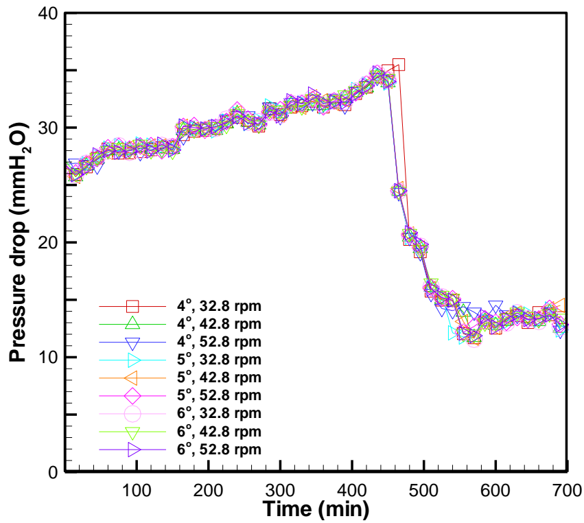
圖 16 細砂粒徑 0.2~0.5 mm 下各滾筒傾斜角與滾筒轉速之壓降
