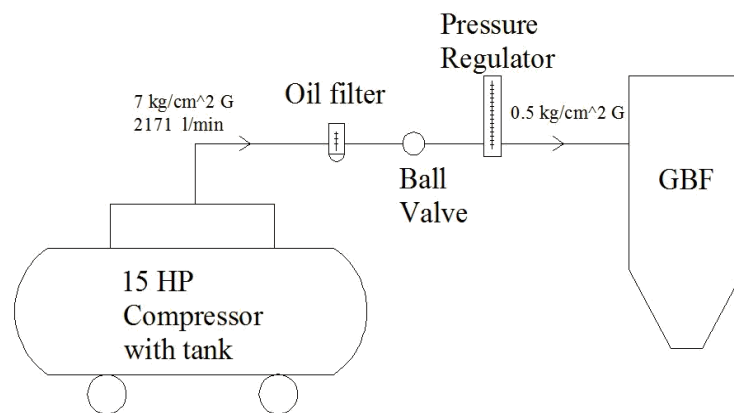
圖 5 氣體供應裝置示意圖
