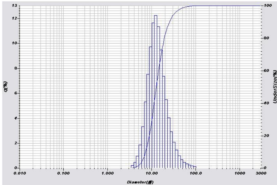
圖 25 細砂 0.5~1 mm，滾筒傾斜角 4°下之粒徑分析(D 50 =12.59 μm)
