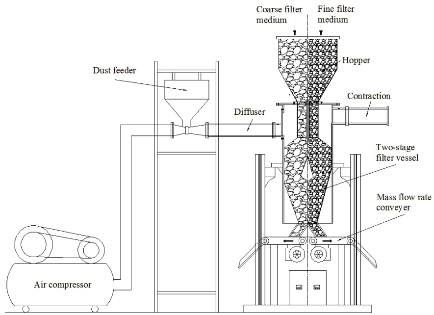
圖 4(a) 三維冷性能過濾系統
