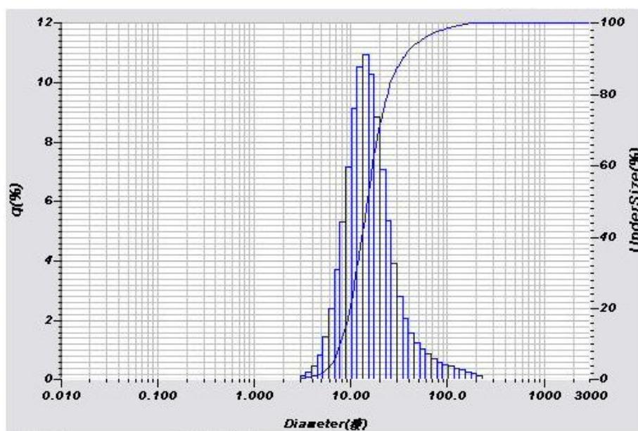
圖 30 細砂 1~2 mm，滾筒傾斜角 6°下之粒徑分析(D 50 =12.70 μm)
