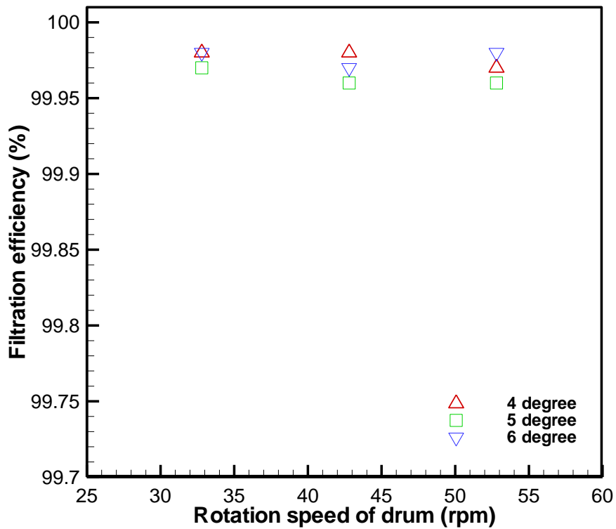
圖 19 細砂濾材 0.2~0.5 mm 之過濾效率
