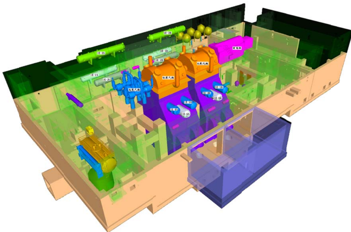
圖 6-35 汽機及飼水加熱器布置圖
