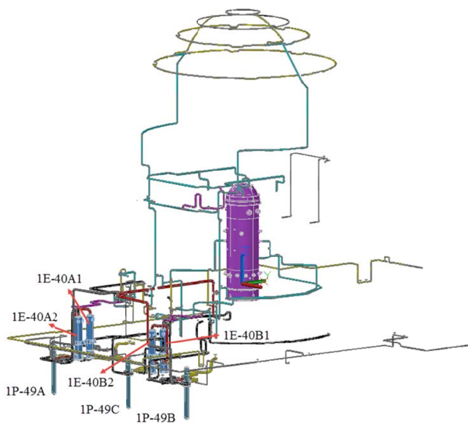
圖 6-26 餘熱移除管路系統
