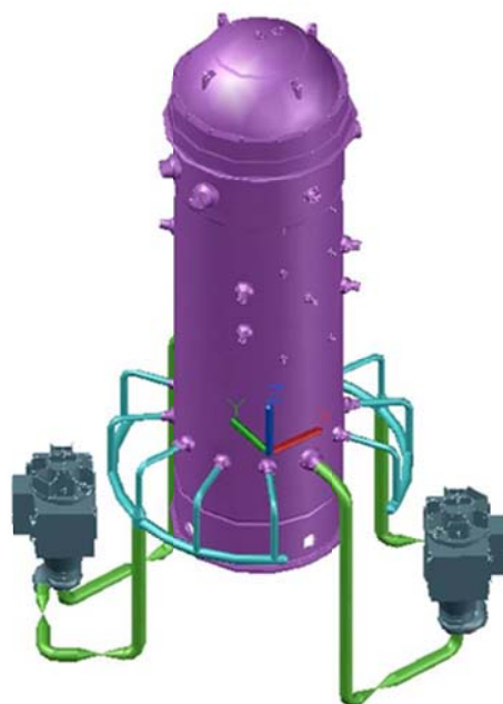
圖 6-27 再循環水系統
