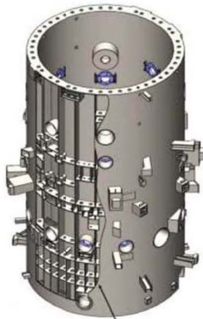
生物屏蔽鋼結構局部剖面圖
