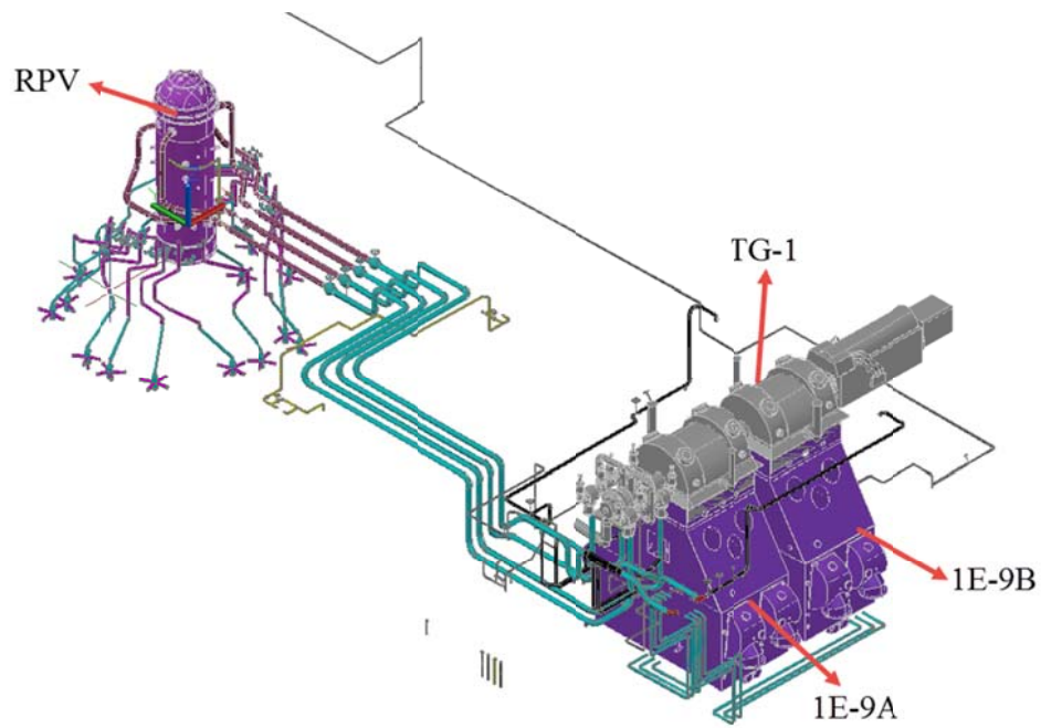
圖 6-28 主蒸汽系統
