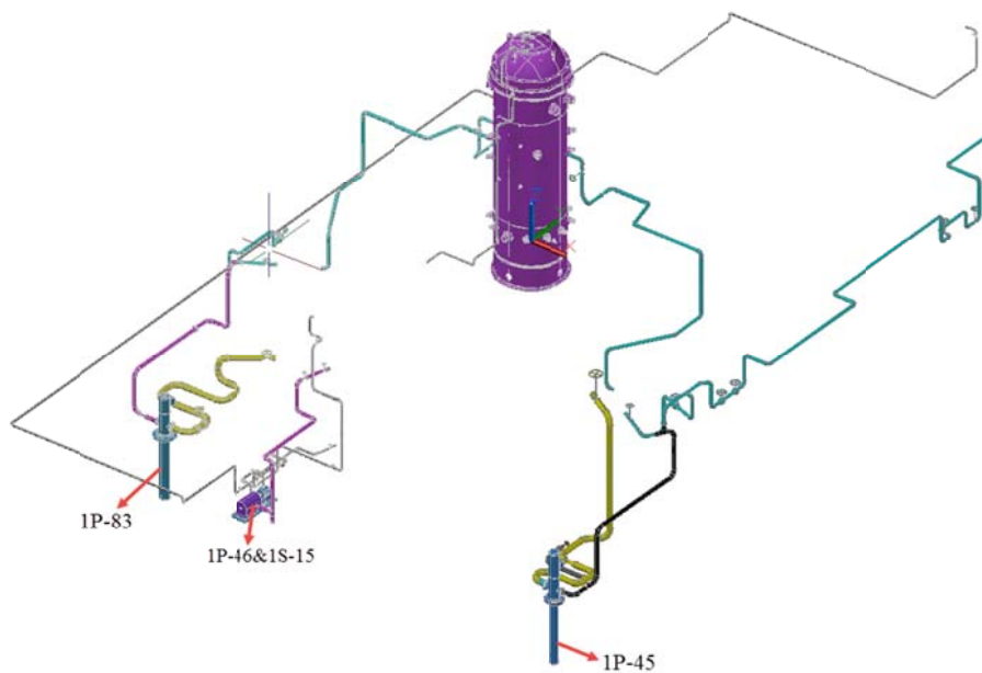
圖 6-30 緊急爐心冷卻系統
