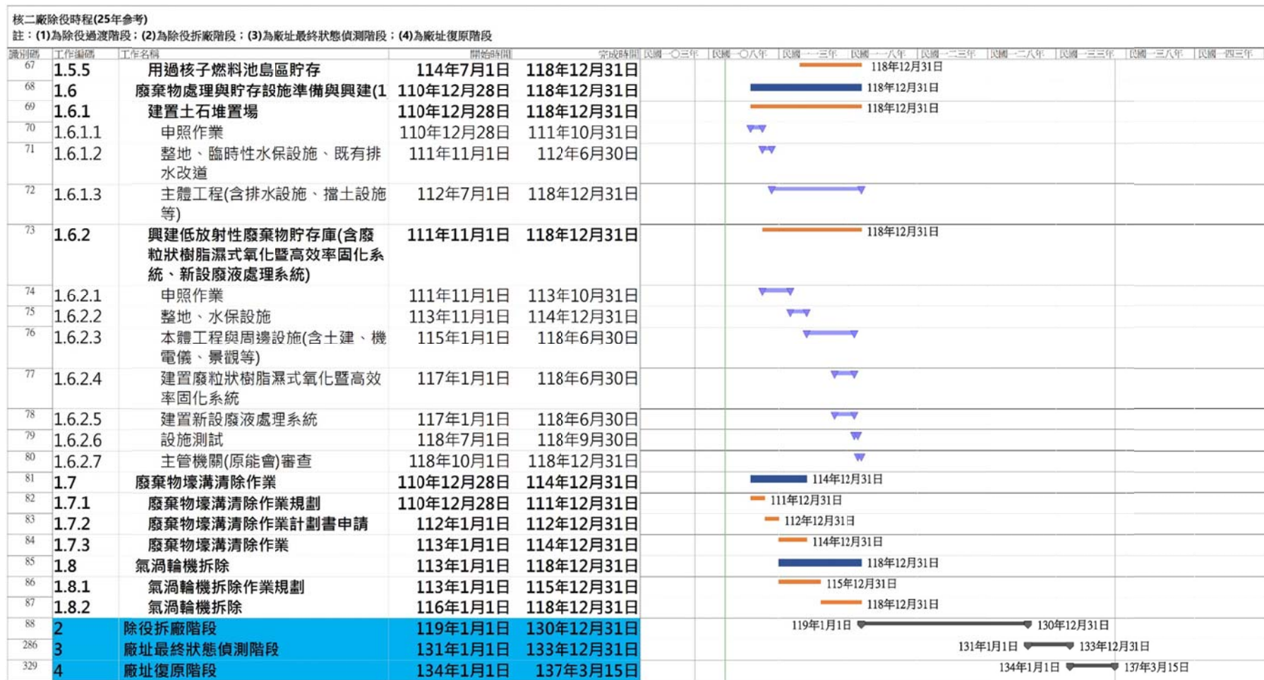
圖 6-1 除役過渡階段作業排程
