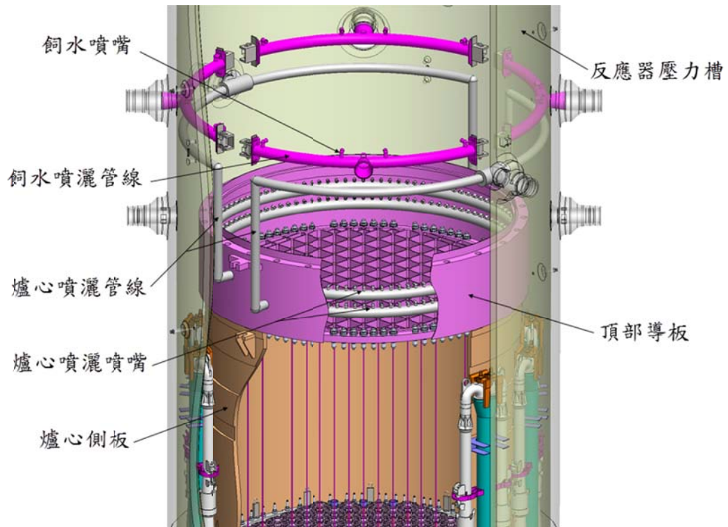
圖 6-15 飼水噴嘴及爐心噴灑噴嘴位置
