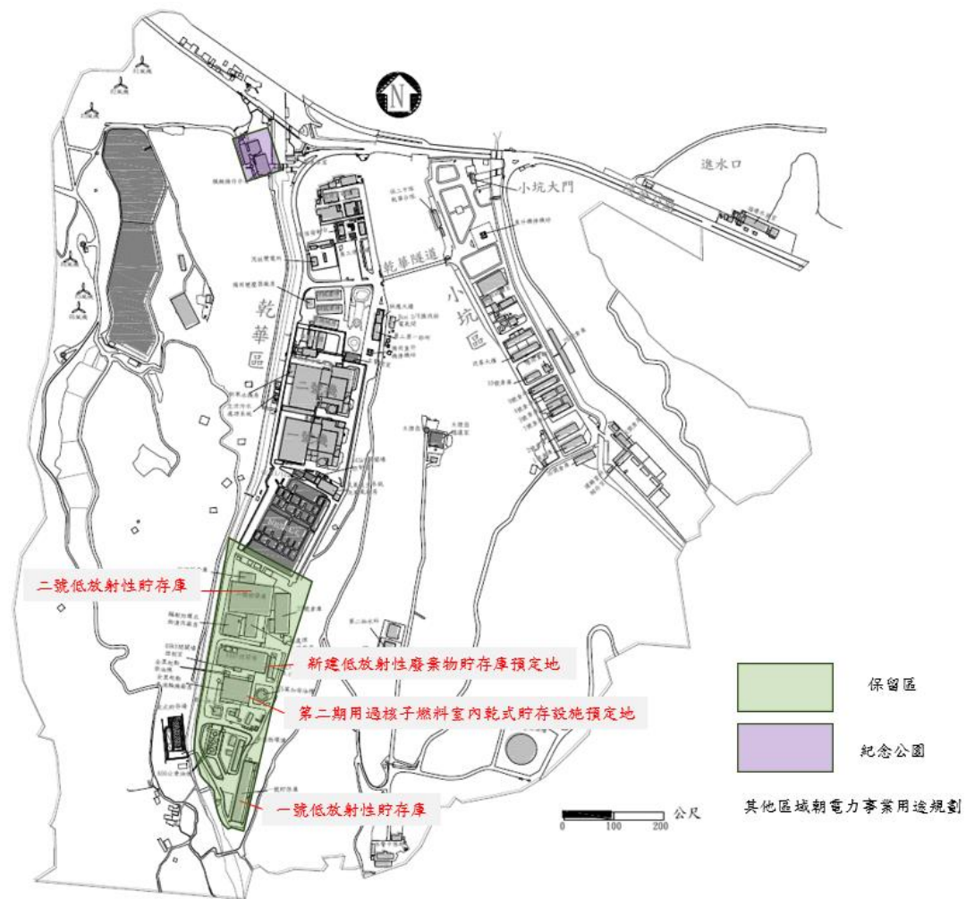
圖 10-3 核一廠保留區平面圖
