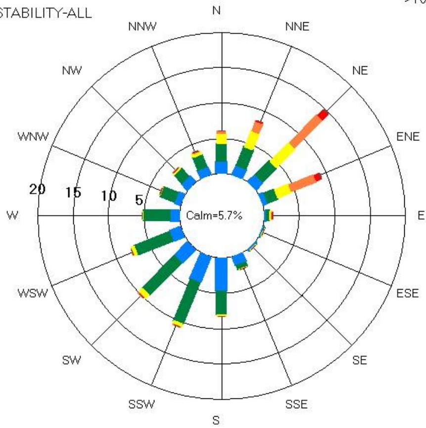
圖 10-1 核一廠 99 年至 103 年計 5 年平均之低塔氣象風花圖
