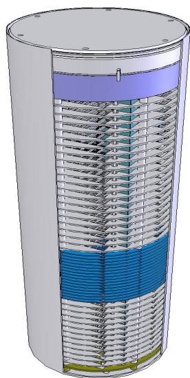
密封鋼筒(含燃料提籃)
