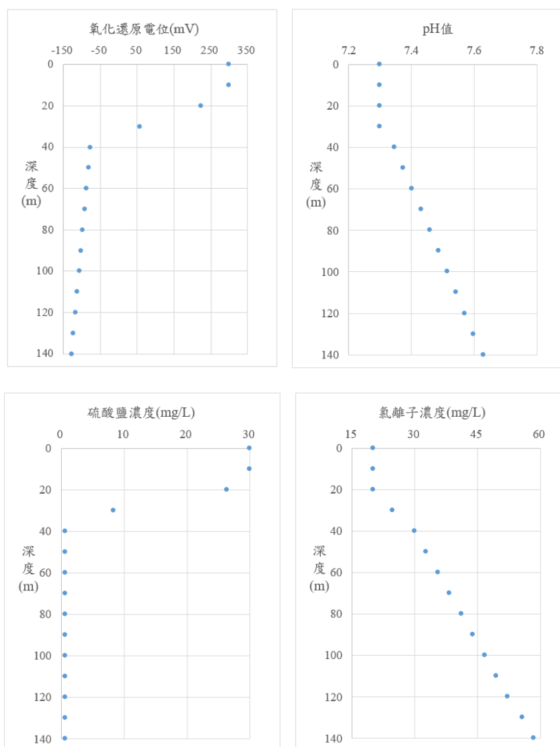
代表場址之 ORP、pH 值、硫酸鹽、氯離子隨深度變化趨勢
