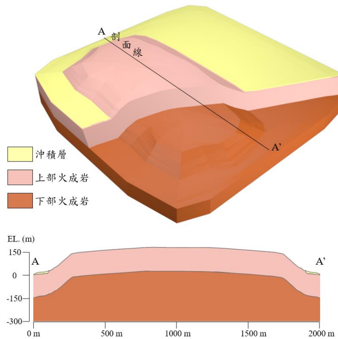
代表場址之地質環境概念模型
