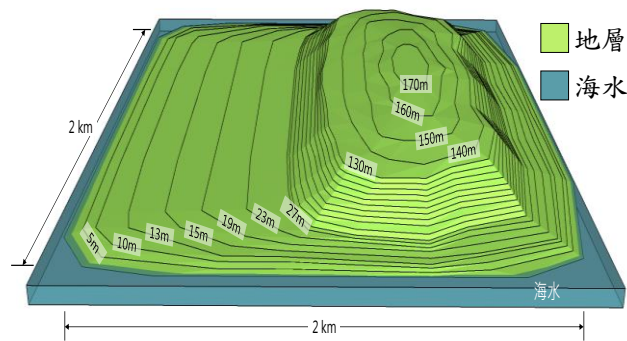
圖 2.2-3 代表場址環境概念示意圖
