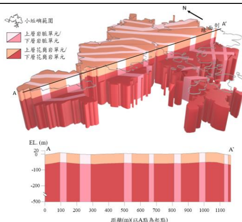
烏坵鄉建議候選場址之地質環境概念模型
