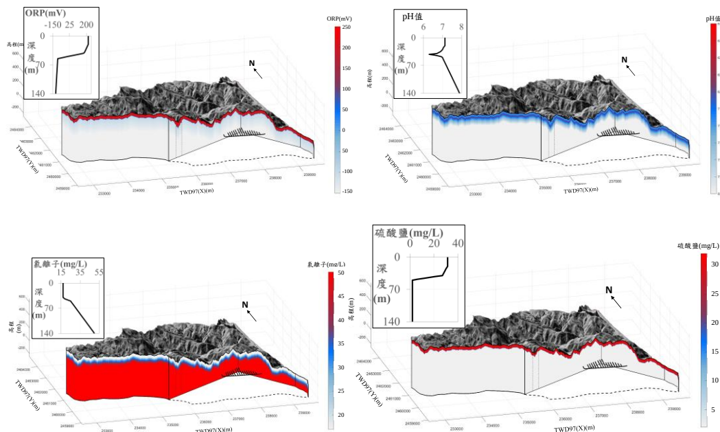
達仁鄉建議候選場址之 ORP、pH 值、氯離子與硫酸鹽隨深度變化
