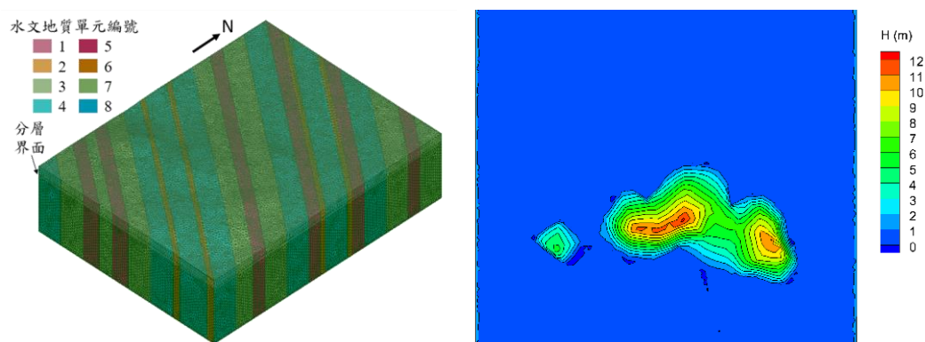
烏坵鄉建議候選場址之水文地質概念模型之數值模型(左)與水頭分布(右)
