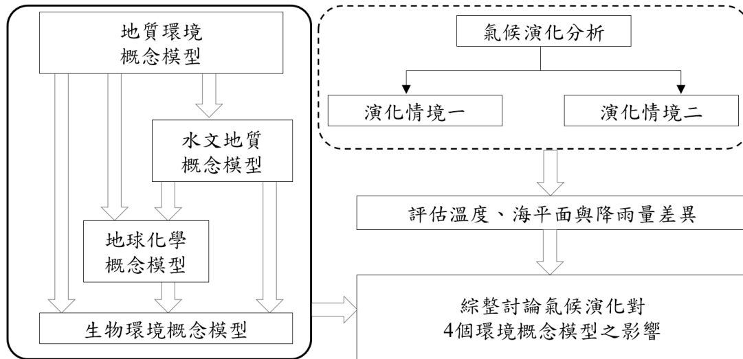
圖 2.2-2 4 個環境特徵模型之繼受關係及氣候演化關聯性
