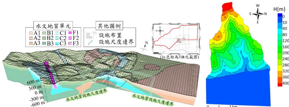
達仁鄉建議候選場址之水文地質概念模型之數值模型(左)與水頭分布(右)
