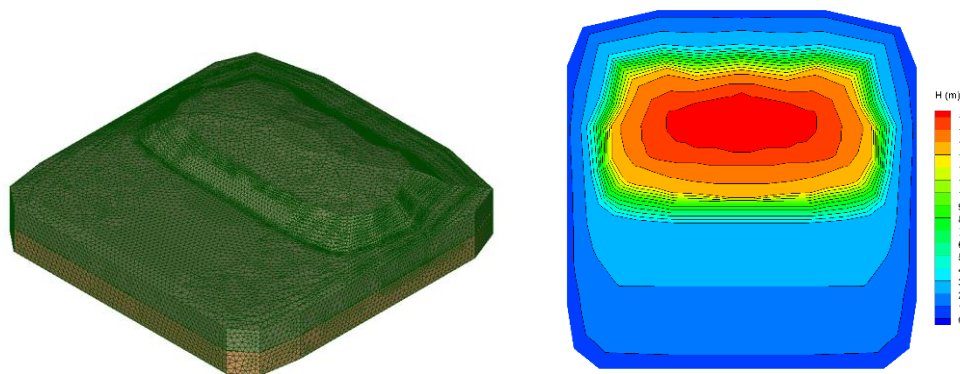
代表場址之水文地質概念模型之數值模型(左)與水頭分布(右)
