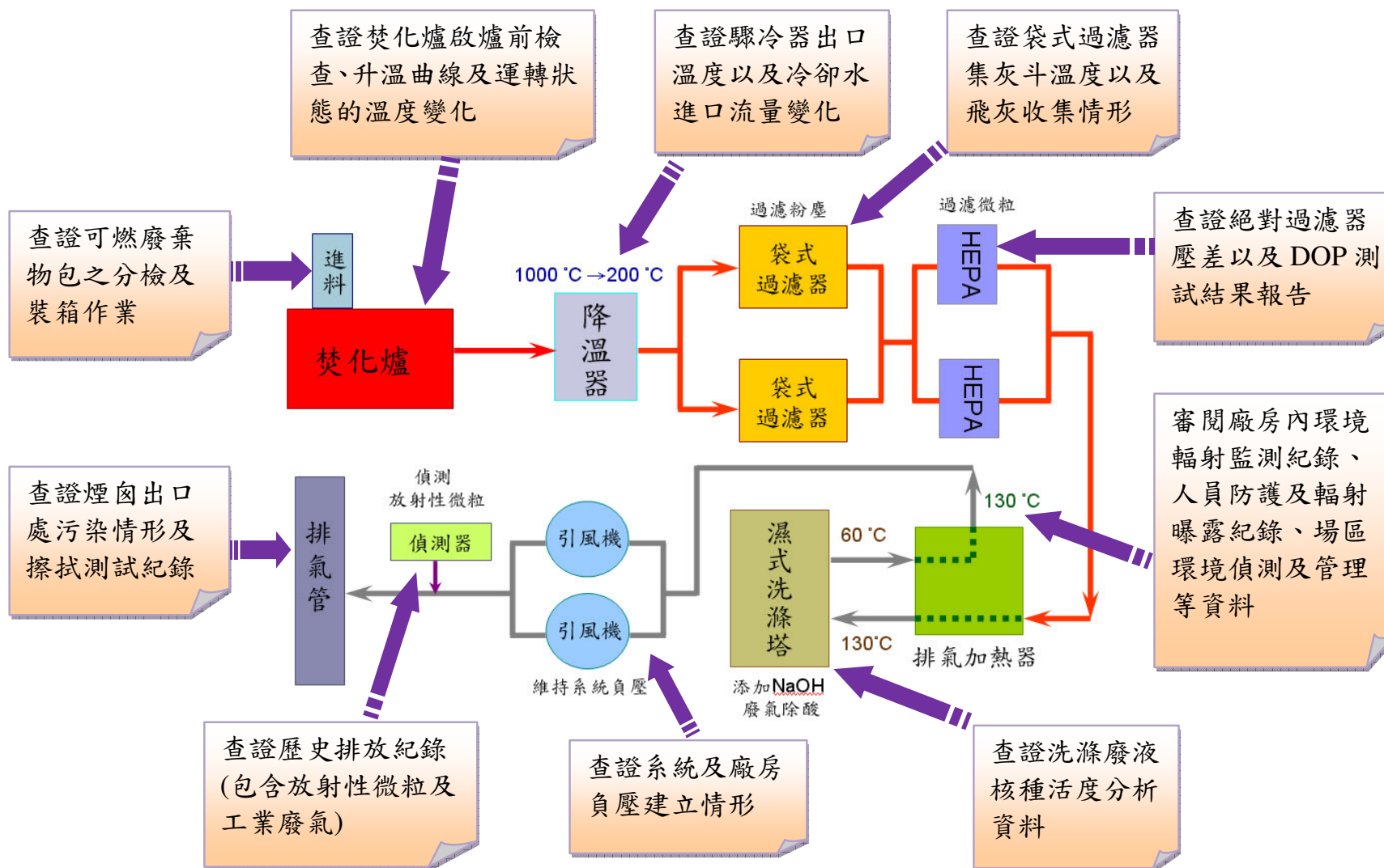
低放射性廢棄物焚化爐之安全管制重點示意圖
