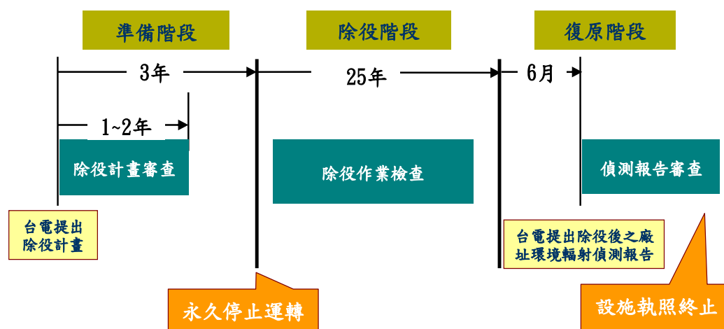
圖 6-1 核能電廠設施除役管制之作業流程
