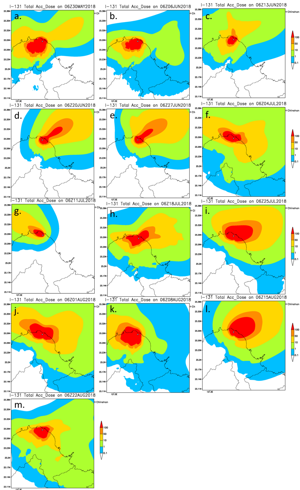
圖 4-20 核一廠夏季，自 2018 年 5 月 29 日至 2018 年 8 月 28 日 I-131 假想事故模擬之 7 日有效劑量累積圖(mSv)。
