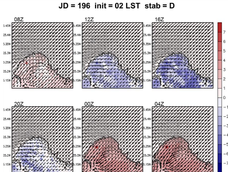
圖 5-83 A2Cflow 調校後之模擬(20m 高)風場，模擬日期太陽日為第 196 日，模擬初始時間為 20LST，中心位置為核一廠(第 3 層巢狀網格)，風向為 45^\circ ，風速為 8m/s，穩定度參數為 0.002(穩定度分類 D 級)，填色部分為溫度擾動，單位為 ^\circ\text{C} 。
