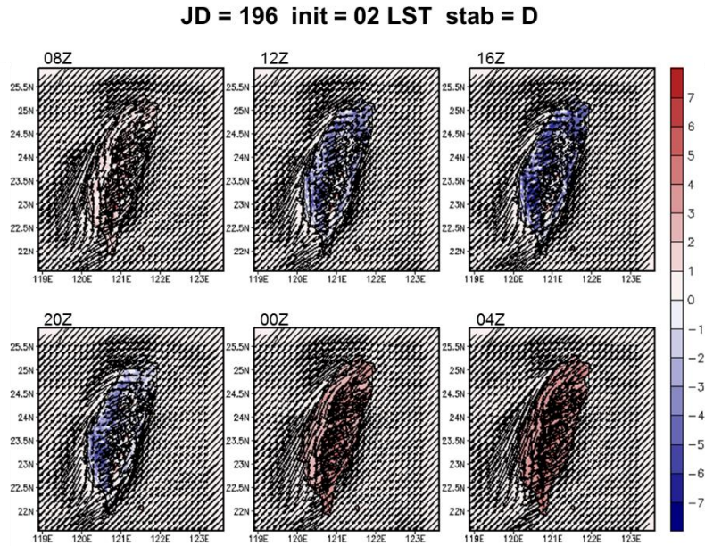
圖 5-81 A2Cflow 調校後之模擬(20m 高)風場，模擬日期太陽日為第 196 日，模擬初始時間為 20LST，中心位置為核一廠(第 1 層巢狀網格)，風向為 45^\circ ，風速為 8m/s，穩定度參數為 0.002(穩定度分類 D 級)，填色部分為溫度擾動，單位為 ^\circ\text{C} 。
