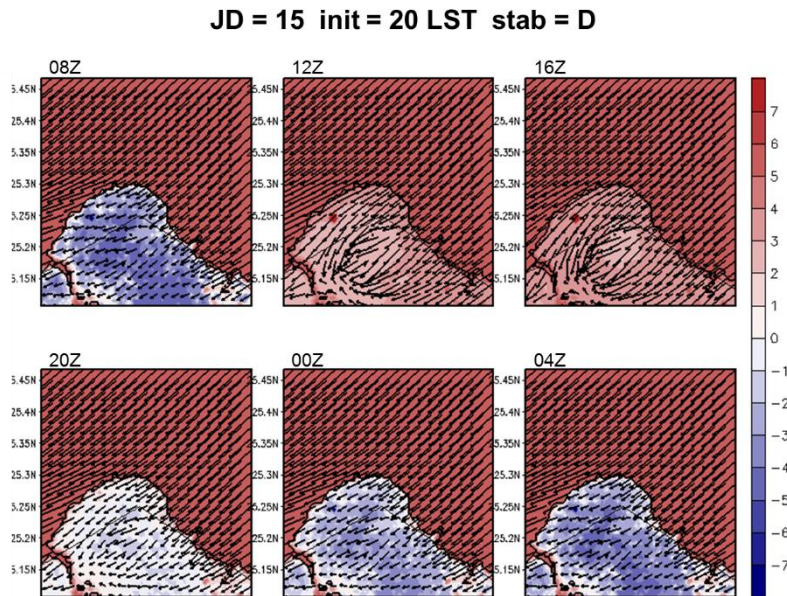
圖 5-35 A2Cflow 調校後之模擬(20m 高)風場，模擬日期太陽日為第 15 日，模擬初始時間為 20LST，中心位置為核一廠(第 3 層巢狀網格)，風向為 45^\circ ，風速為 5m/s，穩定度參數為 0.002(穩定度分類 D 級)，填色部分為溫度擾動，單位為 ^\circ\text{C} 。
