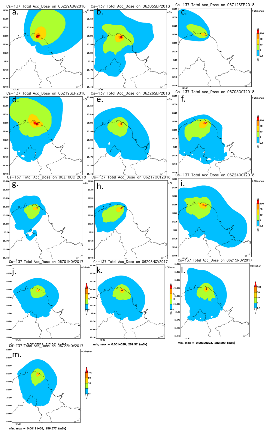
圖 4-25 核一廠秋季，自 2018 年 8 月 29 日至 2018 年 10 月 30 日和 2017 年 11 月 1 日至 11 月 29 日 Cs-137 假想事故模擬之 7 日有效劑量累積圖(mSv)。
