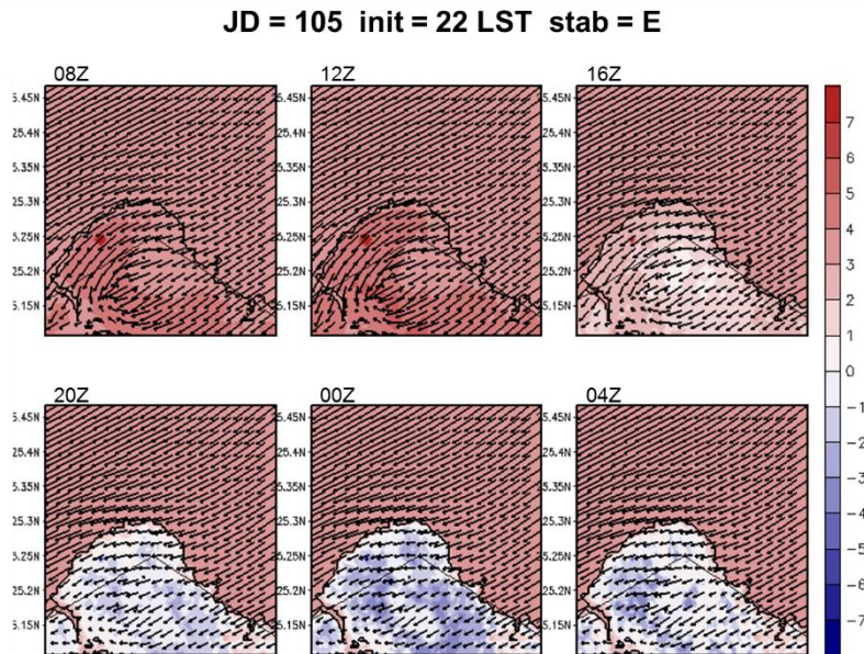
圖 5-79 A2Cflow 調校後之模擬(20m 高)風場，模擬日期太陽日為第 105 日，模擬初始時間為 20LST，中心位置為核一廠(第 3 層巢狀網格)，風向為 45^\circ ，風速為 8m/s，穩定度參數為 0.005(穩定度分類 ED 級)，填色部分為溫度擾動，單位為 ^\circ\text{C} 。
