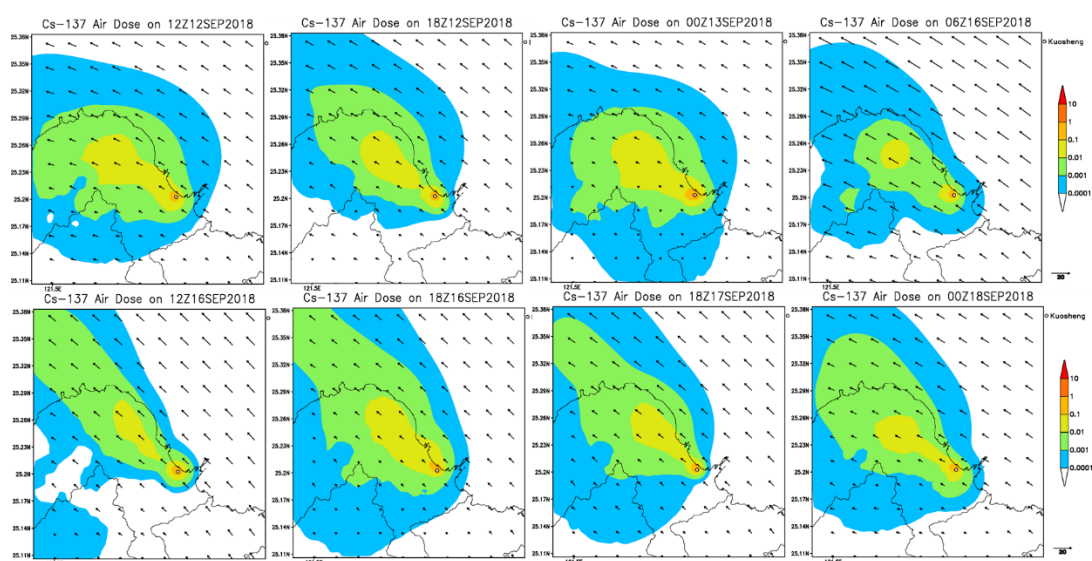
圖 4-29 2018 年 9 月 12 日當周，假想模擬中，Cs-137 劑量累積在金山地區的空 氣劑量率(mSv/hr)及風場。
