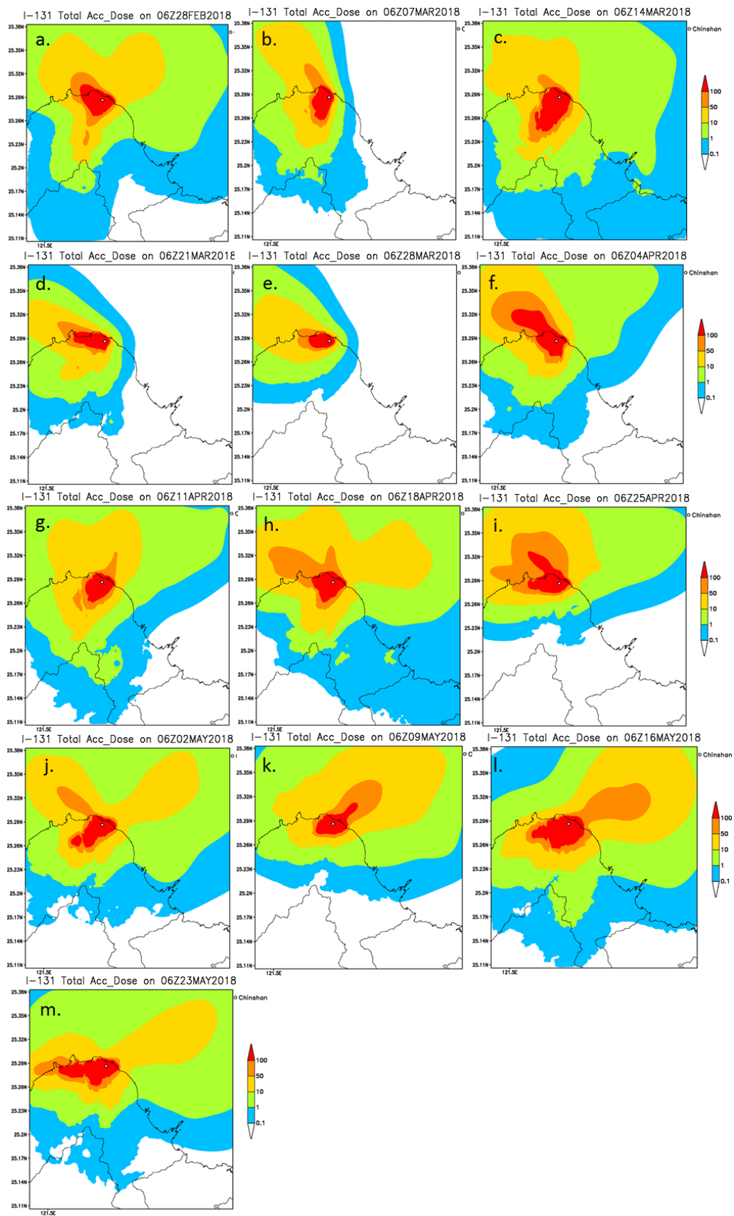
圖 4-13 核一廠春季，自 2018 年 2 月 28 日至 2018 年 5 月 23 日 I-131 假想事故模擬之 7 日有效劑量累積圖(mSv)。
