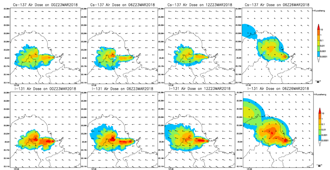
圖 4-16 2018 年 3 月 21 日當周，假想模擬中，劑量累積在大屯山的空氣劑量率及風場。上半部:Cs-137，下半部:I-131
