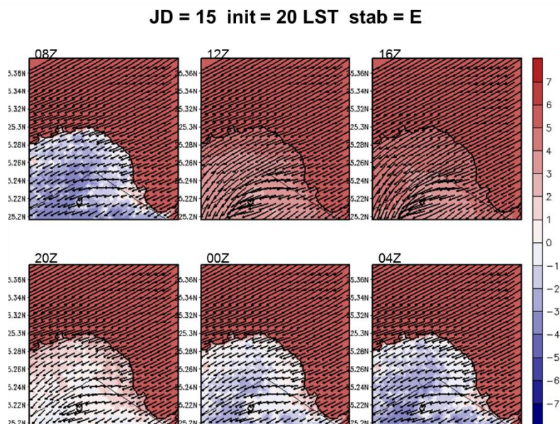
圖 5-40 A2Cflow 調校後之模擬(20m 高)風場，模擬日期太陽日為第 15 日，模擬初始時間為 20LST，中心位置為核一廠(第 4 層巢狀網格)，風向為 45^\circ ，風速為 5m/s，穩定度參數為 0.005(穩定度分類 E 級)，填色部分為溫度擾動，單位為 ^\circ\text{C} 。
