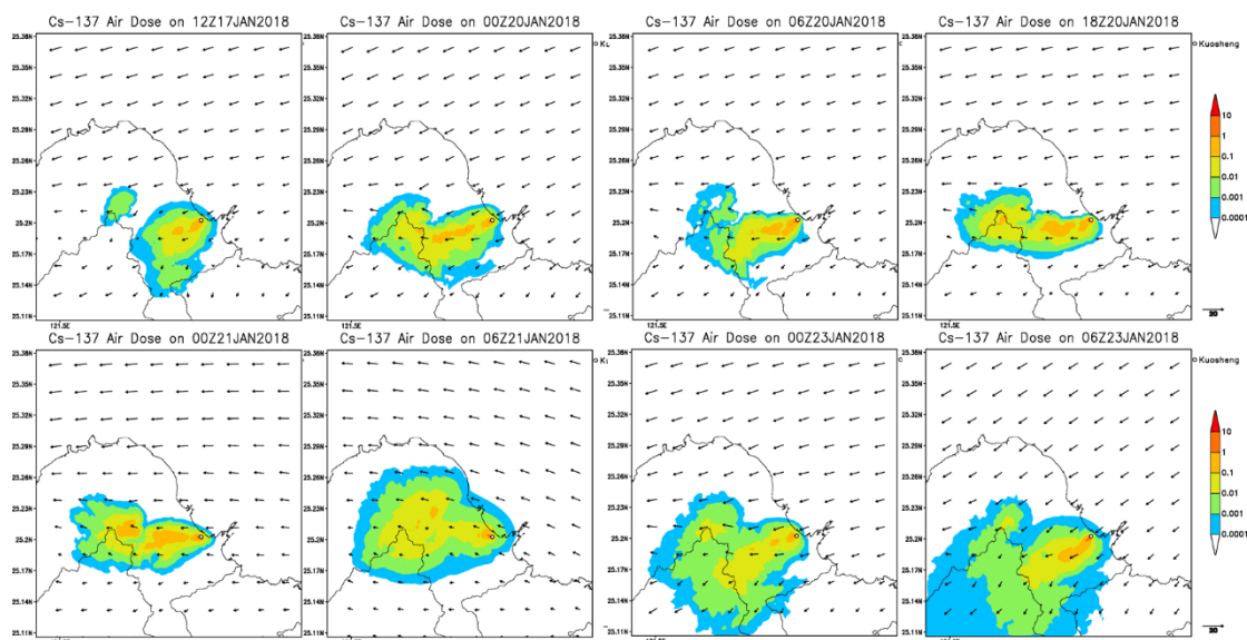
圖 4-6 2018 年 1 月 17 日當周，Cs-137 假想模擬中，劑量累積在大屯山的空氣劑量率及風場。
