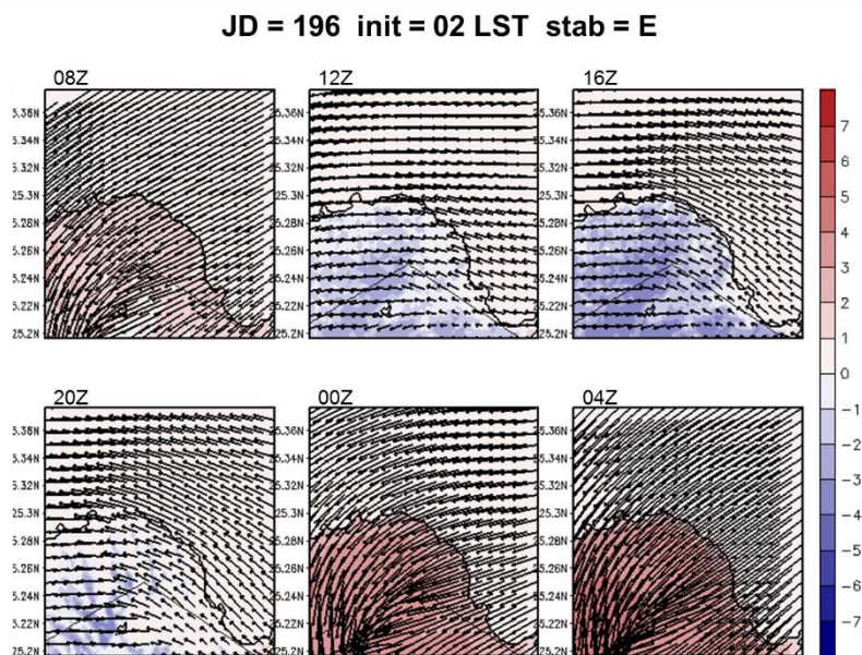
圖 5-24 A2Cflow 調校後之模擬(20m 高)風場，模擬日期太陽日為第 196 日，模擬初始時間為 02LST，中心位置為核一廠(第 4 層巢狀網格)，風向為 45^\circ ，風速為 2m/s，穩定度參數為 0.005(穩定度分類 E 級)，填色部分為溫度擾動，單位為 ^\circ\text{C} 。
