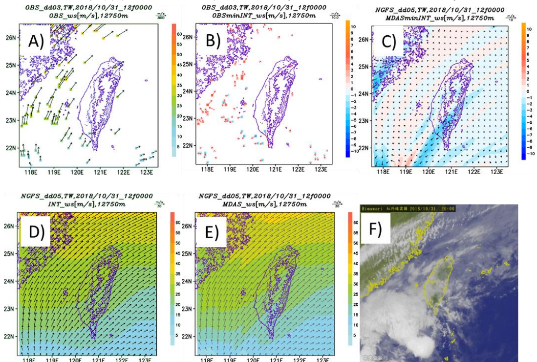
圖 6-7 2018 東北季風(10/31)12750 公尺風速。(A)傳統高空觀測資料、(B)觀測資料減初始猜測場、(C)MDAS 減初始猜測場、(D)初始猜測場、(E)MDAS 與(F)衛星雲圖；(A)(D)(E)風標為向量，(B)(C)風標為向量差。
