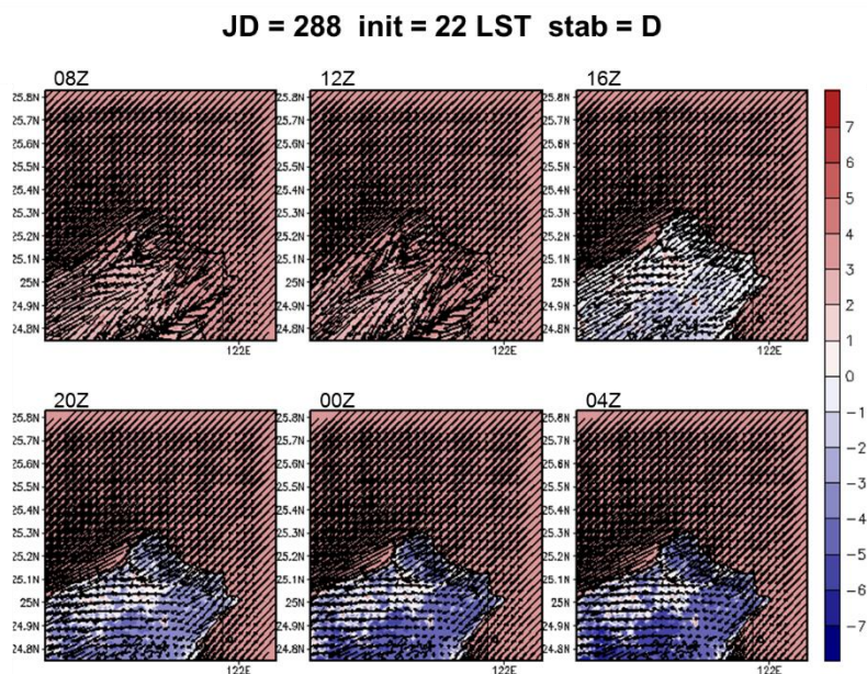
圖 5-58 A2Cflow 調校後之模擬(20m 高)風場，模擬日期太陽日為第 288 日，模擬初始時間為 22LST，中心位置為核一廠(第 2 層巢狀網格)，風向為 45^\circ ，風速為 5m/s，穩定度參數為 0.002(穩定度分類 D 級)，填色部分為溫度擾動，單位為 ^\circ\text{C} 。
