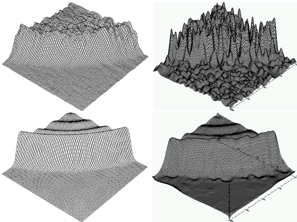
圖 2-10 利用多重尺度之複雜現象的理想化試驗數據進行不同資料同化（或客觀分析）的比較。上圖左為 Barnes 方法、上圖右為現行的 3DVAR 方法、下圖左為理想化試驗數據圖、下圖右為連續變分方法
