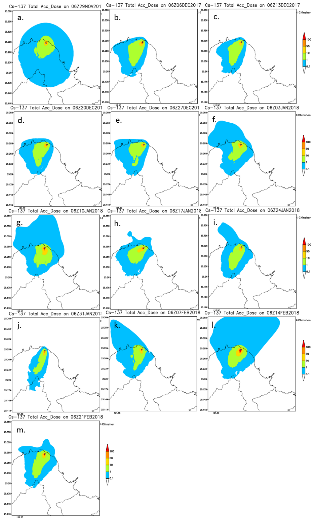
圖 4-2 核一廠冬季，自 2017 年 11 月 29 日至 2018 年 2 月 27 日 Cs-137 假想事故模擬之 7 日有效劑量累積圖(mSv)。
