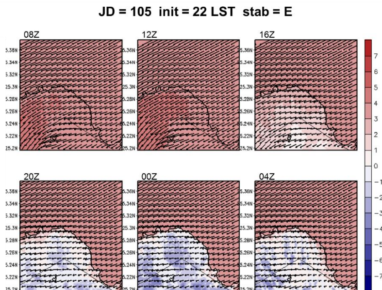
圖 5-80 A2Cflow 調校後之模擬(20m 高)風場，模擬日期太陽日為第 105 日，模擬初始時間為 20LST，中心位置為核一廠(第 4 層巢狀網格)，風向為 45^\circ ，風速為 8m/s，穩定度參數為 0.005(穩定度分類 ED 級)，填色部分為溫度擾動，單位為 ^\circ\text{C} 。
