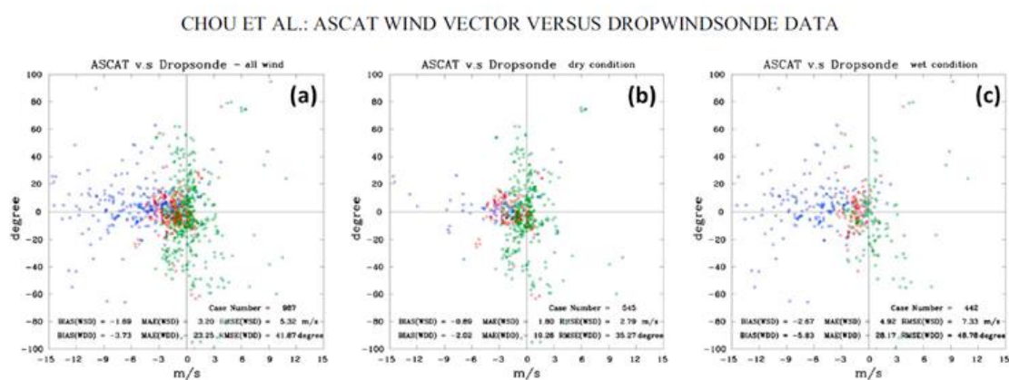
圖 6-2 ASCAT 與投落送於不同溼度條件兩者風向與風速相關性比較。左圖為全部資料，中與右圖為區分為乾燥與潮溼環境。顯示風速在 12~18 m/s 資料品質最好，弱風速時風向 bias 較大，強風速時風速易低估(綠點為風速小於 12 m/s，紅點 12~18m/s，藍點為大於 18 m/s)。
