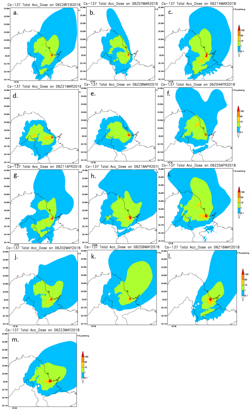
圖 4-14 核二廠春季，自 2018 年 2 月 28 日至 2018 年 5 月 23 日 Cs-137 假想事故模擬之 7 日有效劑量累積圖(mSv)。
