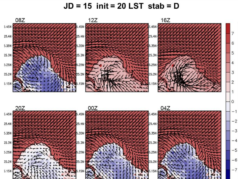
圖 5-3 A2Cflow 調校後之模擬(20m 高)風場，模擬日期太陽日為第 15 日，模擬初始時間為 20LST，中心位置為核一廠(第 3 層巢狀網格)，風向為 45^\circ ，風速為 2m/s，穩定度參數為 0.002(穩定度分類 D 級)；填色部分為溫度擾動，單位為 ^\circ\text{C} 。
