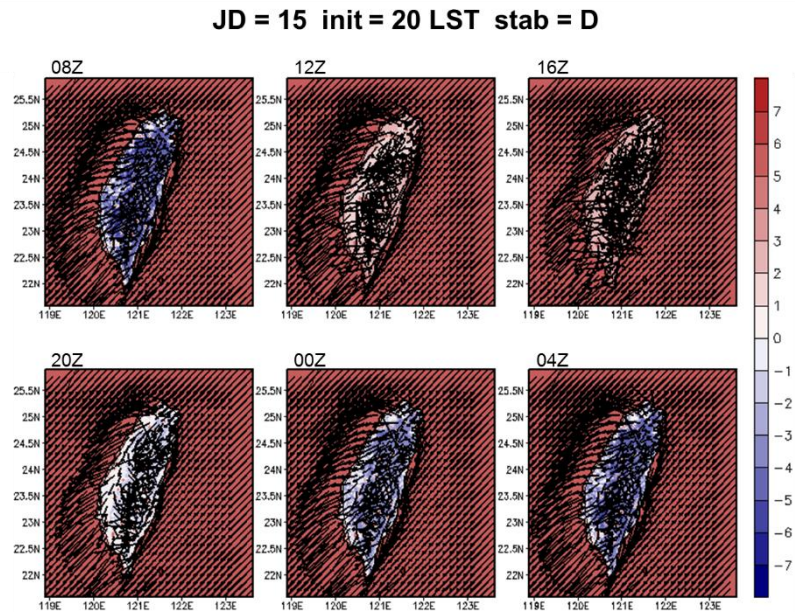
圖 5-1 A2Cflow 調校後之模擬(20m 高)風場，模擬日期太陽日為第 15 日，模擬初始時間為 20LST，中心位置為核一廠(第 1 層巢狀網格)，風向為 45^\circ ，風速為 2m/s，穩定度參數為 0.002(穩定度分類 D 級)；填色部分為溫度擾動，單位為 ^\circ\text{C} 。
