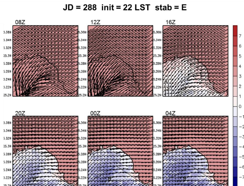
圖 5-32 A2Cflow 調校後之模擬(20m 高)風場，模擬日期太陽日為第 288 日，模擬初始時間為 22LST，中心位置為核一廠(第 4 層巢狀網格)，風向為 45^\circ ，風速為 2m/s，穩定度參數為 0.005(穩定度分類 E 級)，填色部分為溫度擾動，單位為 ^\circ\text{C} 。
