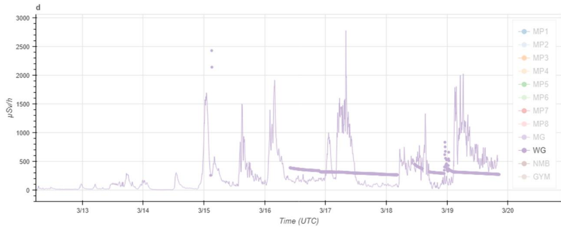
圖 7-9 福島電廠 WG 測站劑量率模擬結果
