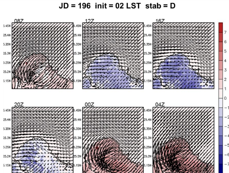
圖 5-19 A2Cflow 調校後之模擬(20m 高)風場，模擬日期太陽日為第 196 日，模擬初始時間為 02LST，中心位置為核一廠(第 3 層巢狀網格)，風向為 45^\circ ，風速為 2m/s，穩定度參數為 0.002(穩定度分類 D 級)；填色部分為溫度擾動，單位為 ^\circ\text{C} 。
