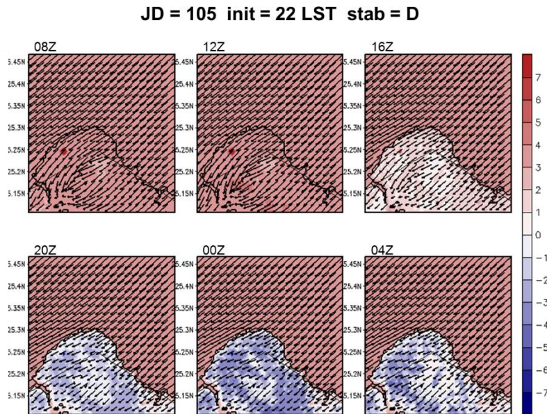
圖 5-75 A2Cflow 調校後之模擬(20m 高)風場，模擬日期太陽日為第 105 日，模擬初始時間為 20LST，中心位置為核一廠(第 3 層巢狀網格)，風向為 45^\circ ，風速為 8m/s，穩定度參數為 0.002(穩定度分類 D 級)，填色部分為溫度擾動，單位為 ^\circ\text{C} 。
