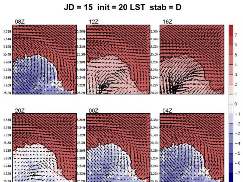
圖 5-4 A2Cflow 調校後之模擬(20m 高)風場，模擬日期太陽日為第 15 日，模擬初始時間為 20LST，中心位置為核一廠(第 4 層巢狀網格)，風向為 45^\circ ，風速為 2m/s，穩定度參數為 0.002(穩定度分類 D 級)；填色部分為溫度擾動，單位為 ^\circ\text{C} 。
