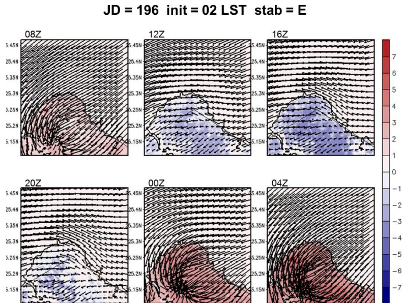
圖 5-23 A2Cflow 調校後之模擬(20m 高)風場，模擬日期太陽日為第 196 日，模擬初始時間為 02LST，中心位置為核一廠(第 3 層巢狀網格)，風向為 45^\circ ，風速為 2m/s，穩定度參數為 0.005(穩定度分類 E 級)，填色部分為溫度擾動，單位為 ^\circ\text{C} 。
