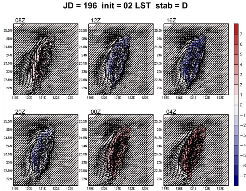
圖 5-49 A2Cflow 調校後之模擬(20m 高)風場，模擬日期太陽日為第 196 日，模擬初始時間為 02LST，中心位置為核一廠(第 1 層巢狀網格)，風向為 45^\circ ，風速為 5m/s，穩定度參數為 0.002(穩定度分類 D 級)，填色部分為溫度擾動，單位為 ^\circ\text{C} 。
