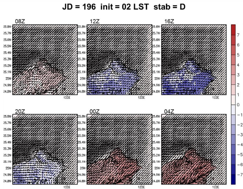
圖 5-82 A2Cflow 調校後之模擬(20m 高)風場，模擬日期太陽日為第 196 日，模擬初始時間為 20LST，中心位置為核一廠(第 2 層巢狀網格)，風向為 45^\circ ，風速為 8m/s，穩定度參數為 0.002(穩定度分類 D 級)，填色部分為溫度擾動，單位為 ^\circ\text{C} 。
