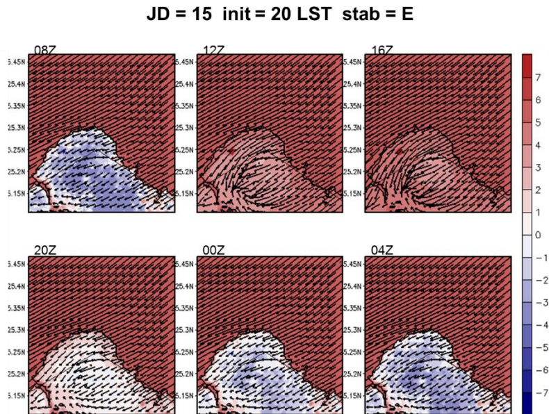
圖 5-39 A2Cflow 調校後之模擬(20m 高)風場，模擬日期太陽日為第 15 日，模擬初始時間為 20LST，中心位置為核一廠(第 3 層巢狀網格)，風向為 45^\circ ，風速為 5m/s，穩定度參數為 0.005(穩定度分類 E 級)，填色部分為溫度擾動，單位為 ^\circ\text{C} 。
