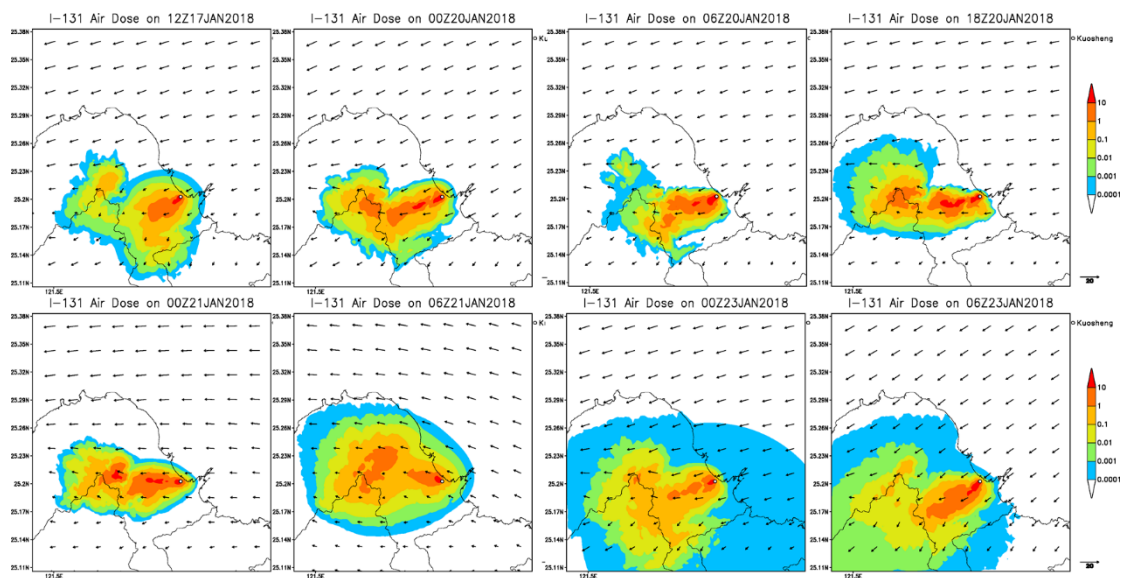
圖 4-7 2018 年 1 月 17 日當周，I-131 假想模擬中，劑量累積在大屯山的空氣劑量率及風場。
