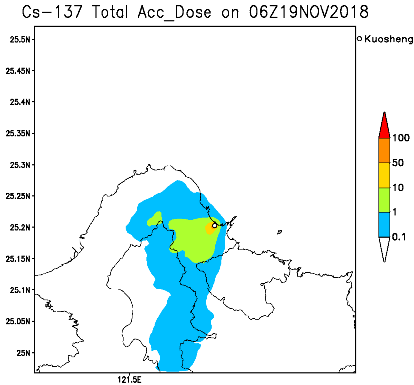
圖 7-24 核二廠 Cs-137 核種假想事故於 2018/11/19 七天有效劑量累積分布(mSv)
