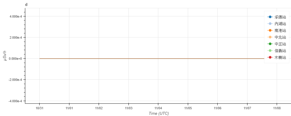
圖 7-23 核一廠在台北測站扣掉背景範圍值後劑量率模擬結果
