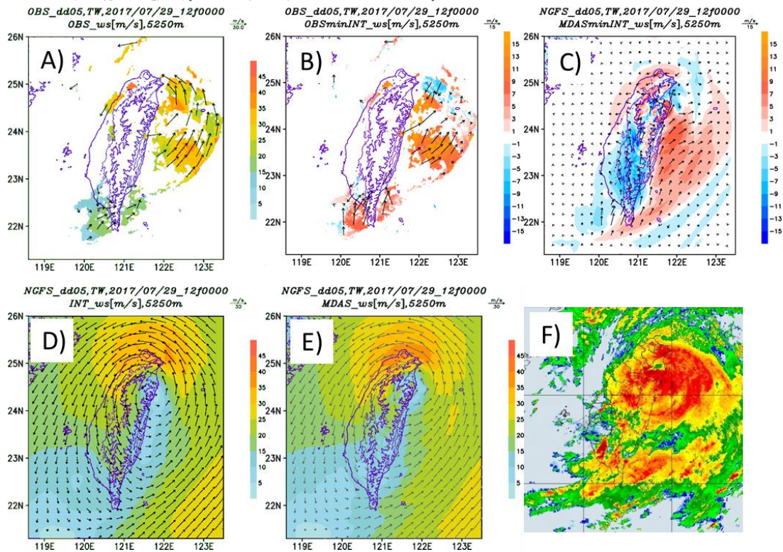
圖 6-12 2017 尼莎颱風 5250 公尺風速。(A)QPESUMS 雷達反演風、(B)QPESUMS 雷達反演風減初始猜測場、(C)MDAS 減初始猜測場、(D)初始猜測場、(E)MDAS 與(F) 合成雷達迴波；(A)(D)(E)風標為向量，(B)(C)風標為向量差。
