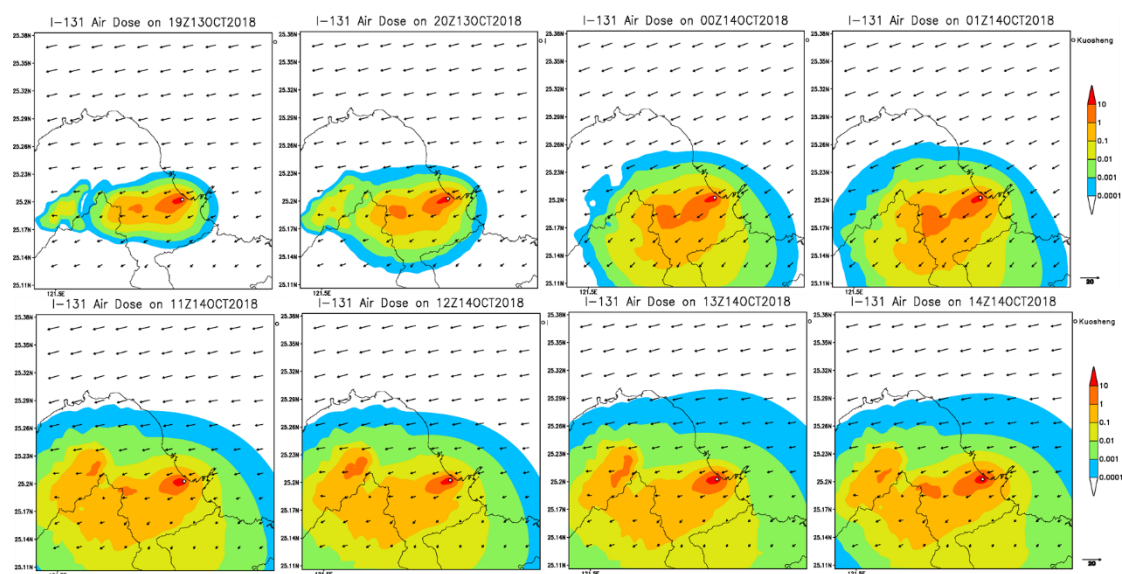
圖 4-34 2018 年 10 月 10 日當周，假想模擬中，I-131 劑量累積在大屯山區的空氣劑量率(mSv/hr)及風場。
