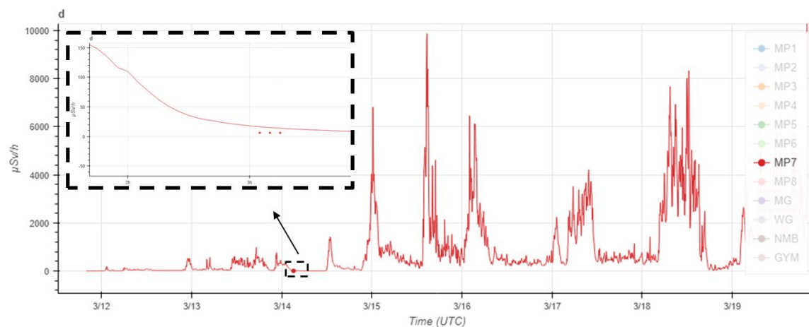
圖 7-16 福島電廠 MP7 測站劑量率模擬結果
