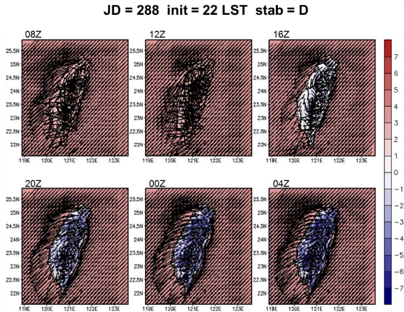
圖 5-25 A2Cflow 調校後之模擬(20m 高)風場，模擬日期太陽日為第 288 日，模擬初始時間為 02LST，中心位置為核一廠(第 1 層巢狀網格)，風向為 45^\circ ，風速為 2m/s，穩定度參數為 0.002(穩定度分類 D 級)，填色部分為溫度擾動，單位為 ^\circ\text{C} 。
