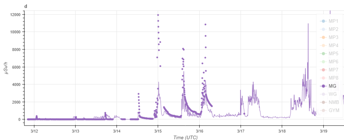
圖 7-6 福島電廠 MG 測站劑量率模擬結果
