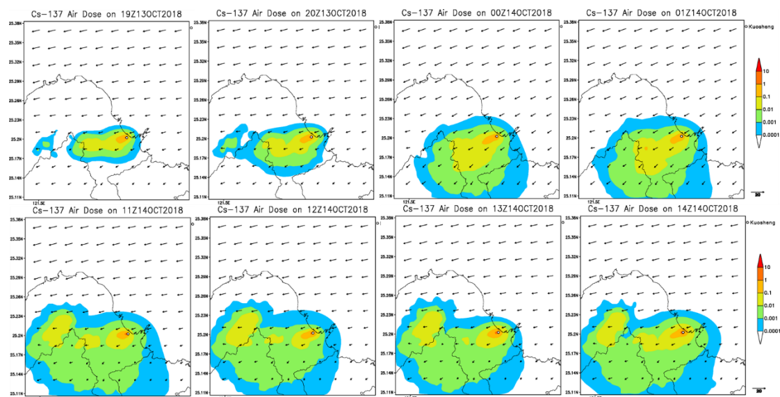
圖 4-33 2018 年 10 月 10 日當周，假想模擬中，Cs-137 核種累積在大屯山區的空氣劑量率(mSv/hr)及風場。
