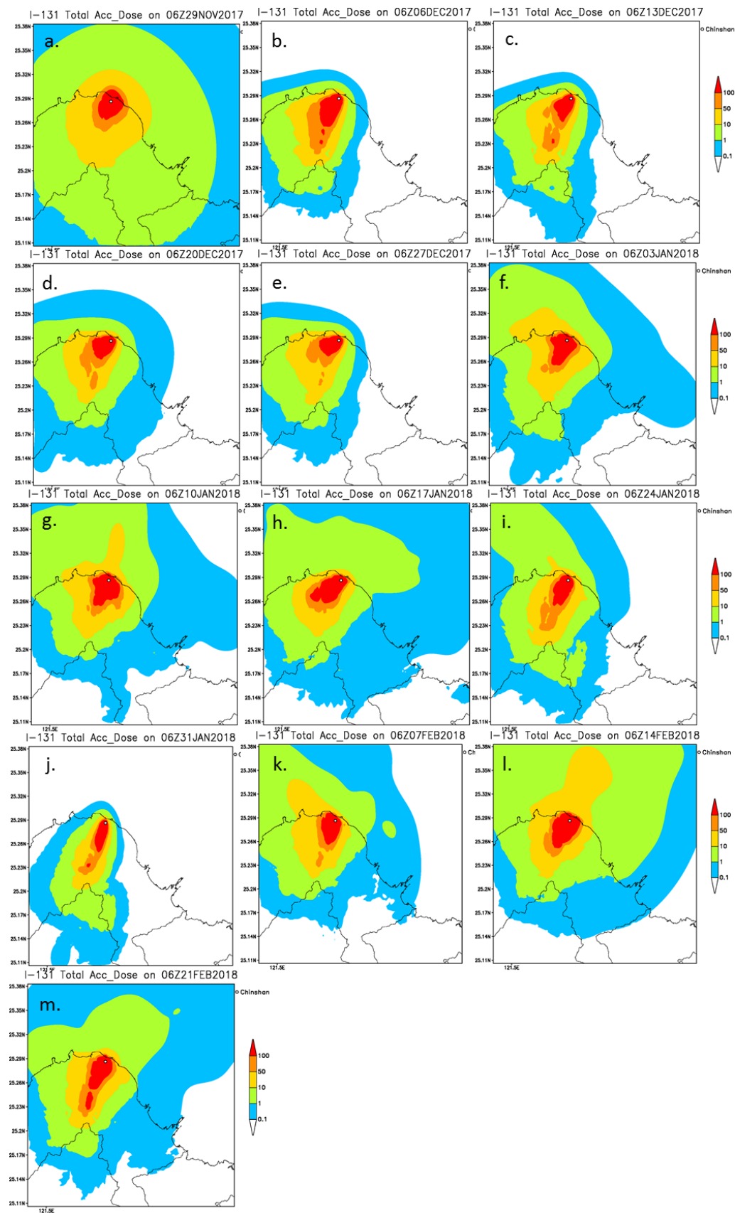
圖 4-3 核一廠冬季，自 2017 年 11 月 29 日至 2018 年 2 月 27 日 I-131 假想事故模擬之 7 日有效劑量累積圖(mSv)。
