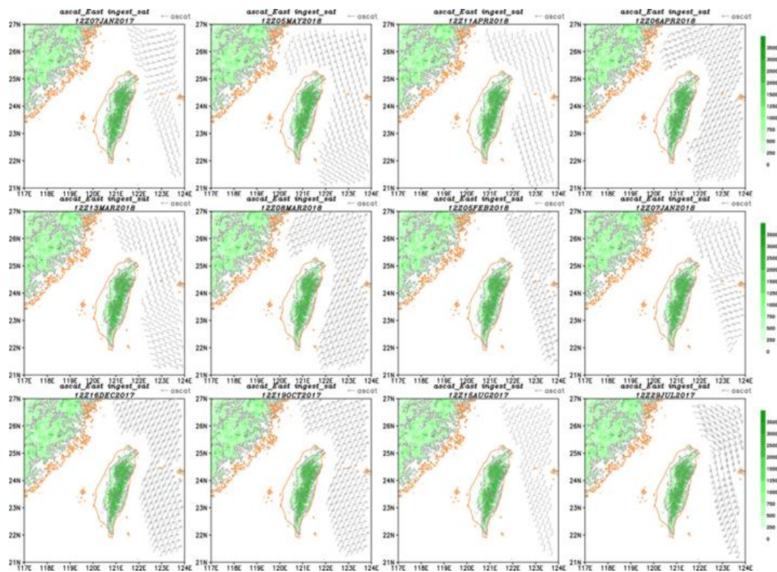
圖 6-3 ASCAT 海面風場資料不同時間點經品質控制後示意圖。品質控制策略不採用風速低於 2m/s 的觀測資料，並移除陸地及近海岸的觀測資料。
