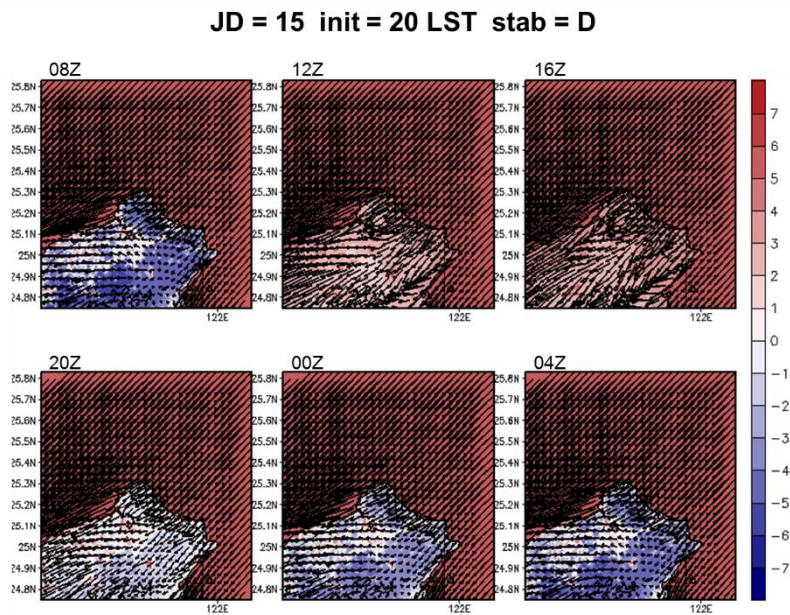
圖 5-34 A2Cflow 調校後之模擬(20m 高)風場，模擬日期太陽日為第 15 日，模擬初始時間為 20LST，中心位置為核一廠(第 2 層巢狀網格)，風向為 45^\circ ，風速為 5m/s，穩定度參數為 0.002(穩定度分類 D 級)，填色部分為溫度擾動，單位為 ^\circ\text{C} 。
