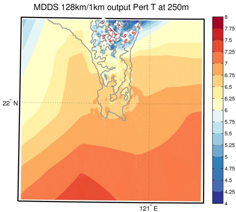
圖 3-27 MDDS 核三廠第一層巢狀網格(1 公里解析度)溫度擾動場。同樣受到冷高壓影響，南北溫度梯度較大，由北到南分別由低溫到高溫，同樣可以看到隨著解析度的增加，越能解析出溫度擾動場在地形上面的變化，地形越高溫度越低。
