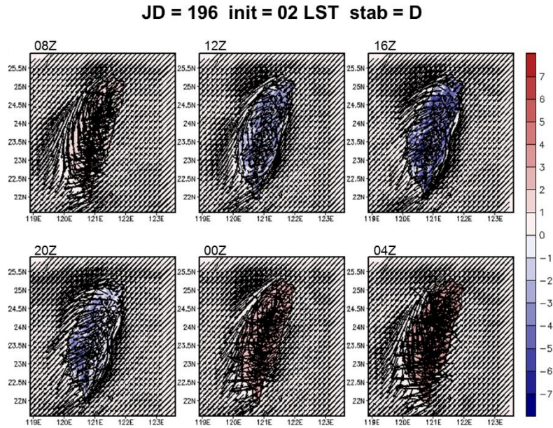
圖 5-17 A2Cflow 調校後之模擬(20m 高)風場，模擬日期太陽日為第 196 日，模擬初始時間為 02LST，中心位置為核一廠(第 1 層巢狀網格)，風向為 45^\circ ，風速為 2m/s，穩定度參數為 0.002(穩定度分類 D 級)；填色部分為溫度擾動，單位為 ^\circ\text{C} 。
