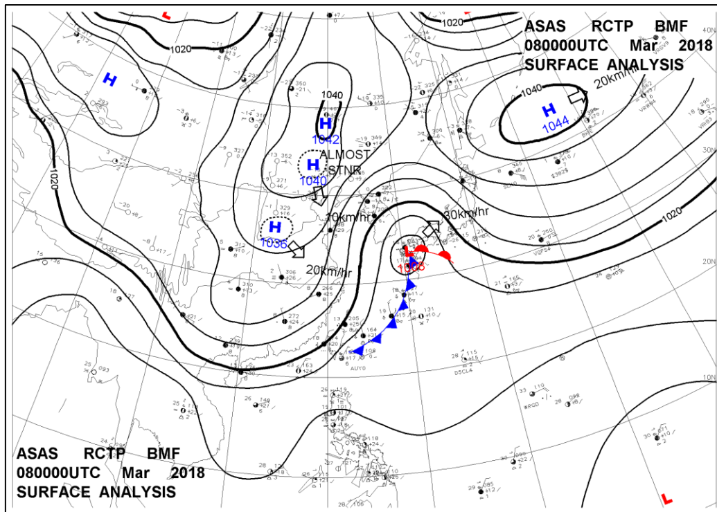
圖 3-19 2018 年 3 月 8 號地面天氣圖，其時間台灣正被冷鋒後的冷高壓勢力所籠罩，全台灣風場均為較強烈的東北風。
