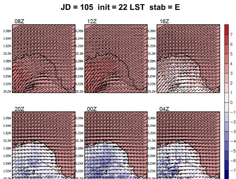
圖 5-48 A2Cflow 調校後之模擬(20m 高)風場，模擬日期太陽日為第 105 日，模擬初始時間為 22LST，中心位置為核一廠(第 4 層巢狀網格)，風向為 45^\circ ，風速為 5m/s，穩定度參數為 0.005(穩定度分類 E 級)，填色部分為溫度擾動，單位為 ^\circ\text{C} 。
