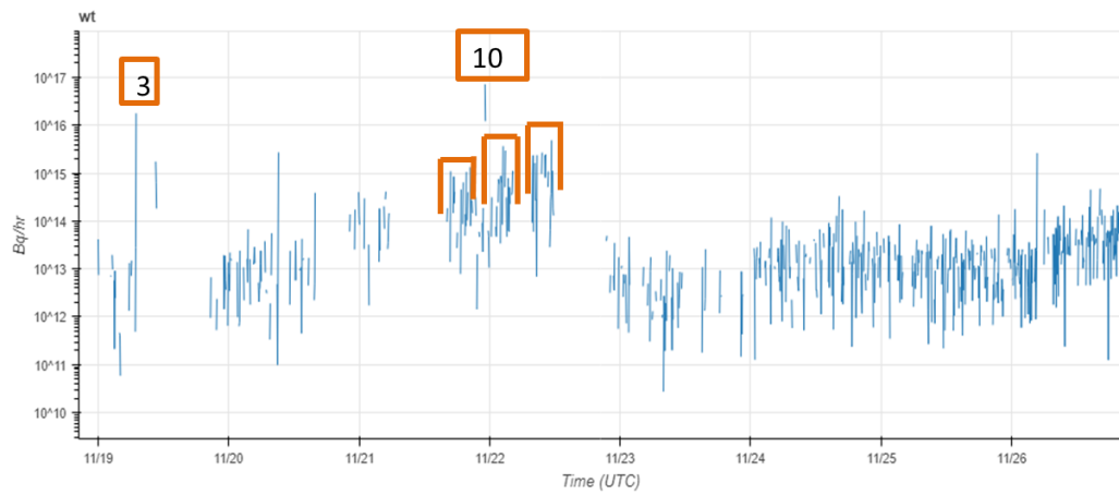
圖 7-26 福島事件外釋於核二廠後用臺灣測站回推出釋放率結果
