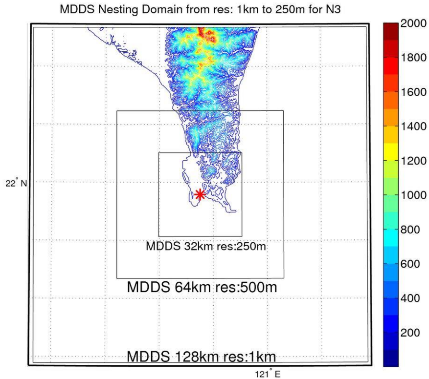
圖 3-18 核三廠區 MDDS 3 層巢狀網格區範圍圖。最外圍的黑色框為 MDDS 第一層巢狀網格 1 公里解析度共 128 公里範圍，其次黑色框為 MDDS 第二層巢狀網格 500 公尺解析度共 64 公里範圍，最小的黑色框為 MDDS 第三層巢狀網格 250 公尺解析度 32 公里範圍
