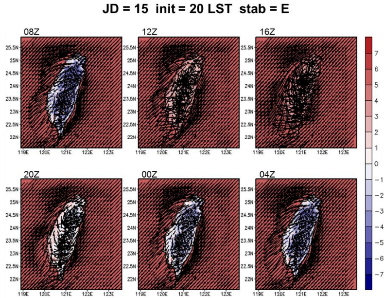
圖 5-5 A2Cflow 調校後之模擬(20m 高)風場，模擬日期太陽日為第 15 日，模擬初始時間為 20LST，中心位置為核一廠(第 1 層巢狀網格)，風向為 45^\circ ，風速為 2m/s，穩定度參數為 0.005(穩定度分類 E 級)；填色部分為溫度擾動，單位為 ^\circ\text{C} 。
