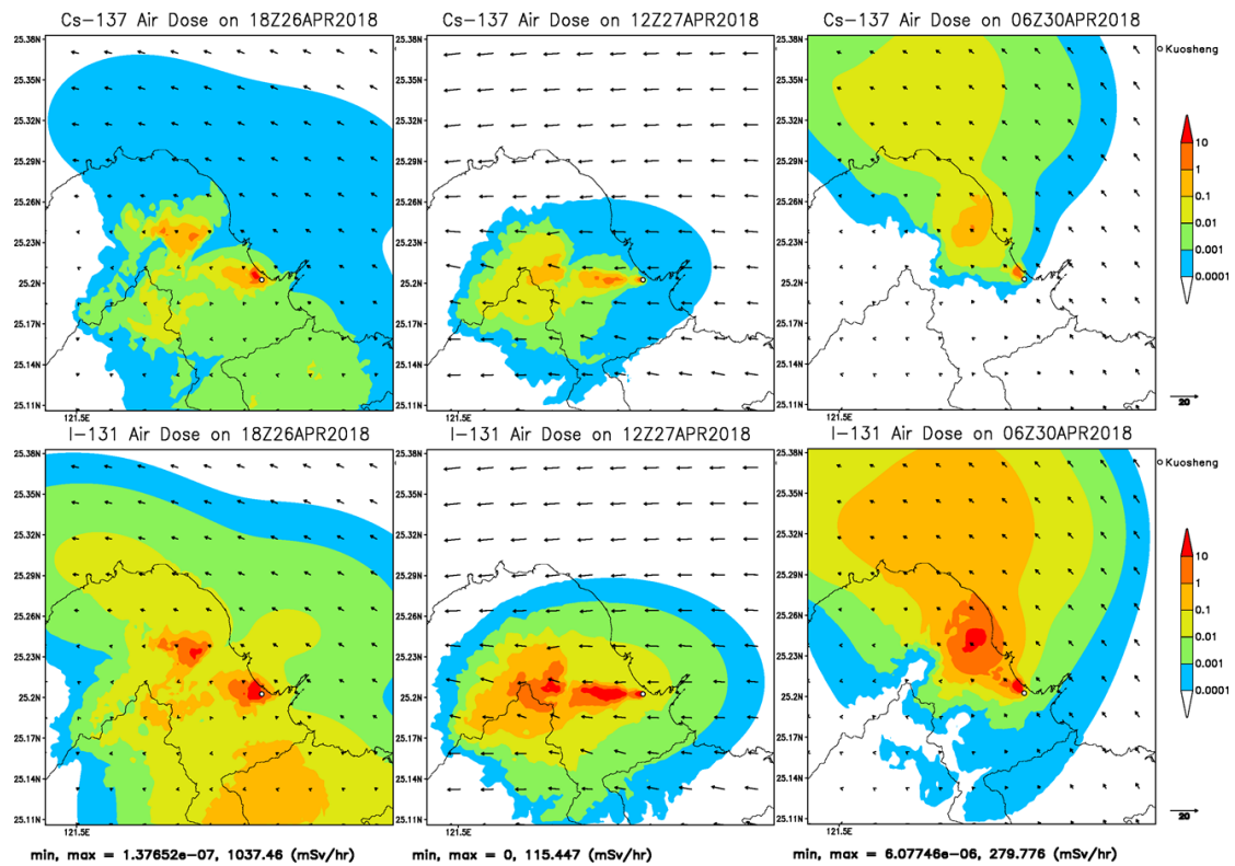
圖 4-18 2018 年 4 月 25 日當周，假想模擬中，劑量累積在大屯山的空氣劑量率及風場。上半部:Cs-137，下半部:I-131
