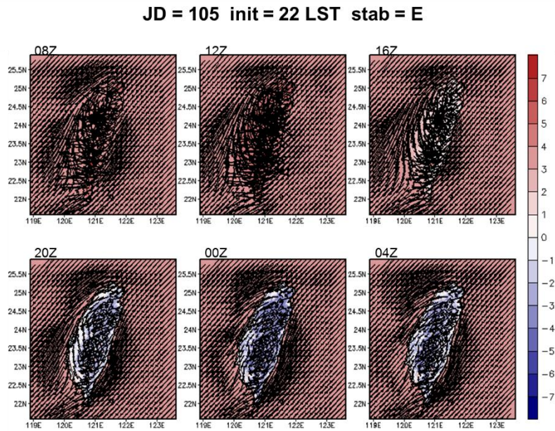
圖 5-13 A2Cflow 調校後之模擬(20m 高)風場，模擬日期太陽日為第 105 日，模擬初始時間為 22LST，中心位置為核一廠(第 1 層巢狀網格)，風向為 45^\circ ，風速為 2m/s，穩定度參數為 0.005(穩定度分類 E 級)；填色部分為溫度擾動，單位為 ^\circ\text{C} 。
