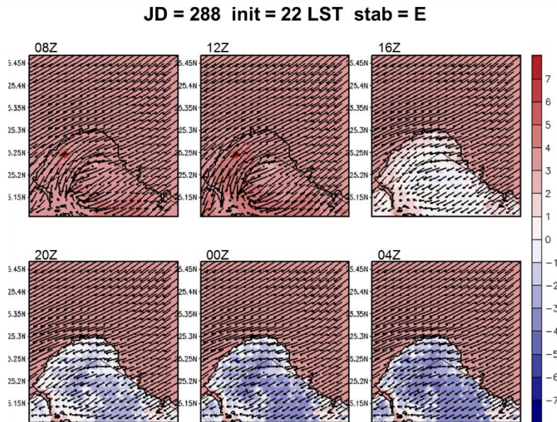
圖 5-63 A2Cflow 調校後之模擬(20m 高)風場，模擬日期太陽日為第 288 日，模擬初始時間為 22LST，中心位置為核一廠(第 3 層巢狀網格)，風向為 45^\circ ，風速為 5m/s，穩定度參數為 0.005(穩定度分類 E 級)，填色部分為溫度擾動，單位為 ^\circ\text{C} 。
