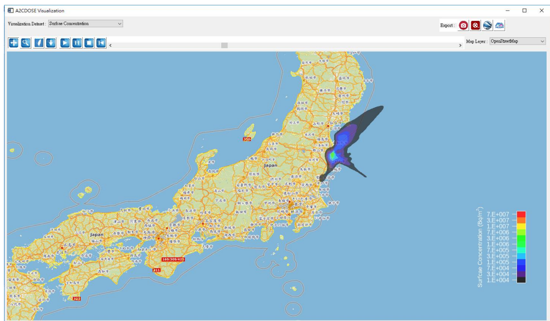
圖 3-11 日本福島案例地表濃度分布顯示
