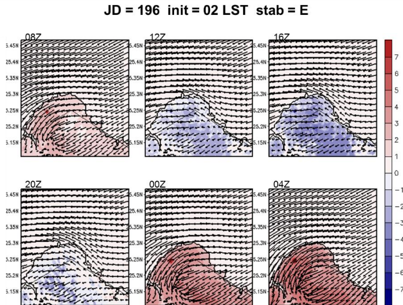
圖 5-55 A2Cflow 調校後之模擬(20m 高)風場，模擬日期太陽日為第 196 日，模擬初始時間為 02LST，中心位置為核一廠(第 3 層巢狀網格)，風向為 45^\circ ，風速為 5m/s，穩定度參數為 0.005(穩定度分類 E 級)，填色部分為溫度擾動，單位為 ^\circ\text{C} 。
