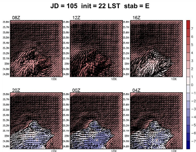
圖 5-14 A2Cflow 調校後之模擬(20m 高)風場，模擬日期太陽日為第 105 日，模擬初始時間為 22LST，中心位置為核一廠(第 2 層巢狀網格)，風向為 45^\circ ，風速為 2m/s，穩定度參數為 0.005(穩定度分類 E 級)；填色部分為溫度擾動，單位為 ^\circ\text{C} 。
