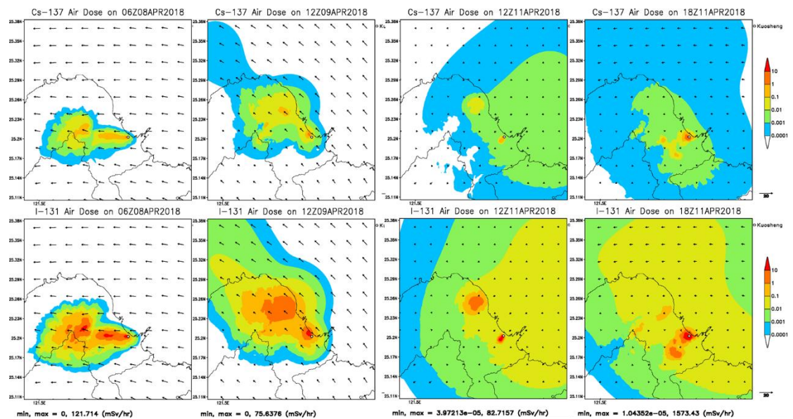
圖 4-17 2018 年 4 月 4 日當周，假想模擬中，劑量累積在大屯山的空氣劑量率及風場。上半部:Cs-137，下半部:I-131
