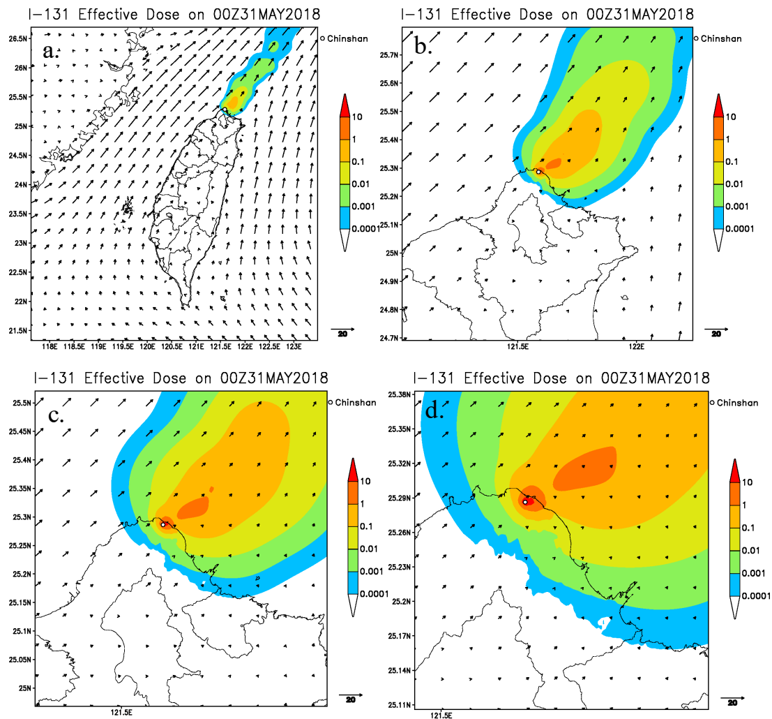
圖 3-15 核一廠 4 層巢狀網格之劑量評估系統結果，圖為 2018/05/30 I-131 的假想案例模擬，預報 24 小時後(2018/05/31)的有效劑量率分布，單位:mSv/hr。由左至右，由上至下依序為 a. 解析度 2.5 公里 b.解析度 1 公里 c.解析度 500 公尺 d.解析度 250 公尺。
