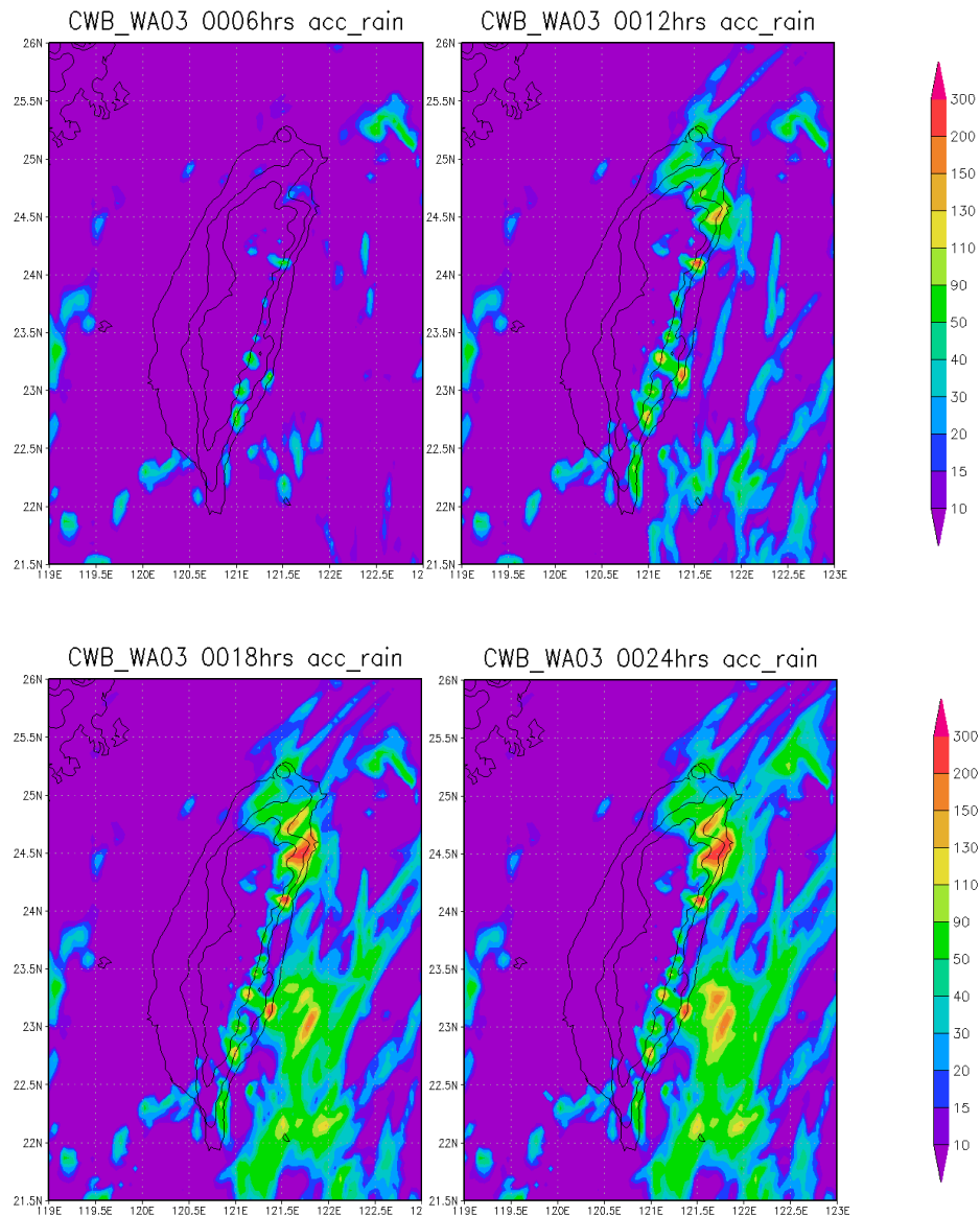
圖 3-31 2018 年 9 月 24 日 CWB WRF 每六小時累積降雨預報分布圖 (mm)，水平解析度為 5 公里。
