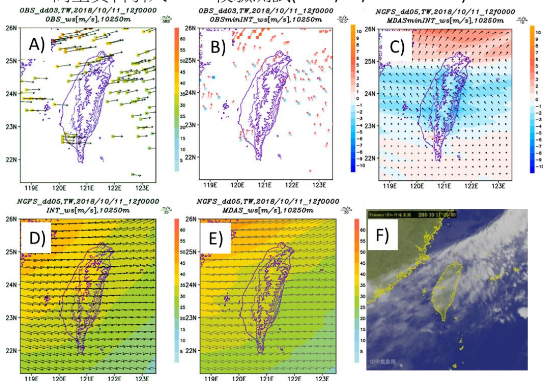
圖 6-6 2018 東北季風(10/11)10250 公尺風速。(A)傳統高空觀測資料、(B)觀測資料減初始猜測場、(C)MDAS 減初始猜測場、(D)初始猜測場、(E)MDAS 與(F)衛星雲圖；(A)(D)(E)風標為向量，(B)(C)風標為向量差。
