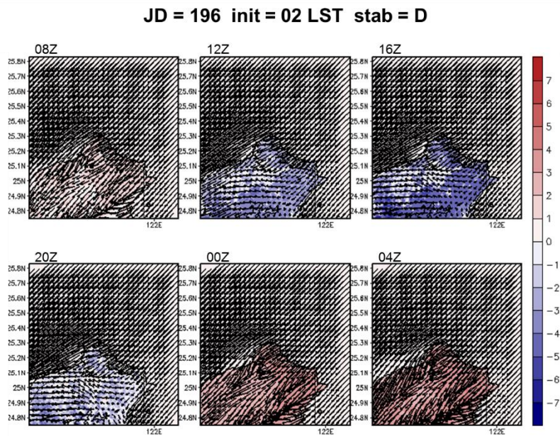
圖 5-50 A2Cflow 調校後之模擬(20m 高)風場，模擬日期太陽日為第 196 日，模擬初始時間為 02LST，中心位置為核一廠(第 2 層巢狀網格)，風向為 45^\circ ，風速為 5m/s，穩定度參數為 0.002(穩定度分類 D 級)，填色部分為溫度擾動，單位為 ^\circ\text{C} 。
