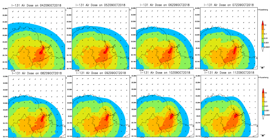
圖 4-32 2018 年 10 月 3 日當周，假想模擬中，I-131 劑量累積在大屯山的空氣劑量率(mSv/hr)及風場。
