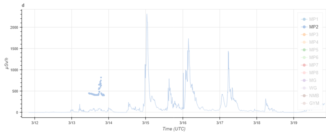
圖 7-11 福島電廠 MP2 測站劑量率模擬結果
