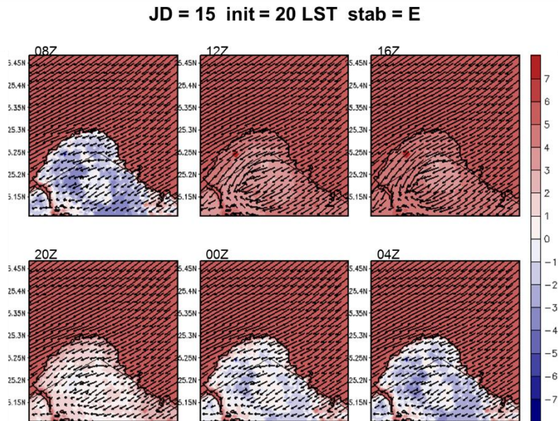
圖 5-71 A2Cflow 調校後之模擬(20m 高)風場，模擬日期太陽日為第 15 日，模擬初始時間為 20LST，中心位置為核一廠(第 3 層巢狀網格)，風向為 45^\circ ，風速為 8m/s，穩定度參數為 0.005(穩定度分類 ED 級)，填色部分為溫度擾動，單位為 ^\circ\text{C} 。
