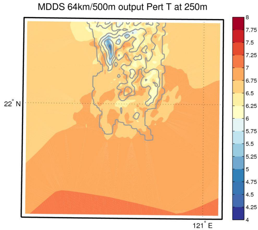
圖 3-28 MDDS 核三廠第二層巢狀網格(500 公尺解析度)溫度擾動場
