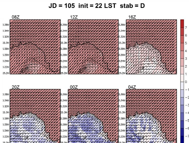
圖 5-76 A2Cflow 調校後之模擬(20m 高)風場，模擬日期太陽日為第 105 日，模擬初始時間為 20LST，中心位置為核一廠(第 4 層巢狀網格)，風向為 45^\circ ，風速為 8m/s，穩定度參數為 0.002(穩定度分類 D 級)，填色部分為溫度擾動，單位為 ^\circ\text{C} 。
