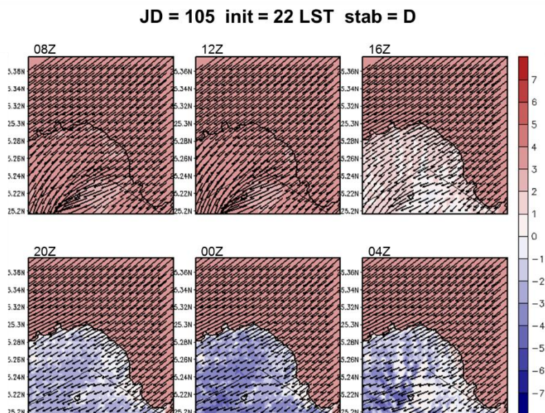
圖 5-44 A2Cflow 調校後之模擬(20m 高)風場，模擬日期太陽日為第 105 日，模擬初始時間為 22LST，中心位置為核一廠(第 4 層巢狀網格)，風向為 45^\circ ，風速為 5m/s，穩定度參數為 0.002(穩定度分類 D 級)，填色部分為溫度擾動，單位為 ^\circ\text{C} 。
