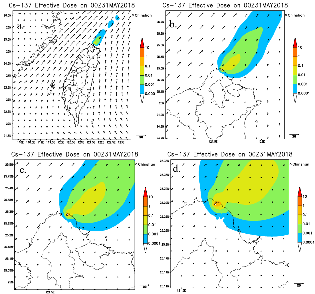
圖 3-12 核一廠 4 層巢狀網格之劑量評估系統結果，圖為 2018/05/30 Cs-137 的假想案例模擬，預報 24 小時後(2018/05/31)的有效劑量率分布，單位:mSv/hr。由左至右，由上至下依序為 a. 解析度 2.5 公里 b.解析度 1 公里 c.解析度 500 公尺 d.解析度 250 公尺。
