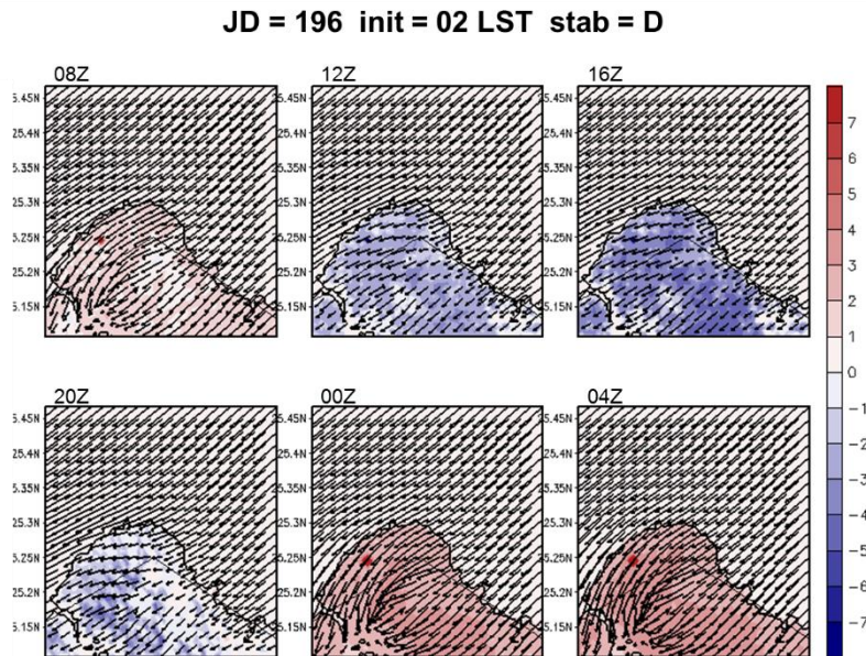
圖 5-51 A2Cflow 調校後之模擬(20m 高)風場，模擬日期太陽日為第 196 日，模擬初始時間為 02LST，中心位置為核一廠(第 3 層巢狀網格)，風向為 45^\circ ，風速為 5m/s，穩定度參數為 0.002(穩定度分類 D 級)，填色部分為溫度擾動，單位為 ^\circ\text{C} 。
