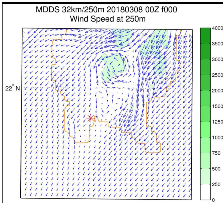
圖 3-22 MDDS 核三廠第三層巢狀網格(250 公尺解析度)風場圖。隨著解析度的增加，可以看到 MDDS 解析出東北風系遇到大佛山所形成的繞流及渦漩。墾丁一帶則因為地勢較為平緩仍維持東北風系。
