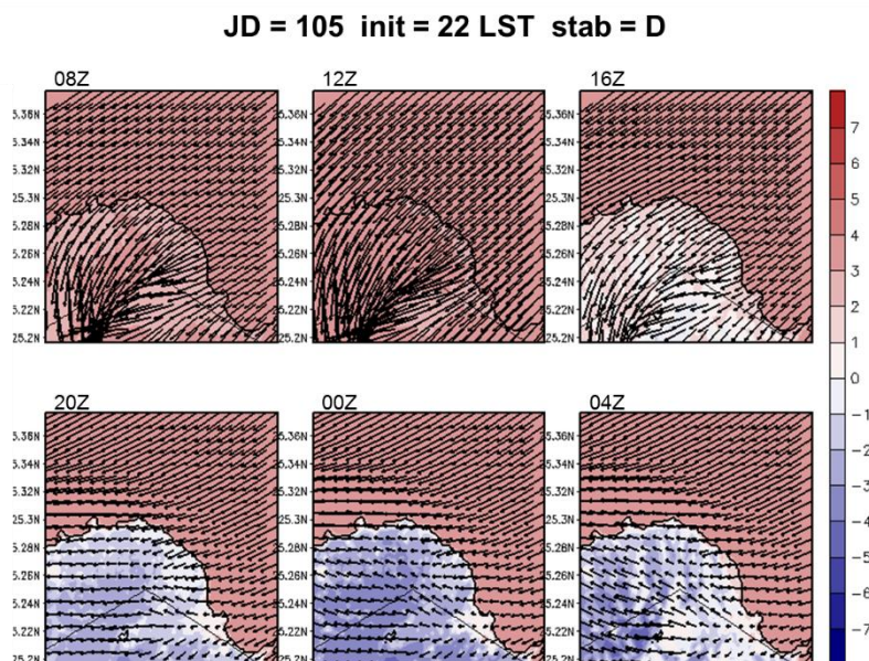
圖 5-12 A2Cflow 調校後之模擬(20m 高)風場，模擬日期太陽日為第 105 日，模擬初始時間為 22LST，中心位置為核一廠(第 4 層巢狀網格)，風向為 45^\circ ，風速為 2m/s，穩定度參數為 0.002(穩定度分類 D 級)；填色部分為溫度擾動，單位為 ^\circ\text{C} 。
