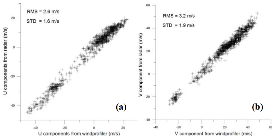
圖6-9 辛樂克(2008)、薔蜜(2008)及莫拉克(2009)颱風所有分析高度之雙都卜勒反演風速與與那國島剖風儀風速觀測散布圖，顯示雷達反演風場資料與剖風儀觀測資料相近。(a)為東西風分量，(b)為南北風分量。(摘自張，2014)
