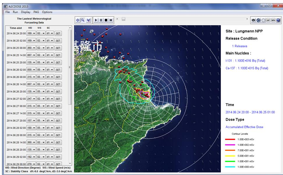
圖 2-6 劑量評估系統 2016 年版介面
