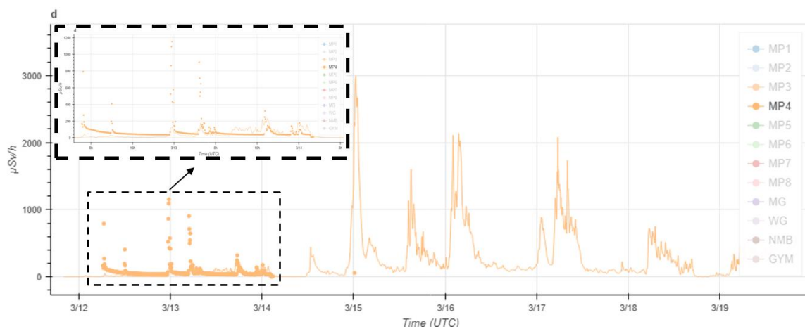
圖 7-13 福島電廠 MP4 測站劑量率模擬結果
