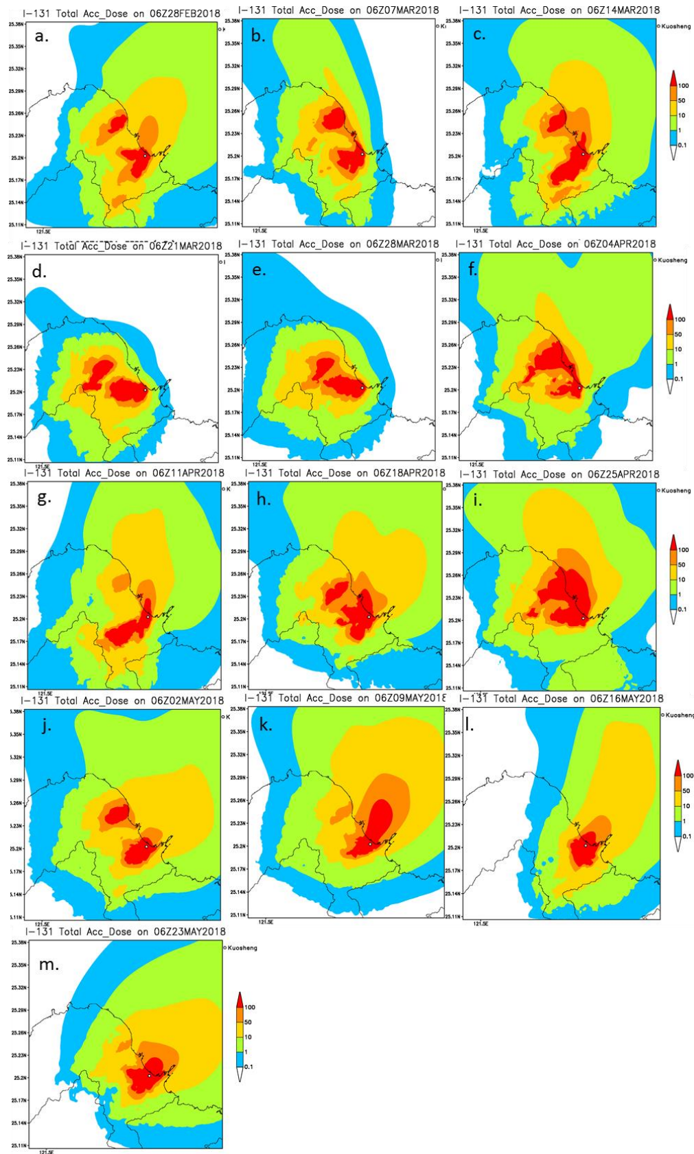
圖 4-15 核二廠春季，自 2018 年 2 月 28 日至 2018 年 5 月 23 日 I-131 假想事故模擬之 7 日有效劑量累積圖(mSv)。
