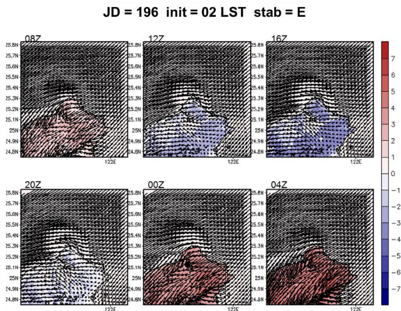
圖 5-54 A2Cflow 調校後之模擬(20m 高)風場，模擬日期太陽日為第 196 日，模擬初始時間為 02LST，中心位置為核一廠(第 2 層巢狀網格)，風向為 45^\circ ，風速為 5m/s，穩定度參數為 0.005(穩定度分類 E 級)，填色部分為溫度擾動，單位為 ^\circ\text{C} 。
