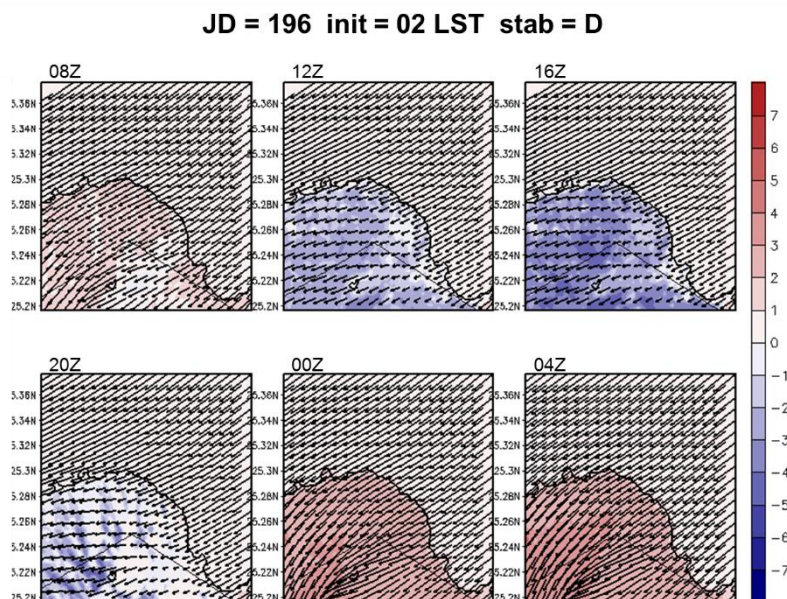
圖 5-52 A2Cflow 調校後之模擬(20m 高)風場，模擬日期太陽日為第 196 日，模擬初始時間為 02LST，中心位置為核一廠(第 4 層巢狀網格)，風向為 45^\circ ，風速為 5m/s，穩定度參數為 0.002(穩定度分類 D 級)，填色部分為溫度擾動，單位為 ^\circ\text{C} 。
