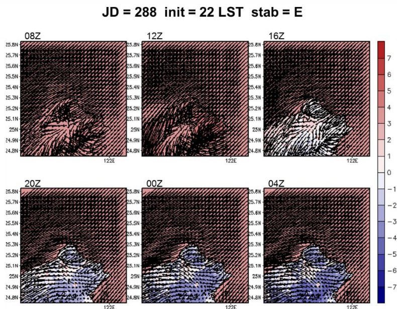
圖 5-30 A2Cflow 調校後之模擬(20m 高)風場，模擬日期太陽日為第 288 日，模擬初始時間為 22LST，中心位置為核一廠(第 2 層巢狀網格)，風向為 45^\circ ，風速為 2m/s，穩定度參數為 0.005(穩定度分類 E 級)，填色部分為溫度擾動，單位為 ^\circ\text{C} 。
