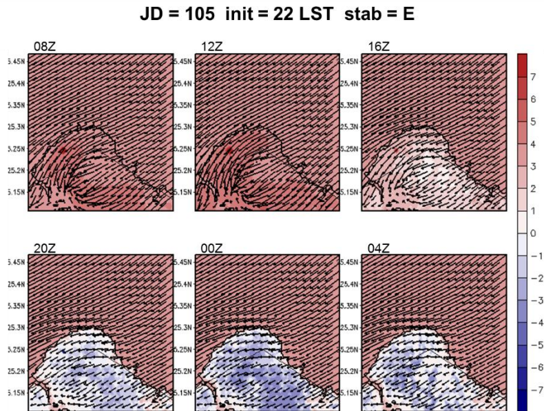
圖 5-47 A2Cflow 調校後之模擬(20m 高)風場，模擬日期太陽日為第 105 日，模擬初始時間為 22LST，中心位置為核一廠(第 3 層巢狀網格)，風向為 45^\circ ，風速為 5m/s，穩定度參數為 0.005(穩定度分類 E 級)，填色部分為溫度擾動，單位為 ^\circ\text{C} 。
