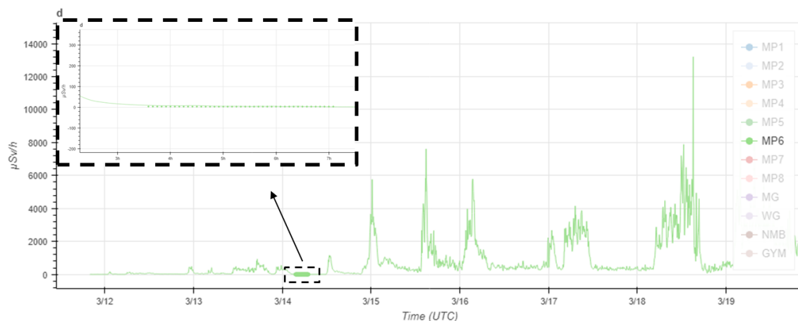
圖 7-15 福島電廠 MP6 測站劑量率模擬結果
