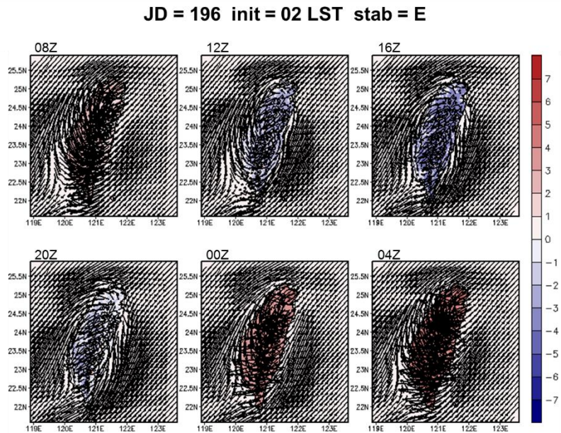
圖 5-21 A2Cflow 調校後之模擬(20m 高)風場，模擬日期太陽日為第 196 日，模擬初始時間為 02LST，中心位置為核一廠(第 1 層巢狀網格)，風向為 45^\circ ，風速為 2m/s，穩定度參數為 0.005(穩定度分類 E 級)，填色部分為溫度擾動，單位為 ^\circ\text{C} 。
