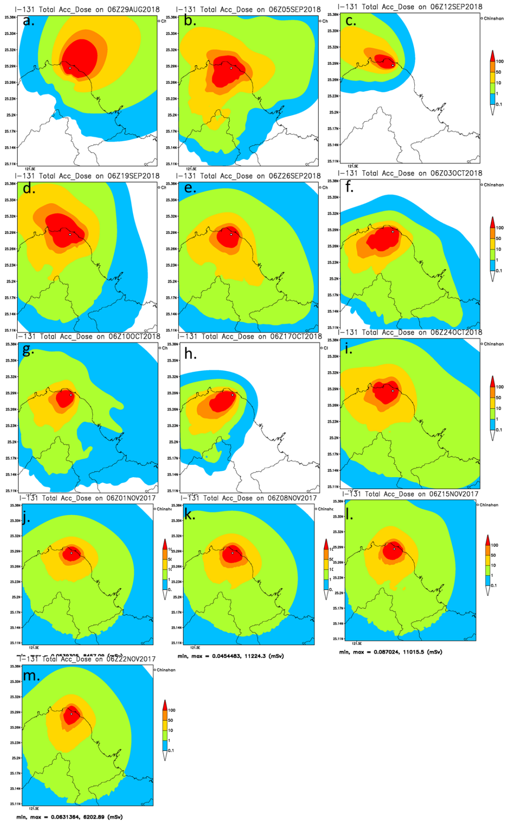
圖 4-26 核一廠秋季，自 2018 年 8 月 29 日至 2018 年 10 月 30 日和 2017 年 11 月 1 日至 11 月 29 日 I-131 假想事故模擬之 7 日有效劑量累積圖(mSv)。
