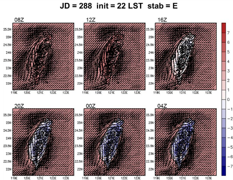
圖 5-61 A2Cflow 調校後之模擬(20m 高)風場，模擬日期太陽日為第 288 日，模擬初始時間為 22LST，中心位置為核一廠(第 1 層巢狀網格)，風向為 45^\circ ，風速為 5m/s，穩定度參數為 0.005(穩定度分類 E 級)，填色部分為溫度擾動，單位為 ^\circ\text{C} 。
