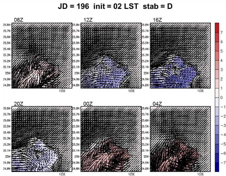
圖 5-18 A2Cflow 調校後之模擬(20m 高)風場，模擬日期太陽日為第 196 日，模擬初始時間為 02LST，中心位置為核一廠(第 2 層巢狀網格)，風向為 45^\circ ，風速為 2m/s，穩定度參數為 0.002(穩定度分類 D 級)；填色部分為溫度擾動，單位為 ^\circ\text{C} 。
