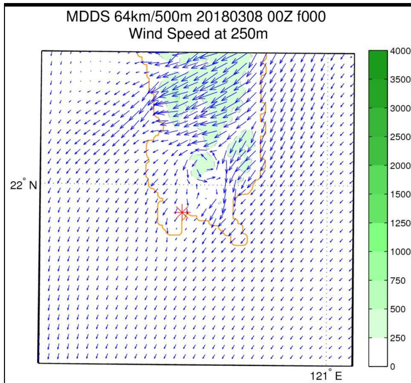
圖 3-21 MDDS 核三廠第二層巢狀網格(500 公尺解析度)風場圖。
