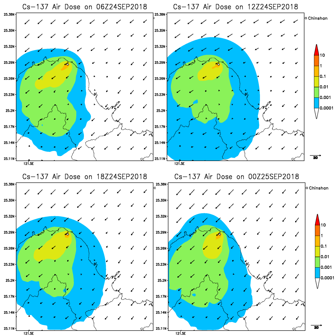
圖 3-32 2018 年 9 月 24 日僅有乾沉降過程之每六小時之空氣劑量率 (mSv/hr) 分布。
