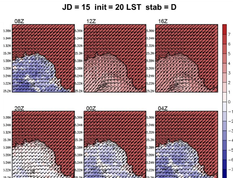
圖 5-68 A2Cflow 調校後之模擬(20m 高)風場，模擬日期太陽日為第 15 日，模擬初始時間為 20LST，中心位置為核一廠(第 4 層巢狀網格)，風向為 45^\circ ，風速為 8m/s，穩定度參數為 0.002(穩定度分類 D 級)，填色部分為溫度擾動，單位為 ^\circ\text{C} 。
