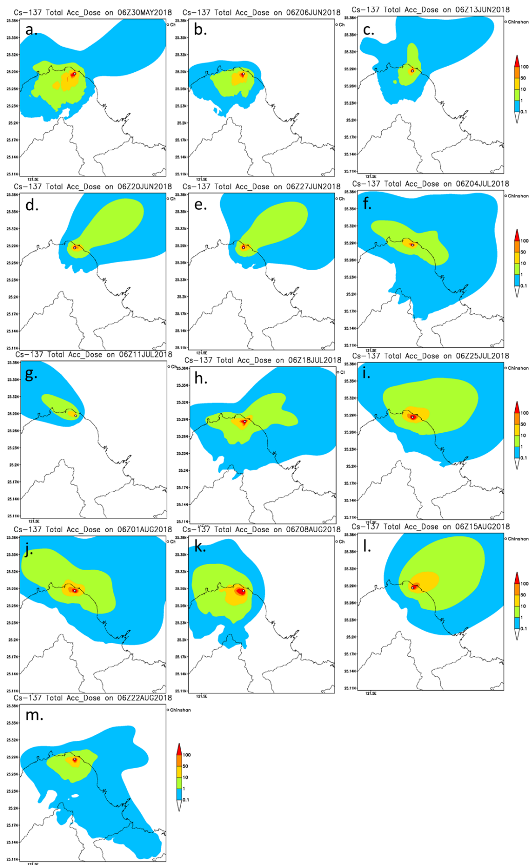
圖 4-19 核一廠夏季，自 2018 年 5 月 29 日至 2018 年 8 月 28 日 Cs-137 假想事故模擬之 7 日有效劑量累積圖(mSv)。
