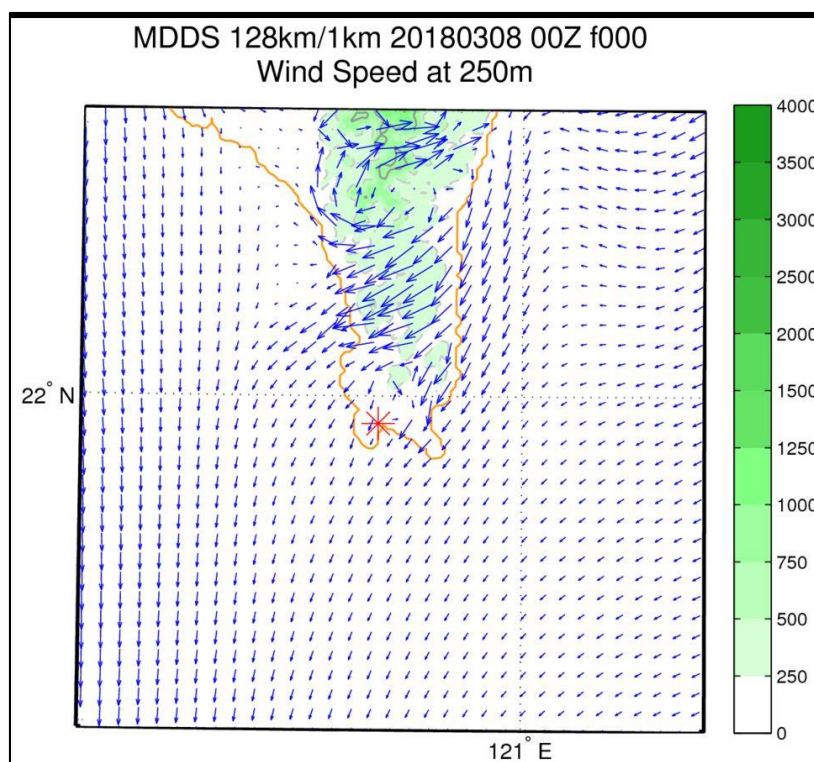
圖 3-20 MDDS 核三廠第一層巢狀網格(1 公里解析度)風場圖。東部海面的東風遇到屏東北部較高的中央山脈而轉向成北風系，直到南邊山勢較低轉為東北風過山，隨後在山後弱風速區產生依順時針渦旋(枋山東部山區)。
