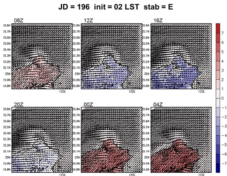
圖 5-86 A2Cflow 調校後之模擬(20m 高)風場，模擬日期太陽日為第 196 日，模擬初始時間為 20LST，中心位置為核一廠(第層巢狀網格)，風向為 45^\circ ，風速為 8m/s，穩定度參數為 0.005(穩定度分類 E 級)，填色部分為溫度擾動，單位為 ^\circ\text{C} 。
