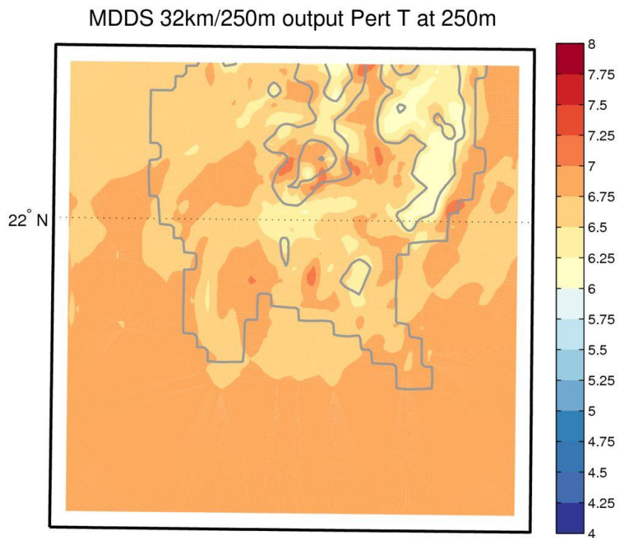
圖 3-29 MDDS 核三廠第三層巢狀網格(250 公尺解析度)溫度擾動場
