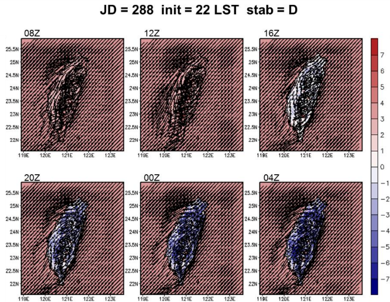
圖 5-57 A2Cflow 調校後之模擬(20m 高)風場，模擬日期太陽日為第 288 日，模擬初始時間為 22LST，中心位置為核一廠(第 1 層巢狀網格)，風向為 45^\circ ，風速為 5m/s，穩定度參數為 0.002(穩定度分類 D 級)，填色部分為溫度擾動，單位為 ^\circ\text{C} 。
