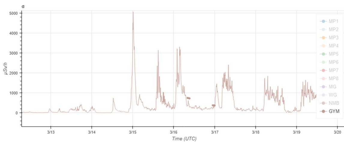
圖 7-8 福島電廠 GYM 測站劑量率模擬結果
