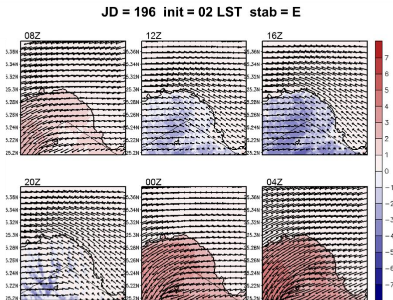
圖 5-56 A2Cflow 調校後之模擬(20m 高)風場，模擬日期太陽日為第 196 日，模擬初始時間為 02LST，中心位置為核一廠(第 4 層巢狀網格)，風向為 45^\circ ，風速為 5m/s，穩定度參數為 0.005(穩定度分類 E 級)，填色部分為溫度擾動，單位為 ^\circ\text{C} 。
