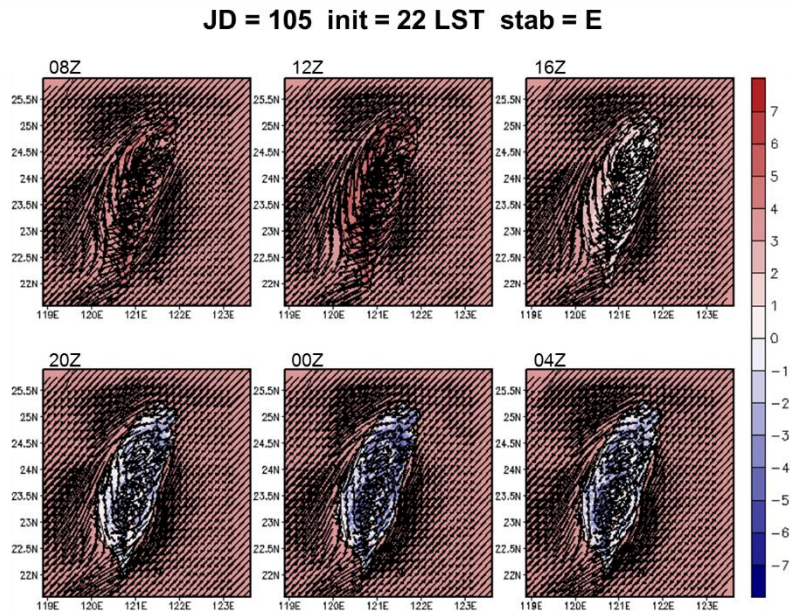
圖 5-45 A2Cflow 調校後之模擬(20m 高)風場，模擬日期太陽日為第 105 日，模擬初始時間為 22LST，中心位置為核一廠(第 1 層巢狀網格)，風向為 45^\circ ，風速為 5m/s，穩定度參數為 0.005(穩定度分類 E 級)，填色部分為溫度擾動，單位為 ^\circ\text{C} 。
