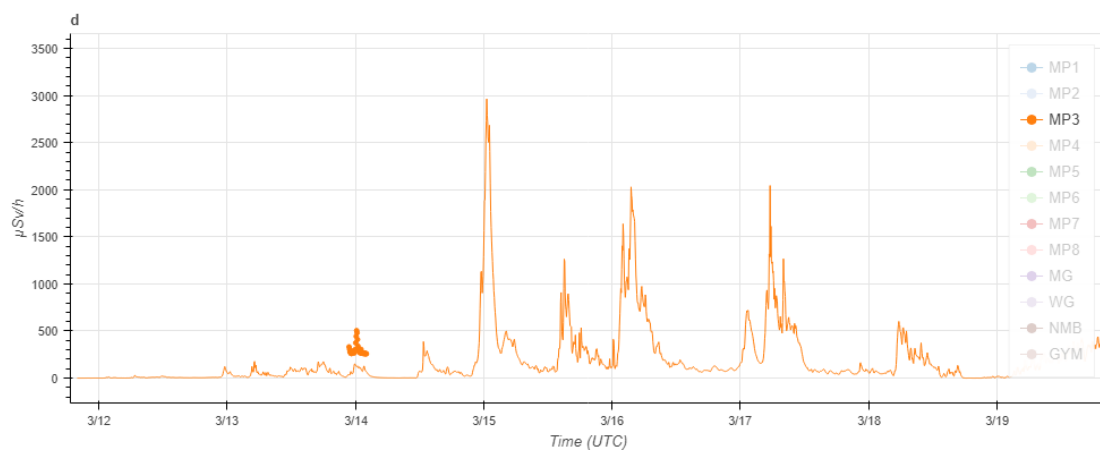
圖 7-12 福島電廠 MP3 測站劑量率模擬結果
