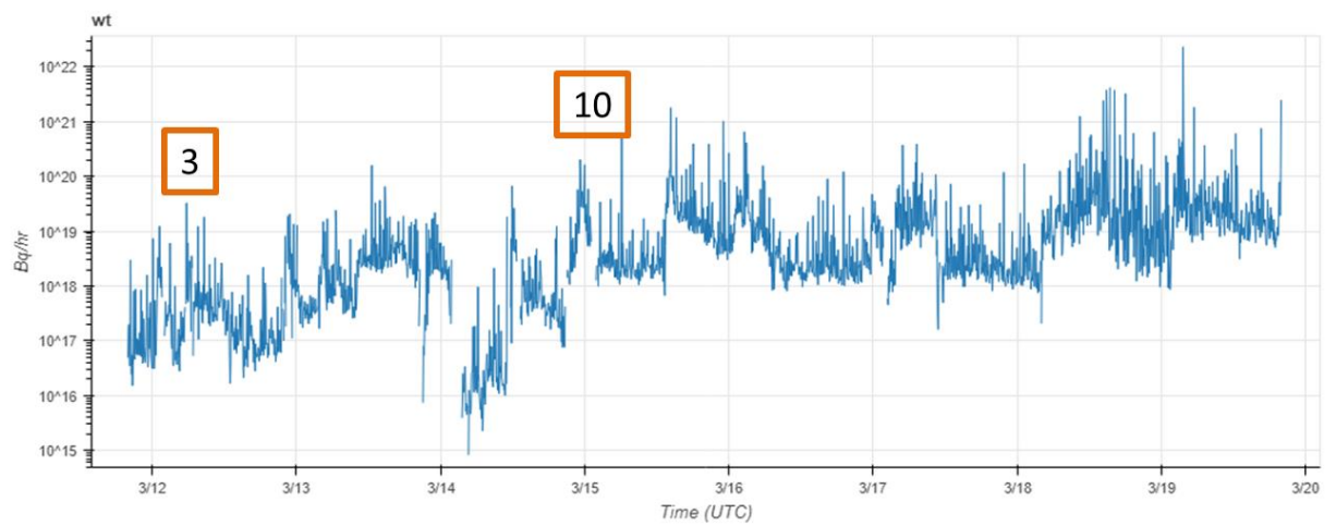
圖 7-4 福島事故射源項回推結果
