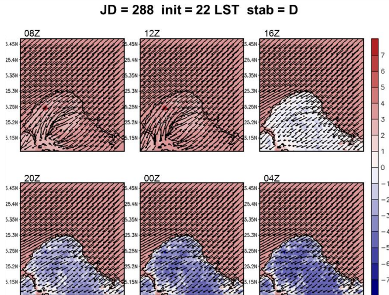
圖 5-59 A2Cflow 調校後之模擬(20m 高)風場，模擬日期太陽日為第 288 日，模擬初始時間為 22LST，中心位置為核一廠(第 3 層巢狀網格)，風向為 45^\circ ，風速為 5m/s，穩定度參數為 0.002(穩定度分類 D 級)，填色部分為溫度擾動，單位為 ^\circ\text{C} 。
