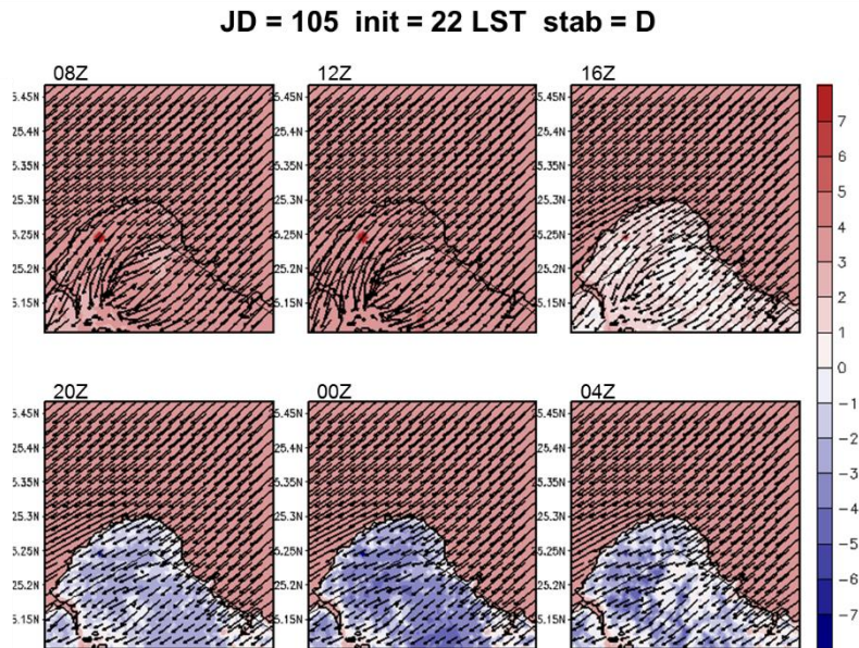
圖 5-43 A2Cflow 調校後之模擬(20m 高)風場，模擬日期太陽日為第 105 日，模擬初始時間為 22LST，中心位置為核一廠(第 3 層巢狀網格)，風向為 45^\circ ，風速為 5m/s，穩定度參數為 0.002(穩定度分類 D 級)，填色部分為溫度擾動，單位為 ^\circ\text{C} 。
