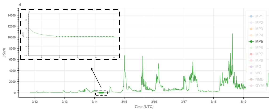
圖 7-14 福島電廠 MP5 測站劑量率模擬結果
