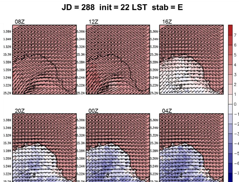
圖 5-64 A2Cflow 調校後之模擬(20m 高)風場，模擬日期太陽日為第 288 日，模擬初始時間為 22LST，中心位置為核一廠(第 4 層巢狀網格)，風向為 45^\circ ，風速為 5m/s，穩定度參數為 0.005(穩定度分類 E 級)，填色部分為溫度擾動，單位為 ^\circ\text{C} 。
