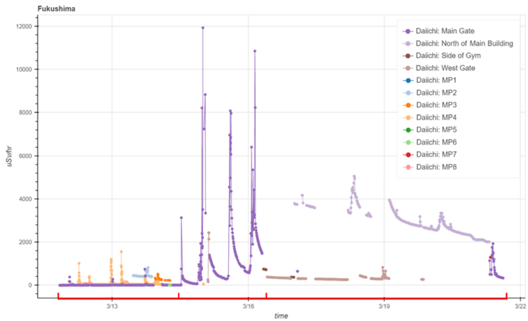
圖 7-3 福島電廠內 3 月 11 日至 21 日的輻射偵測值
