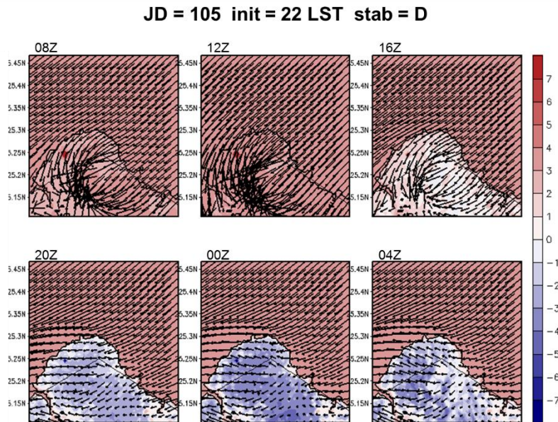
圖 5-11 A2Cflow 調校後之模擬(20m 高)風場，模擬日期太陽日為第 105 日，模擬初始時間為 22LST，中心位置為核一廠(第 3 層巢狀網格)，風向為 45^\circ ，風速為 2m/s，穩定度參數為 0.002(穩定度分類 D 級)；填色部分為溫度擾動，單位為 ^\circ\text{C} 。
