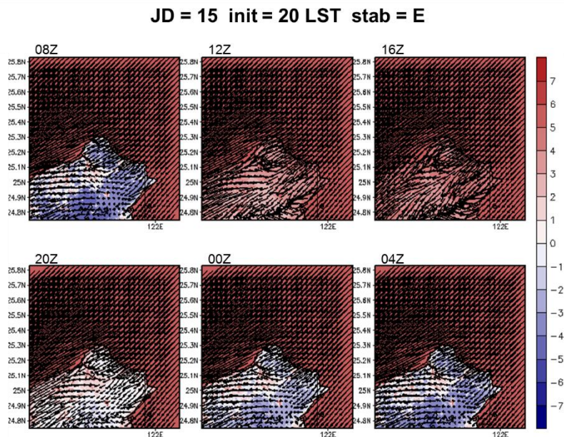
圖 5-38 A2Cflow 調校後之模擬(20m 高)風場，模擬日期太陽日為第 15 日，模擬初始時間為 20LST，中心位置為核一廠(第 2 層巢狀網格)，風向為 45^\circ ，風速為 5m/s，穩定度參數為 0.005(穩定度分類 E 級)，填色部分為溫度擾動，單位為 ^\circ\text{C} 。
