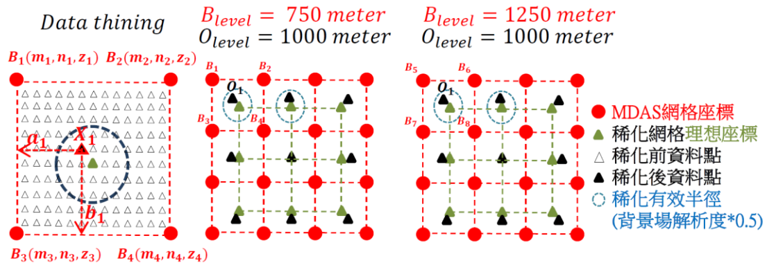
圖 6-4 觀測價值函數計算概念圖。圖中及圖右為稀化資料網格點設計示意圖，圖左為稀化方法示意圖。
