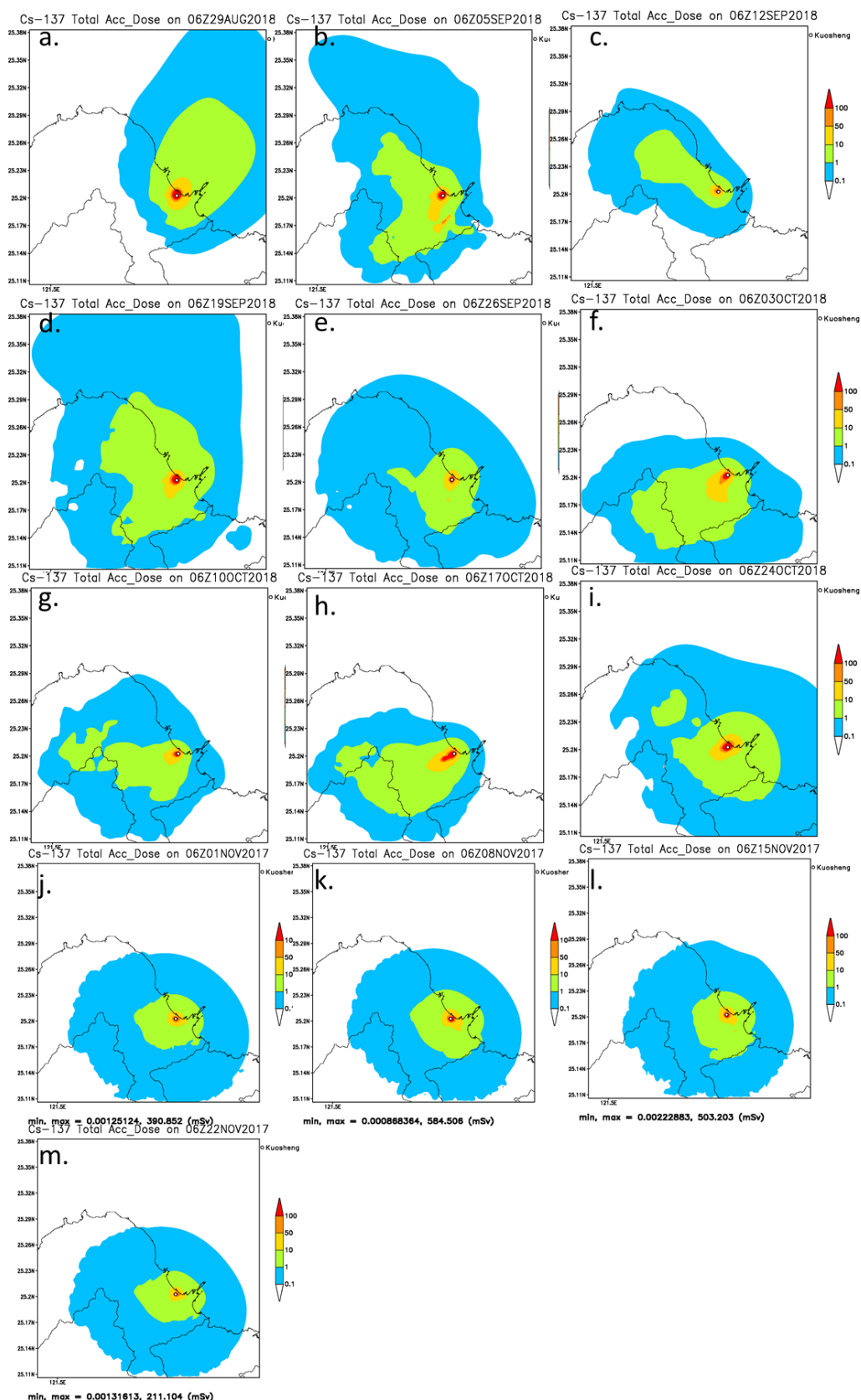
圖 4-27 核二廠秋季，自 2018 年 8 月 29 日至 2018 年 10 月 30 日和 2017 年 11 月 1 日至 11 月 29 日 Cs-137 假想事故模擬之 7 日有效劑量累積圖(mSv)。
