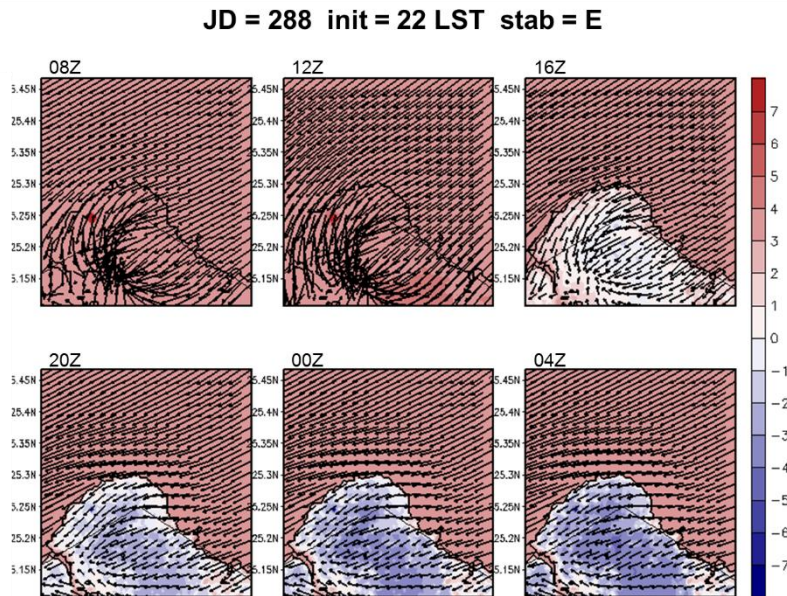
圖 5-31 A2Cflow 調校後之模擬(20m 高)風場，模擬日期太陽日為第 288 日，模擬初始時間為 22LST，中心位置為核一廠(第 3 層巢狀網格)，風向為 45^\circ ，風速為 2m/s，穩定度參數為 0.005(穩定度分類 E 級)，填色部分為溫度擾動，單位為 ^\circ\text{C} 。
