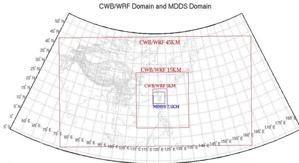
圖 2-9 CWB/WRF 不同解析度所包含的範圍及 MDDS 高解析度氣象資訊之範圍。紅色方框為 CWB/WRF，藍色方框為 MDDS 2.5 公里解析度範圍
