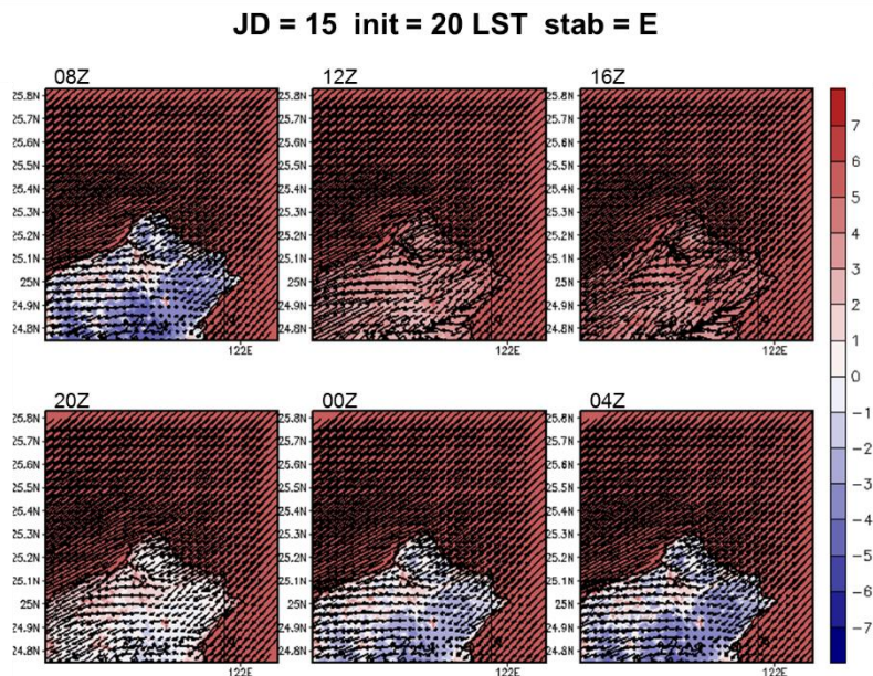
圖 5-70 A2Cflow 調校後之模擬(20m 高)風場，模擬日期太陽日為第 15 日，模擬初始時間為 20LST，中心位置為核一廠(第層巢狀網格)，風向為 45^\circ ，風速為 8m/s，穩定度參數為 0.005(穩定度分類 ED 級)，填色部分為溫度擾動，單位為 ^\circ\text{C} 。
