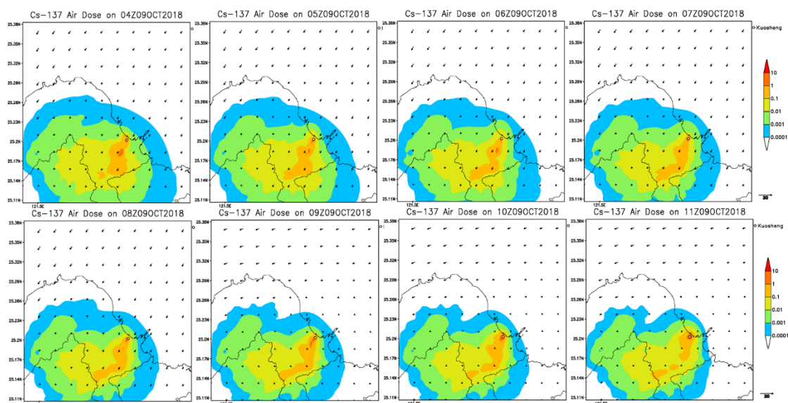
圖 4-31 2018 年 10 月 3 日當周，假想模擬中，Cs-137 劑量累積在大屯山的空氣劑量率(mSv/hr)及風場。
