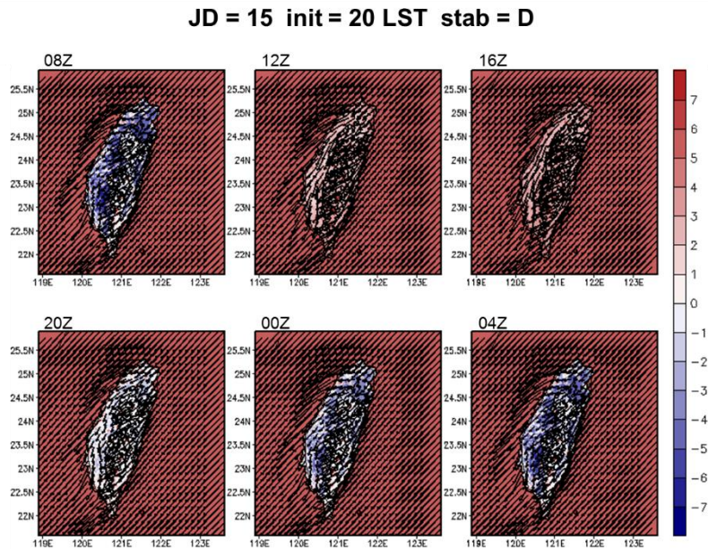
圖 5-65 A2Cflow 調校後之模擬(20m 高)風場，模擬日期太陽日為第 15 日，模擬初始時間為 20LST，中心位置為核一廠(第 1 層巢狀網格)，風向為 45^\circ ，風速為 8m/s，穩定度參數為 0.002(穩定度分類 D 級)，填色部分為溫度擾動，單位為 ^\circ\text{C} 。
