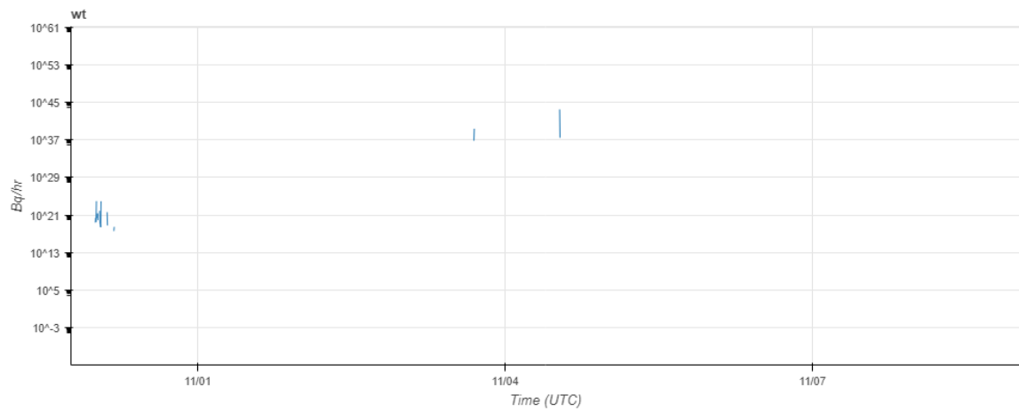
圖 7-20 核一廠尚未扣掉背景輻射值的射源項回推結果
