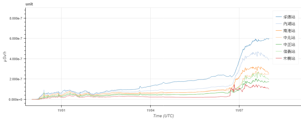
圖 7-19 單位釋放率在台北各測站的劑量表現
