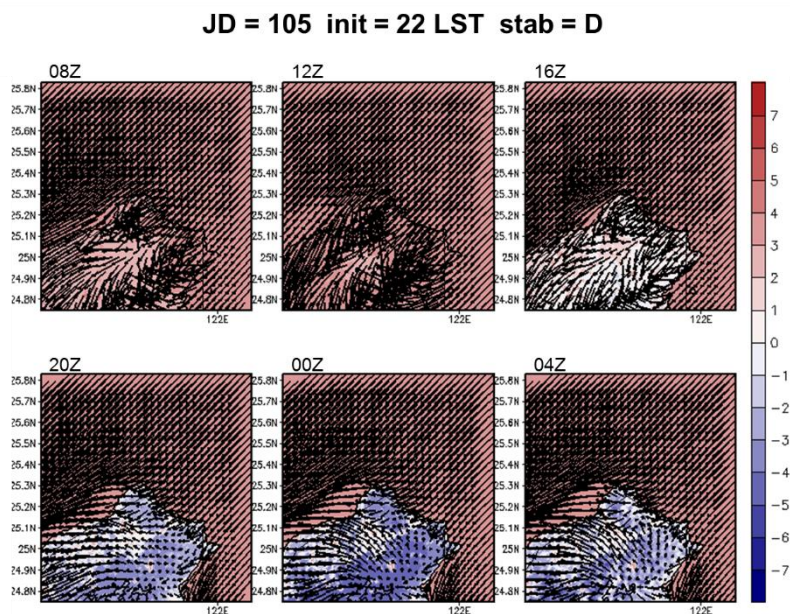
圖 5-10 A2Cflow 調校後之模擬(20m 高)風場，模擬日期太陽日為第 105 日，模擬初始時間為 22LST，中心位置為核一廠(第 2 層巢狀網格)，風向為 45^\circ ，風速為 2m/s，穩定度參數為 0.002(穩定度分類 D 級)；填色部分為溫度擾動，單位為 ^\circ\text{C} 。
