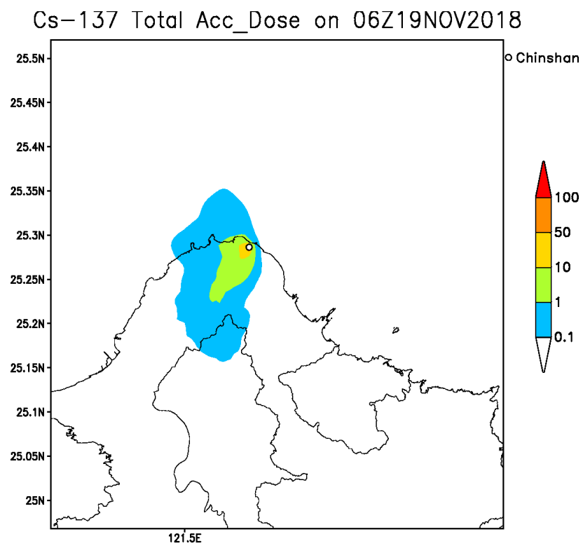
圖 7-25 核一廠 Cs-137 核種假想事故於 2018/11/19 七天有效劑量累積分布(mSv)
