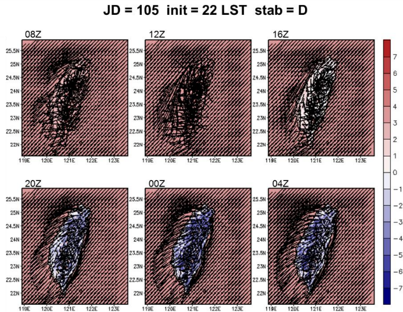
圖 5-9 A2Cflow 調校後之模擬(20m 高)風場，模擬日期太陽日為第 105 日，模擬初始時間為 22LST，中心位置為核一廠(第 1 層巢狀網格)，風向為 45^\circ ，風速為 2m/s，穩定度參數為 0.002(穩定度分類 D 級)；填色部分為溫度擾動，單位為 ^\circ\text{C} 。
