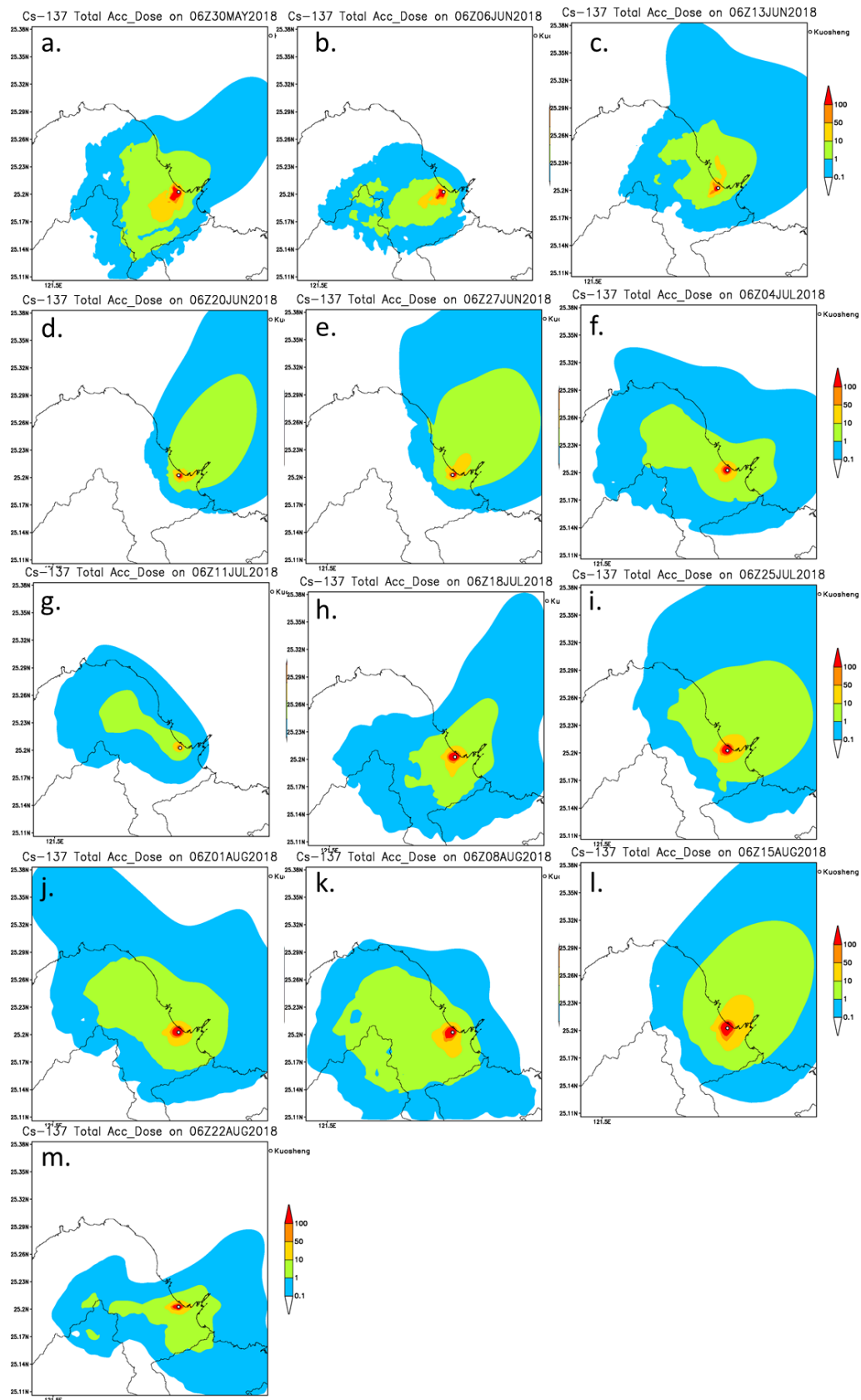
圖 4-21 核二廠夏季，自 2018 年 5 月 29 日至 2018 年 8 月 28 日 Cs-137 假想事故模擬之 7 日有效劑量累積圖(mSv)。
