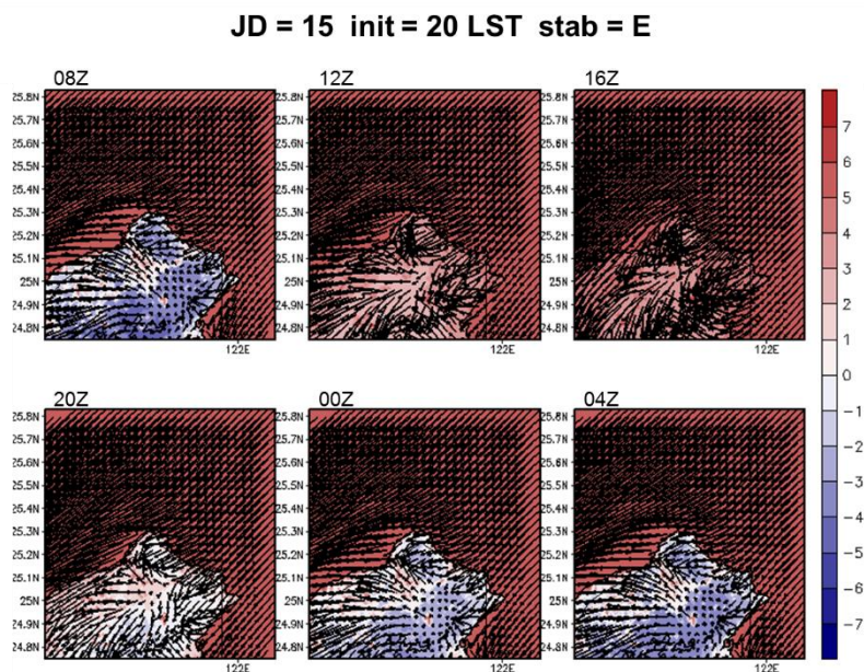
圖 5-6 A2Cflow 調校後之模擬(20m 高)風場，模擬日期太陽日為第 15 日，模擬初始時間為 20LST，中心位置為核一廠(第 2 層巢狀網格)，風向為 45^\circ ，風速為 2m/s，穩定度參數為 0.005(穩定度分類 E 級)；填色部分為溫度擾動，單位為 ^\circ\text{C} 。
