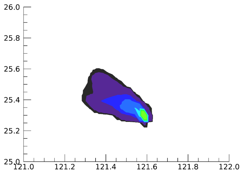
圖 3-5 核一廠案例不同劑量網格設定輸出結果 3
