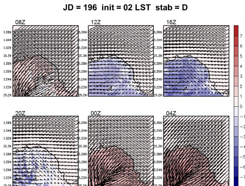
圖 5-20 A2Cflow 調校後之模擬(20m 高)風場，模擬日期太陽日為第 196 日，模擬初始時間為 02LST，中心位置為核一廠(第 4 層巢狀網格)，風向為 45^\circ ，風速為 2m/s，穩定度參數為 0.002(穩定度分類 D 級)；填色部分為溫度擾動，單位為 ^\circ\text{C} 。
