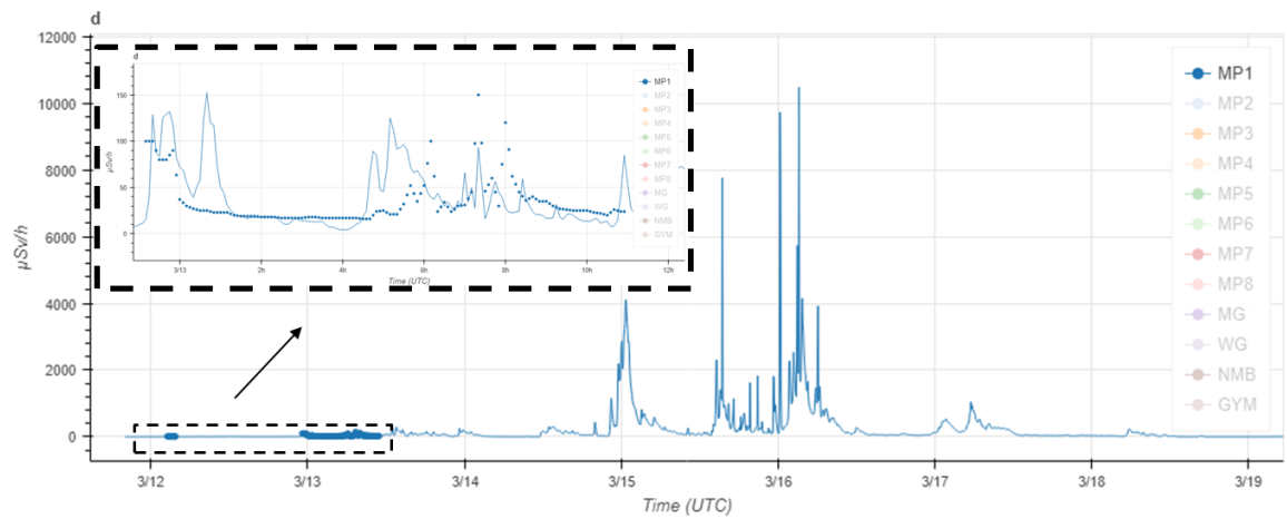
圖 7-10 福島電廠 MP1 測站劑量率模擬結果
