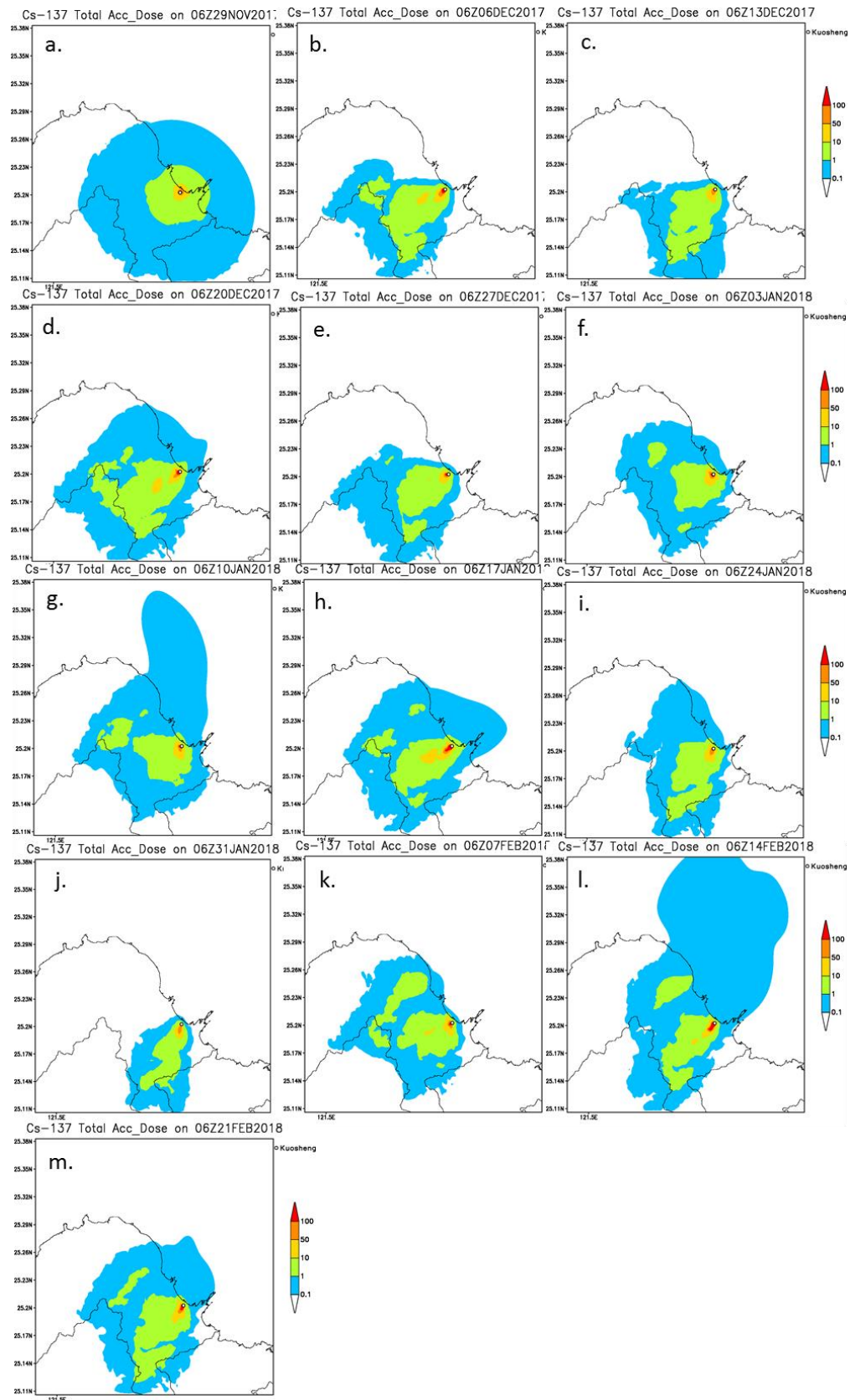
圖 4-4 核二廠冬季，自 2017 年 11 月 29 日至 2018 年 2 月 27 日 Cs-137 假想事故模擬之 7 日有效劑量累積圖(mSv)。
