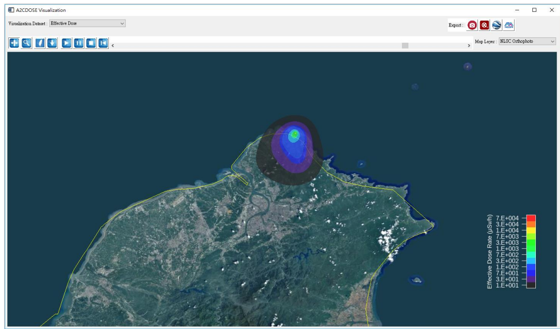
圖 3-10 核一廠案例有效劑量率分布顯示
