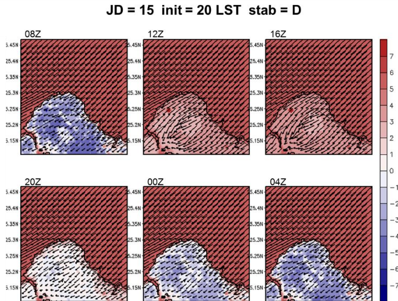
圖 5-67 A2Cflow 調校後之模擬(20m 高)風場，模擬日期太陽日為第 15 日，模擬初始時間為 20LST，中心位置為核一廠(第 3 層巢狀網格)，風向為 45^\circ ，風速為 8m/s，穩定度參數為 0.002(穩定度分類 D 級)，填色部分為溫度擾動，單位為 ^\circ\text{C} 。
