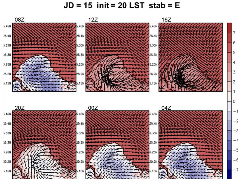
圖 5-7 A2Cflow 調校後之模擬(20m 高)風場，模擬日期太陽日為第 15 日，模擬初始時間為 20LST，中心位置為核一廠(第 3 層巢狀網格)，風向為 45^\circ ，風速為 2m/s，穩定度參數為 0.005(穩定度分類 E 級)；填色部分為溫度擾動，單位為 ^\circ\text{C} 。
