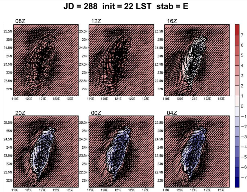
圖 5-29 A2Cflow 調校後之模擬(20m 高)風場，模擬日期太陽日為第 288 日，模擬初始時間為 22LST，中心位置為核一廠(第 1 層巢狀網格)，風向為 45^\circ ，風速為 2m/s，穩定度參數為 0.005(穩定度分類 E 級)，填色部分為溫度擾動，單位為 ^\circ\text{C} 。
