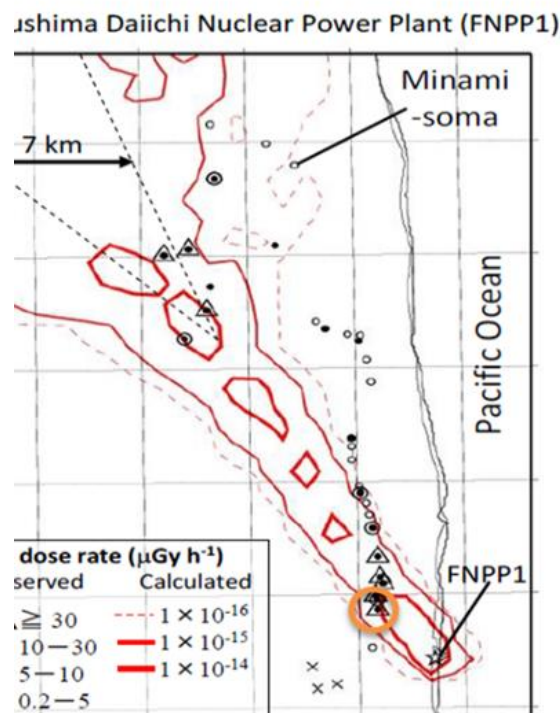
圖 2-11 福島事故觀測資料點與劑量模擬計算結果
