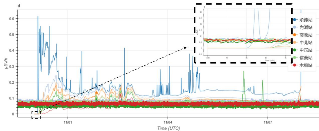
圖 7-21 核一廠在台北測站扣掉背景範圍值後劑量率模擬結果
