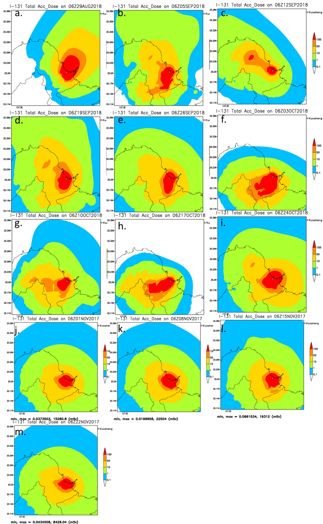
圖 4-28 核二廠秋季，自 2018 年 8 月 29 日至 2018 年 10 月 30 日和 2017 年 11 月 1 日至 11 月 29 日 I-131 假想事故模擬之 7 日有效劑量累積圖(mSv)。
