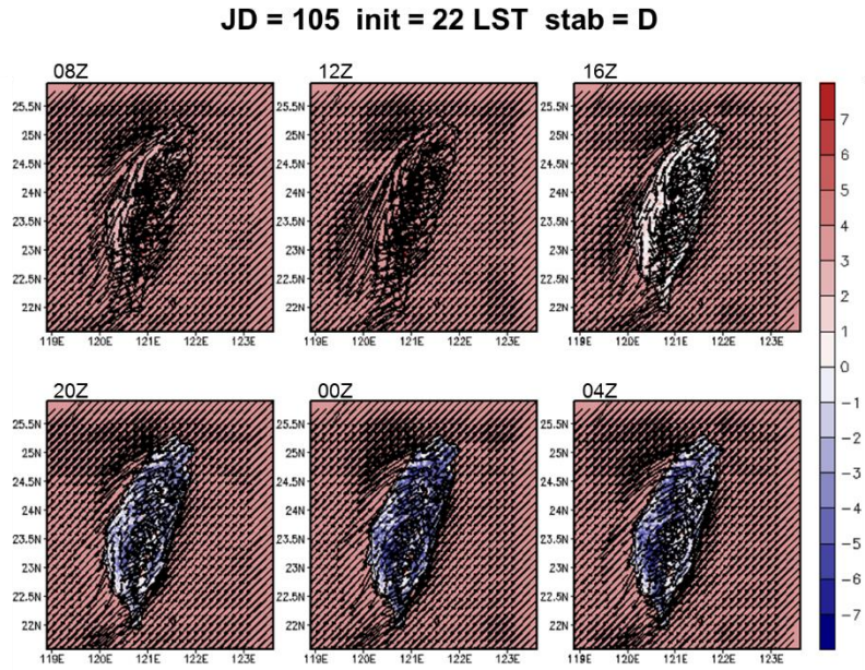
圖 5-41 A2Cflow 調校後之模擬(20m 高)風場，模擬日期太陽日為第 105 日，模擬初始時間為 22LST，中心位置為核一廠(第 1 層巢狀網格)，風向為 45^\circ ，風速為 5m/s，穩定度參數為 0.002(穩定度分類 D 級)，填色部分為溫度擾動，單位為 ^\circ\text{C} 。
