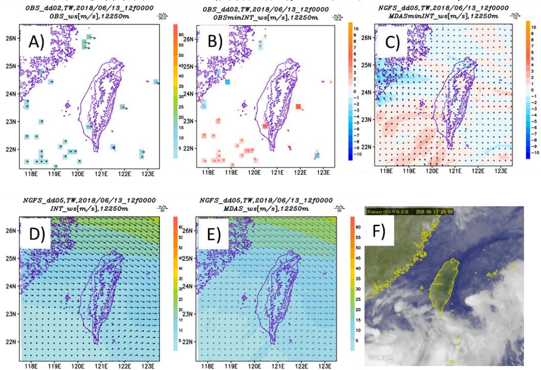
圖 6-8 2018 西南季風(06/13)12250 公尺風速。(A)傳統高空觀測資料、(B)觀測資料減初始猜測場、(C)MDAS 減初始猜測場、(D)初始猜測場、(E)MDAS 與(F)衛星雲圖；(A)(D)(E)風標為向量，(B)(C)風標為向量差。
