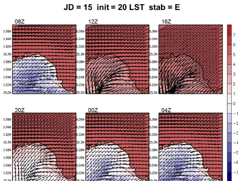
圖 5-8 A2Cflow 調校後之模擬(20m 高)風場，模擬日期太陽日為第 15 日，模擬初始時間為 20LST，中心位置為核一廠(第 4 層巢狀網格)，風向為 45^\circ ，風速為 2m/s，穩定度參數為 0.005(穩定度分類 E 級)；填色部分為溫度擾動，單位為 ^\circ\text{C} 。
