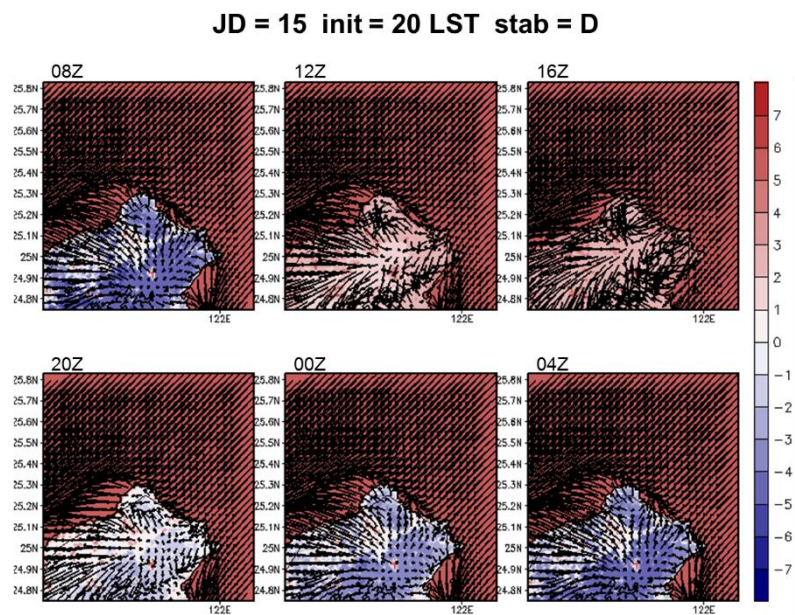
圖 5-2 A2Cflow 調校後之模擬(20m 高)風場，模擬日期太陽日為第 15 日，模擬初始時間為 20LST，中心位置為核一廠(第 2 層巢狀網格)，風向為 45^\circ ，風速為 2m/s，穩定度參數為 0.002(穩定度分類 D 級)；填色部分為溫度擾動，單位為 ^\circ\text{C} 。
