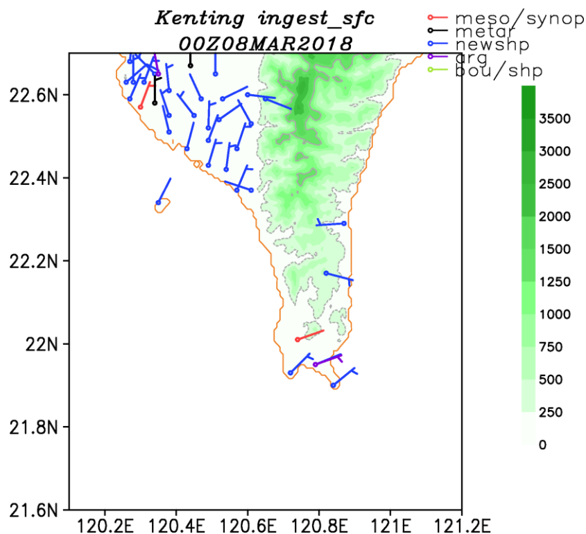
圖 3-23 2018/03/08 氣象局自動氣象站(藍色風標)、氣象局局屬測站(紅色風標)及機場站(黑色風標)測站風向圖。測站觀測結果和 MDDS 解析結果差不多，東部為東北風，西部為西北風，墾丁一帶為東北風系。
