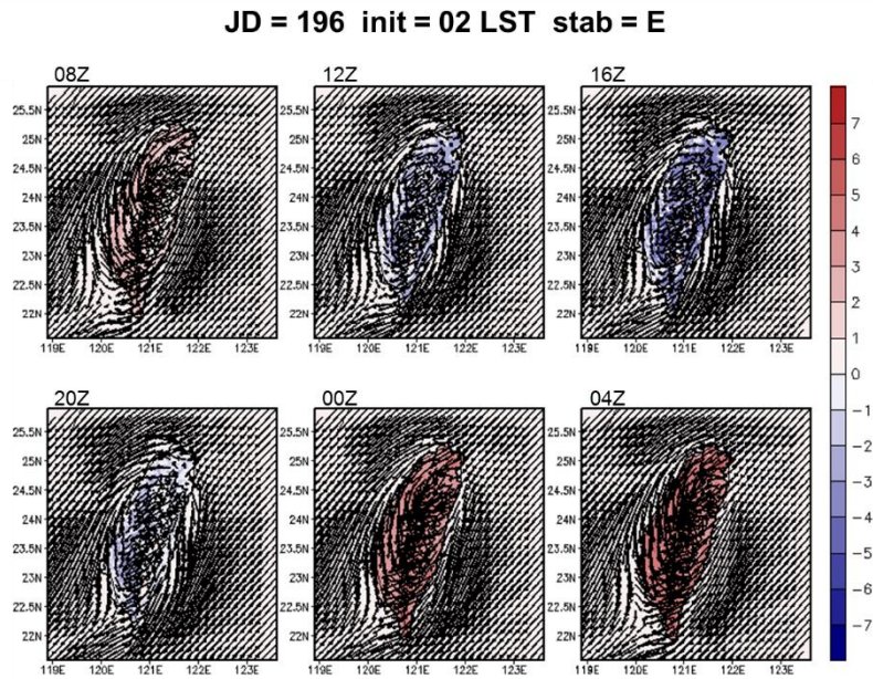
圖 5-53 A2Cflow 調校後之模擬(20m 高)風場，模擬日期太陽日為第 196 日，模擬初始時間為 02LST，中心位置為核一廠(第 1 層巢狀網格)，風向為 45^\circ ，風速為 5m/s，穩定度參數為 0.005(穩定度分類 E 級)，填色部分為溫度擾動，單位為 ^\circ\text{C} 。
