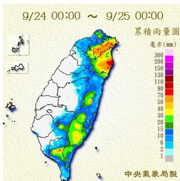
圖 3-30 2018 年 9 月 24 日 24 小時降雨累積圖(圖片來源:中央氣象局官網)
