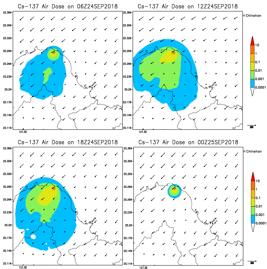
圖 3-34 2018 年 9 月 24 日包含濕沉降過程之每六小時之空氣劑量率 (mSv/hr) 分布。
