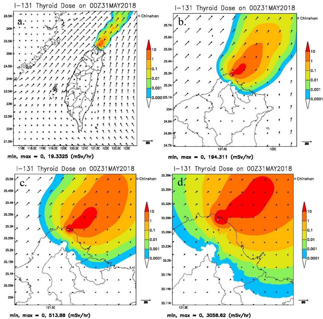
圖 3-17 核一廠 4 層巢狀網格之劑量評估系統結果，圖為 2018/05/30 I-131 的假想案例模擬，預報 24 小時後(2018/05/31)的甲狀腺約定等價劑量分布，單位:mSv/hr。由左至右，由上至下依序為 a. 解析度 2.5 公里 b.解析度 1 公里 c.解析度 500 公尺 d.解析度 250 公尺。
