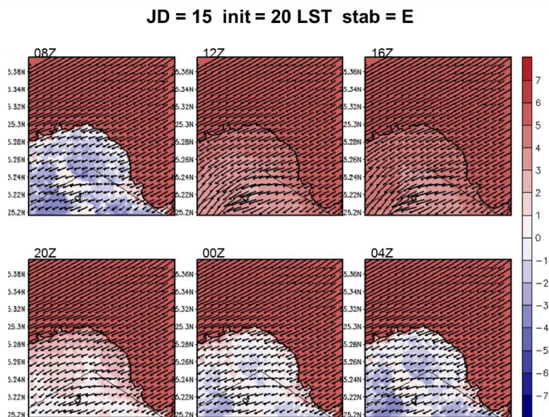
圖 5-72 A2Cflow 調校後之模擬(20m 高)風場，模擬日期太陽日為第 15 日，模擬初始時間為 20LST，中心位置為核一廠(第 4 層巢狀網格)，風向為 45^\circ ，風速為 8m/s，穩定度參數為 0.005(穩定度分類 E 級)，填色部分為溫度擾動，單位為 ^\circ\text{C} 。
