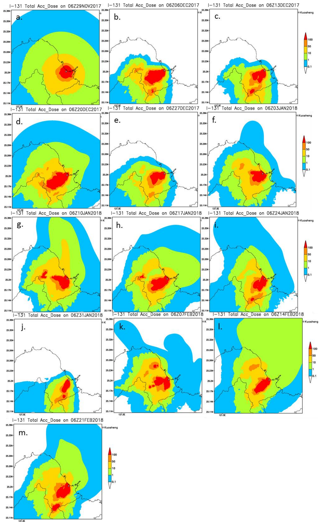
圖 4-5 核二廠冬季，自 2017 年 11 月 29 日至 2018 年 2 月 27 日 I-131 假想事故模擬之 7 日有效劑量累積圖(mSv)。
