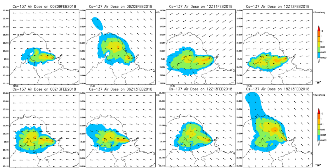
圖 4-8 2018 年 2 月 7 日當周，Cs-137 假想模擬中，劑量累積在大屯山的空氣劑量率及風場。
