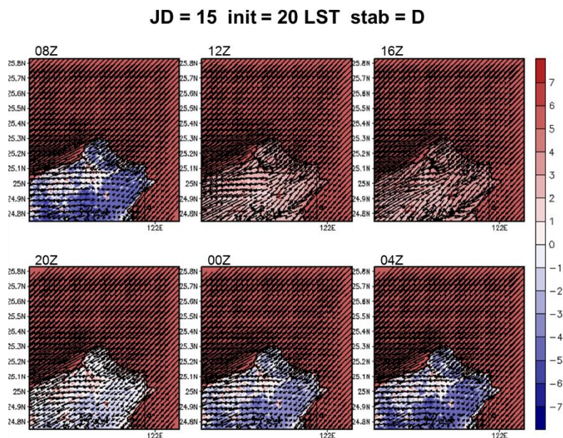
圖 5-66 A2Cflow 調校後之模擬(20m 高)風場，模擬日期太陽日為第 15 日，模擬初始時間為 20LST，中心位置為核一廠(第 2 層巢狀網格)，風向為 45^\circ ，風速為 8m/s，穩定度參數為 0.002(穩定度分類 D 級)，填色部分為溫度擾動，單位為 ^\circ\text{C} 。
