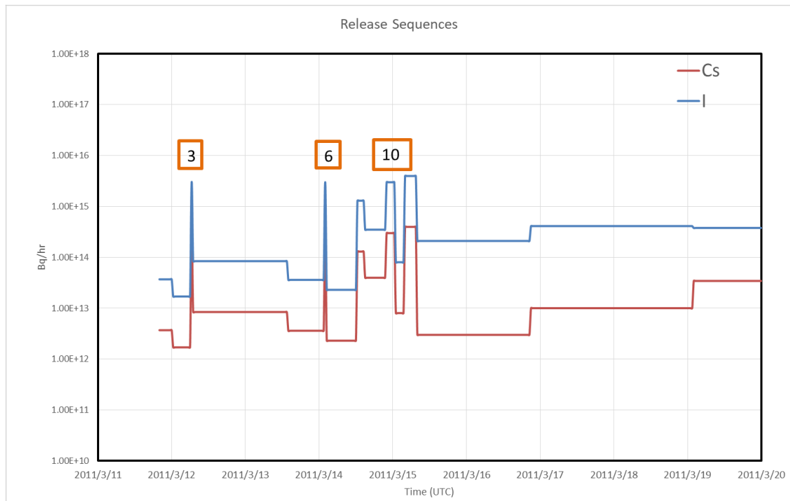
圖 7-5 JAEA 的 I-131 與 Cs-137 的回推研究結果
