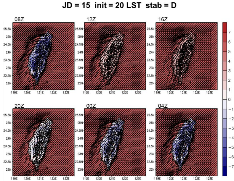
圖 5-33 A2Cflow 調校後之模擬(20m 高)風場，模擬日期太陽日為第 15 日，模擬初始時間為 20LST，中心位置為核一廠(第 1 層巢狀網格)，風向為 45^\circ ，風速為 5m/s，穩定度參數為 0.002(穩定度分類 D 級)，填色部分為溫度擾動，單位為 ^\circ\text{C} 。
