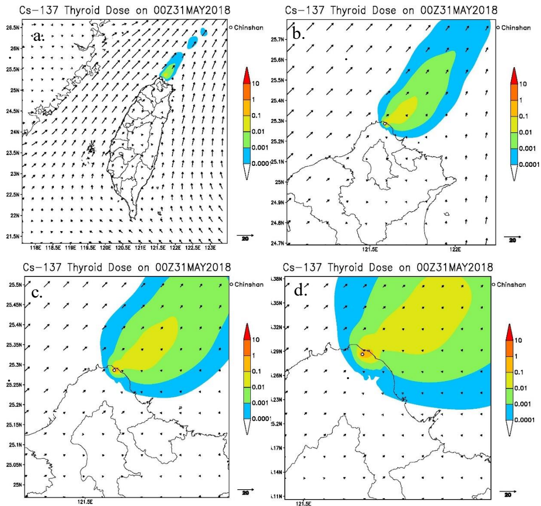
圖 3-14 核一廠 4 層巢狀網格之劑量評估系統結果，圖為 2018/05/30 Cs-137 的假想案例模擬，預報 24 小時後(2018/05/31)的甲狀腺約定等價劑量分布，單位:mSv/hr。由左至右，由上至下依序為 a. 解析度 2.5 公里 b.解析度 1 公里 c.解析度 500 公尺 d.解析度 250 公尺。
