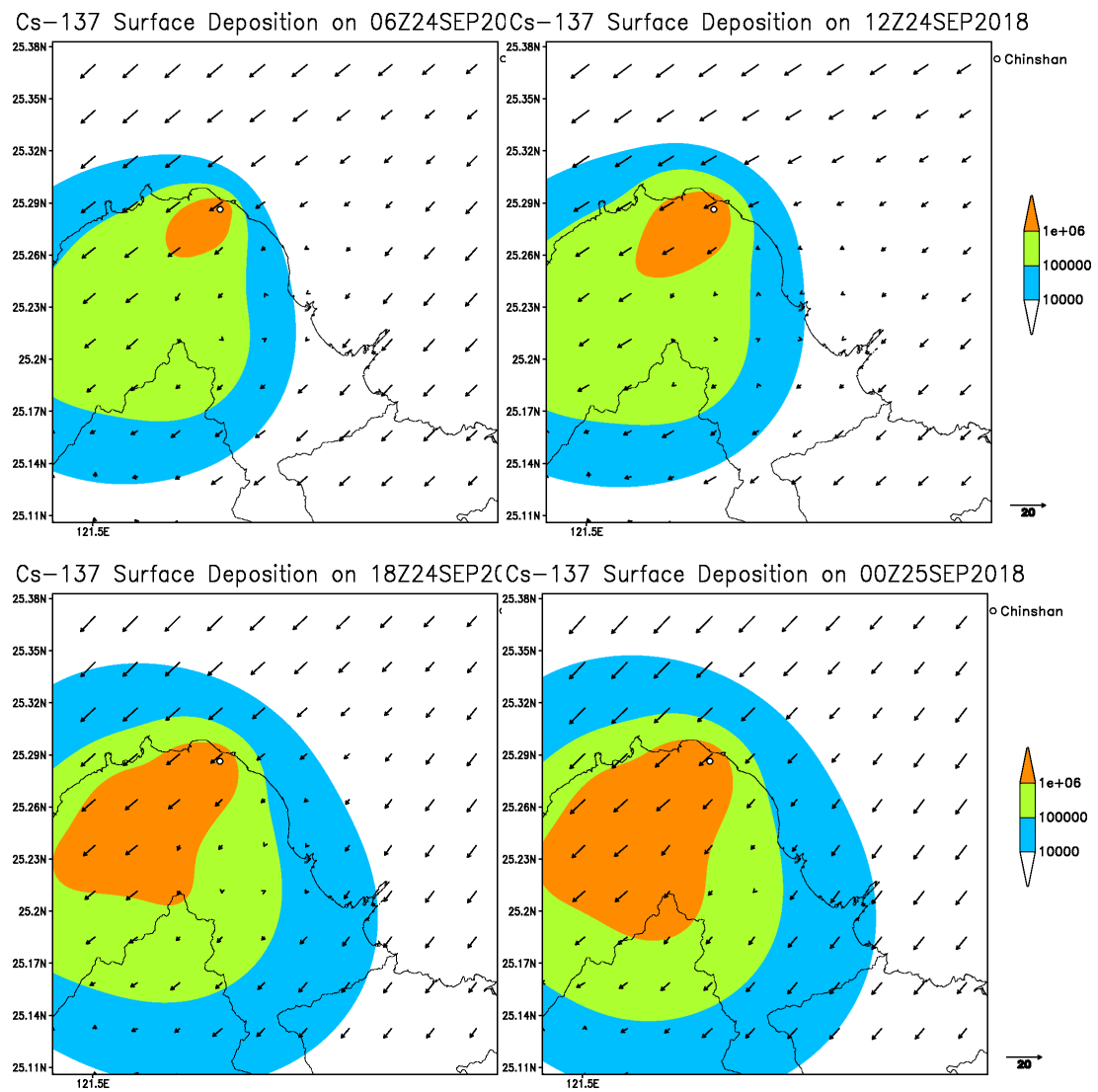
圖 3-35 2018 年 9 月 24 日包含濕沉降過程之每六小時之地表沉降累積量( \text{Bq}/\text{m}^2 )分布。
