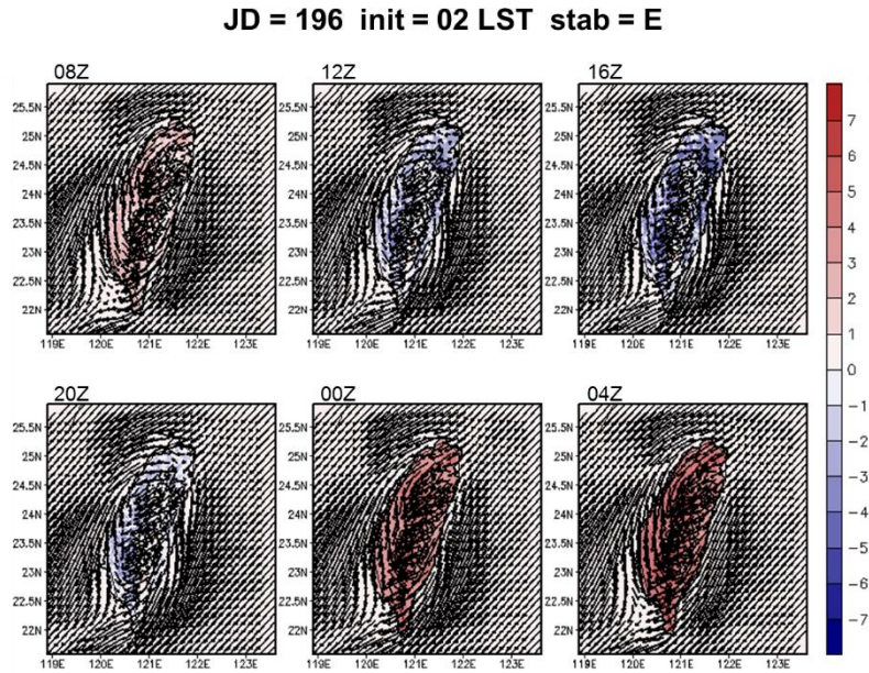
圖 5-85 A2Cflow 調校後之模擬(20m 高)風場，模擬日期太陽日為第 196 日，模擬初始時間為 20LST，中心位置為核一廠(第 1 層巢狀網格)，風向為 45^\circ ，風速為 8m/s，穩定度參數為 0.005(穩定度分類 E 級)，填色部分為溫度擾動，單位為 ^\circ\text{C} 。
