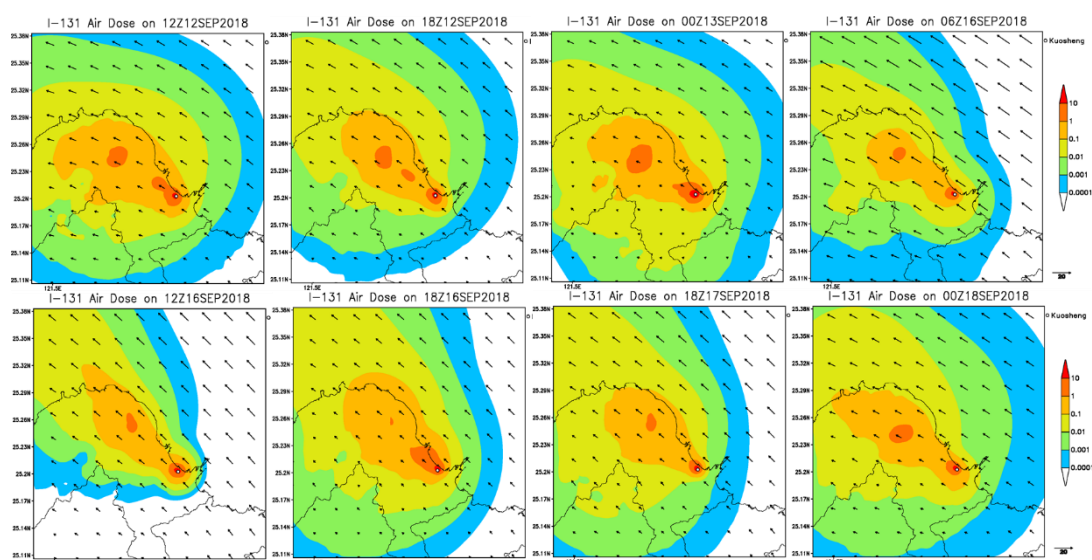
圖 4-30 2018 年 9 月 12 日當周，假想模擬中，I-131 劑量累積在金山地區的空 氣劑量率(mSv/hr)及風場。
