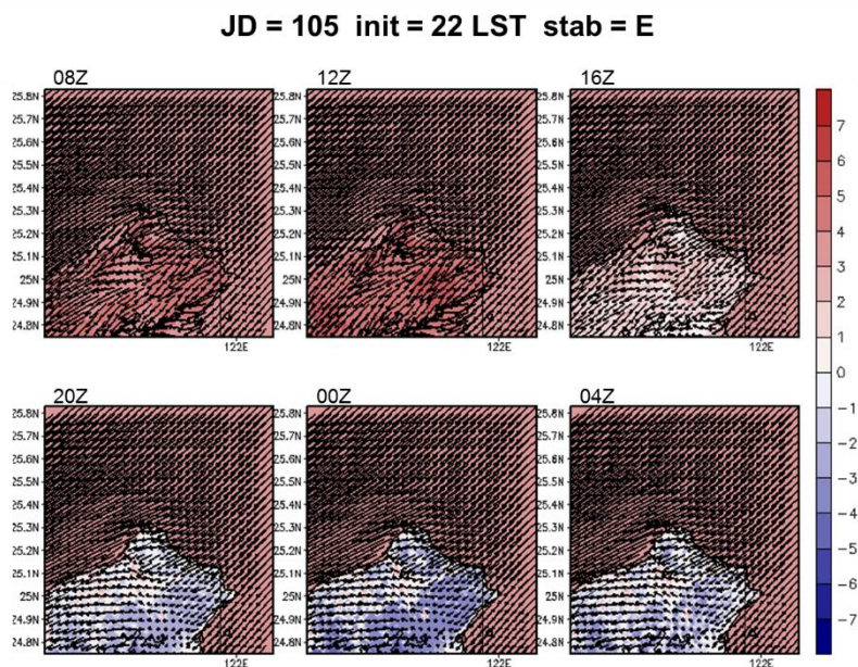
圖 5-78 A2Cflow 調校後之模擬(20m 高)風場，模擬日期太陽日為第 105 日，模擬初始時間為 20LST，中心位置為核一廠(第層巢狀網格)，風向為 45^\circ ，風速為 8m/s，穩定度參數為 0.005(穩定度分類 ED 級)，填色部分為溫度擾動，單位為 ^\circ\text{C} 。
