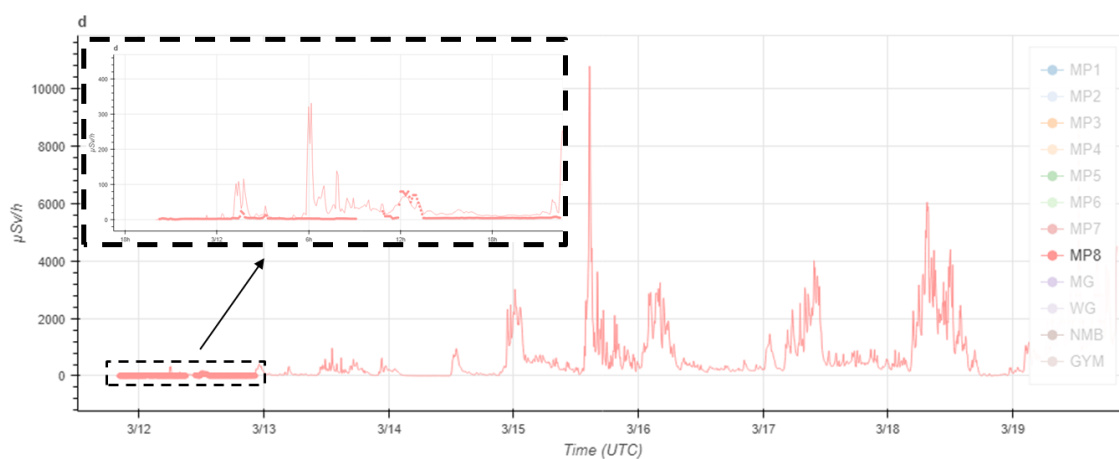
圖 7-17 福島電廠 MP8 測站劑量率模擬結果
