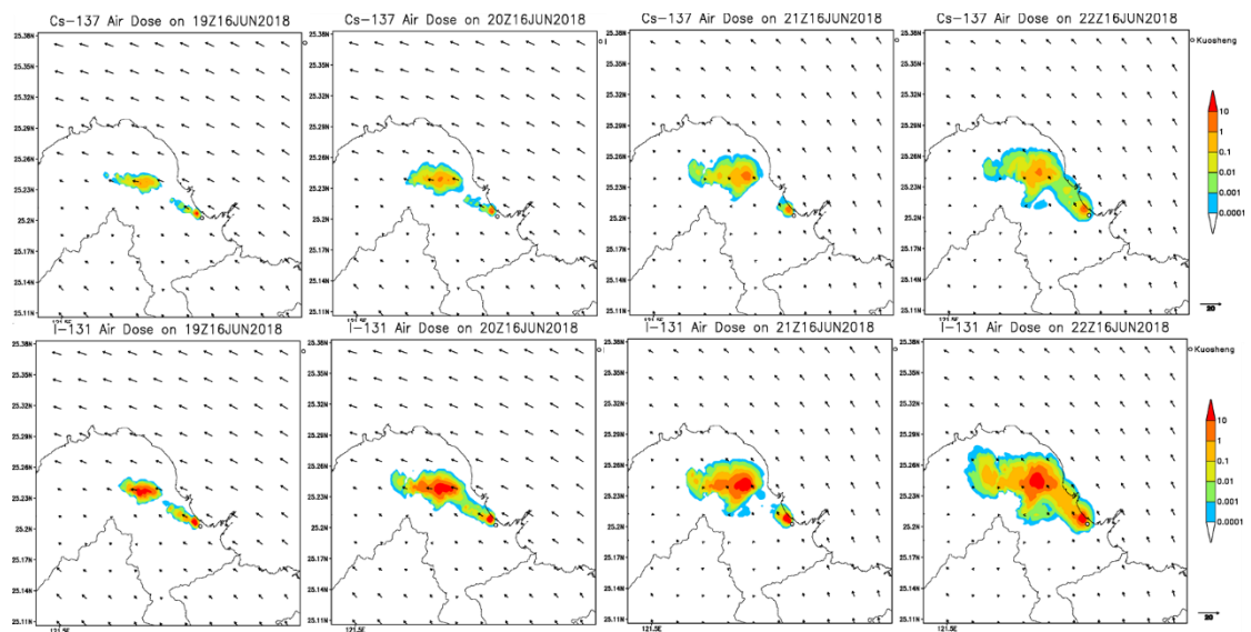
圖 4-24 2018 年 6 月 13 日當周，假想模擬中，劑量累積在大屯山的空氣劑量率及風場。上半部:Cs-137，下半部:I-131
