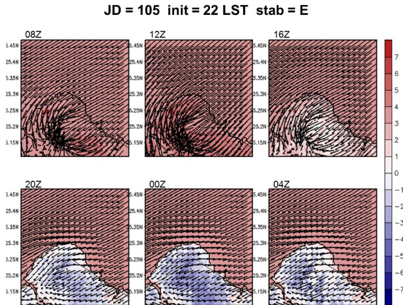
圖 5-15 A2Cflow 調校後之模擬(20m 高)風場，模擬日期太陽日為第 105 日，模擬初始時間為 22LST，中心位置為核一廠(第 3 層巢狀網格)，風向為 45^\circ ，風速為 2m/s，穩定度參數為 0.005(穩定度分類 E 級)；填色部分為溫度擾動，單位為 ^\circ\text{C} 。
