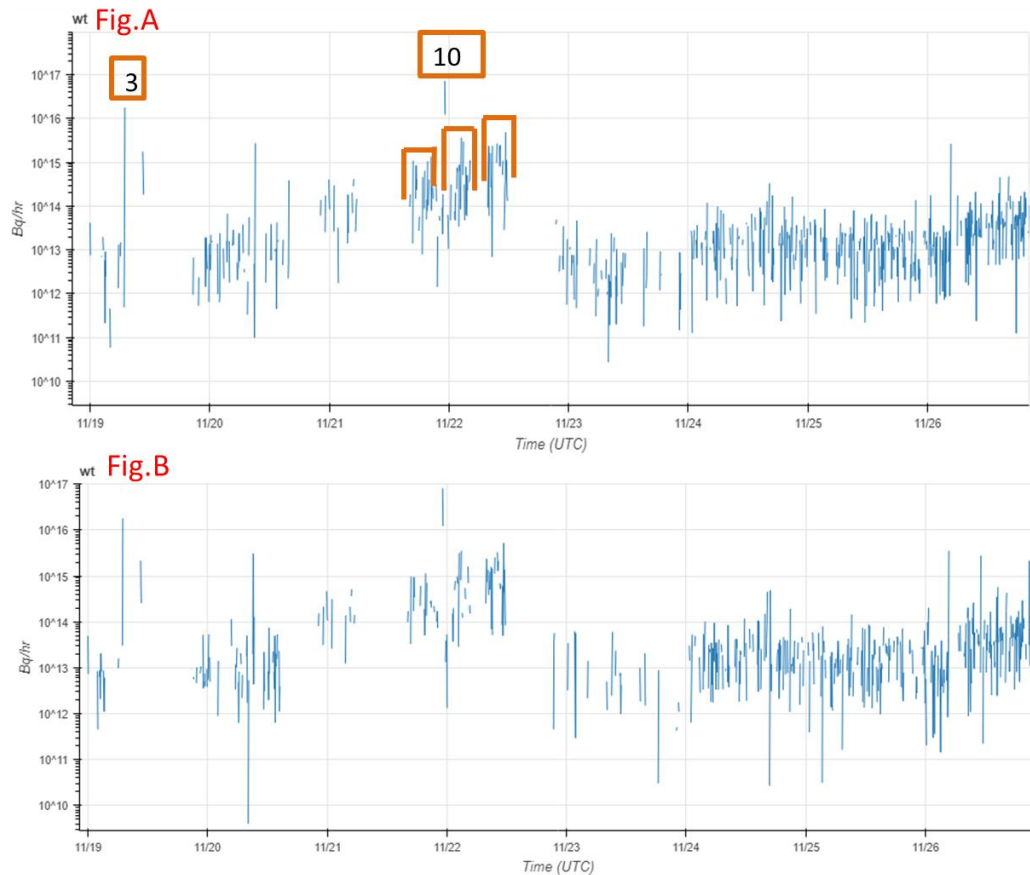
圖 7-28 Fig.A 為福島事件外釋於核二廠後，用臺灣測站回推釋放率結果，FigB 為將觀測資料加減 10% 的誤差值後，計算回推後結果比較。
