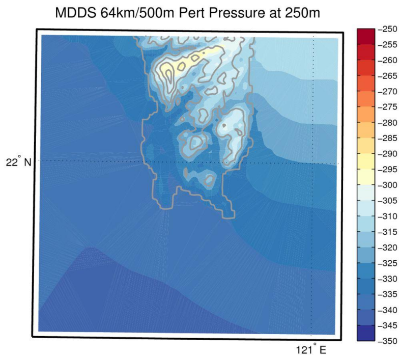
圖 3-25 MDDS 核三廠第二層巢狀網格(500 公尺解析度)壓力擾動場
