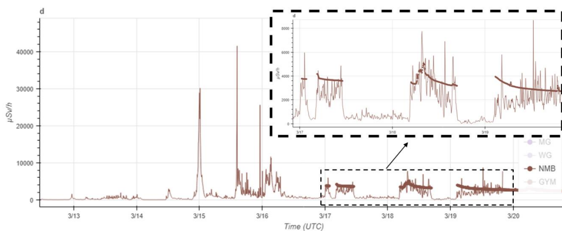
圖 7-7 福島電廠 NMB 測站劑量率模擬結果
