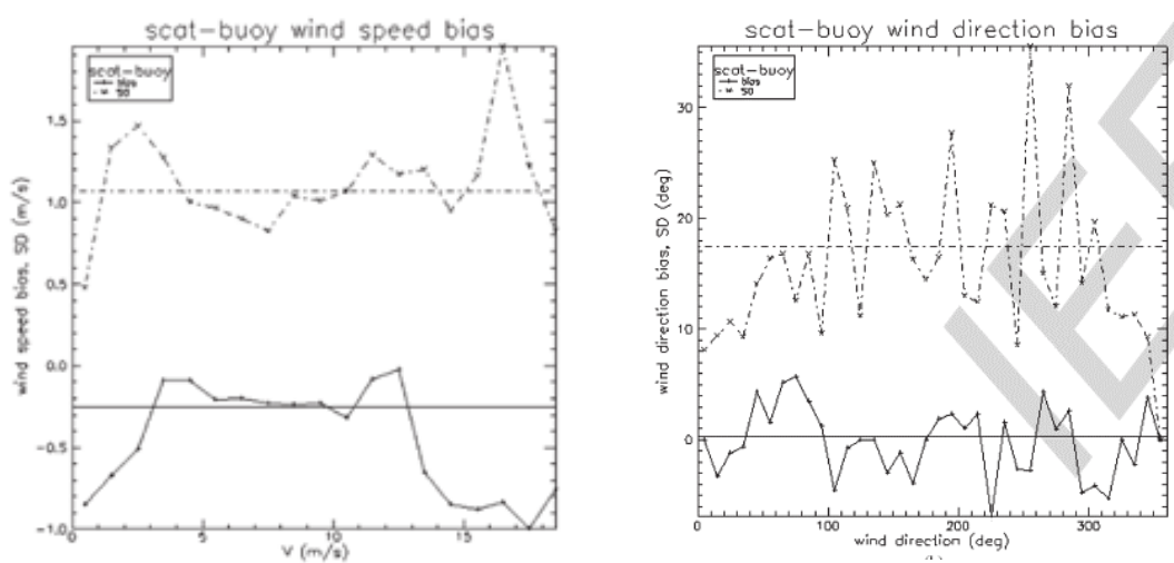
圖 6-1 ASCAT 與浮標之偏差量與標準差，顯示當環境風速為 3~13 m/s 時 bias 最小，反演風場與觀測相近。左圖為風速 m/s，右圖為風向 degree(實線為 Bias，虛線為 Standard Deviation)。摘自 Verspeek et al.(2009)
