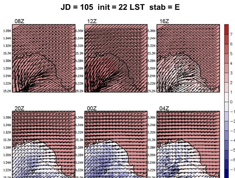
圖 5-16 A2Cflow 調校後之模擬(20m 高)風場，模擬日期太陽日為第 105 日，模擬初始時間為 22LST，中心位置為核一廠(第 4 層巢狀網格)，風向為 45^\circ ，風速為 2m/s，穩定度參數為 0.005(穩定度分類 E 級)；填色部分為溫度擾動，單位為 ^\circ\text{C} 。
