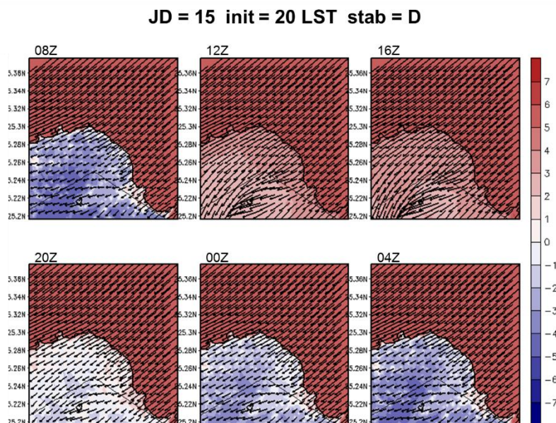
圖 5-36 A2Cflow 調校後之模擬(20m 高)風場，模擬日期太陽日為第 15 日，模擬初始時間為 20LST，中心位置為核一廠(第 4 層巢狀網格)，風向為 45^\circ ，風速為 5m/s，穩定度參數為 0.002(穩定度分類 D 級)，填色部分為溫度擾動，單位為 ^\circ\text{C} 。
