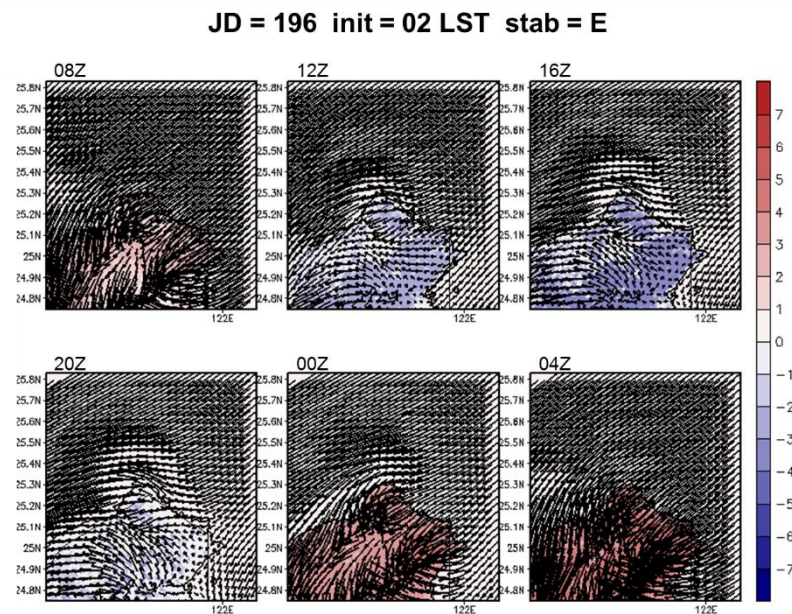
圖 5-22 A2Cflow 調校後之模擬(20m 高)風場，模擬日期太陽日為第 196 日，模擬初始時間為 02LST，中心位置為核一廠(第 2 層巢狀網格)，風向為 45^\circ ，風速為 2m/s，穩定度參數為 0.005(穩定度分類 E 級)，填色部分為溫度擾動，單位為 ^\circ\text{C} 。
