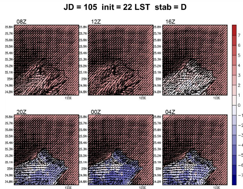
圖 5-42 A2Cflow 調校後之模擬(20m 高)風場，模擬日期太陽日為第 105 日，模擬初始時間為 22LST，中心位置為核一廠(第 2 層巢狀網格)，風向為 45^\circ ，風速為 5m/s，穩定度參數為 0.002(穩定度分類 D 級)，填色部分為溫度擾動，單位為 ^\circ\text{C} 。
