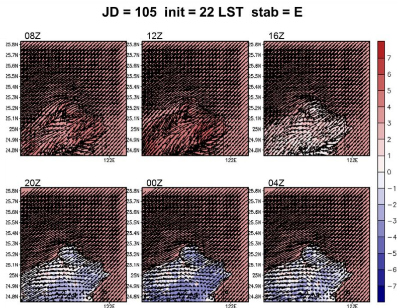
圖 5-46 A2Cflow 調校後之模擬(20m 高)風場，模擬日期太陽日為第 105 日，模擬初始時間為 22LST，中心位置為核一廠(第 2 層巢狀網格)，風向為 45^\circ ，風速為 5m/s，穩定度參數為 0.005(穩定度分類 E 級)，填色部分為溫度擾動，單位為 ^\circ\text{C} 。
