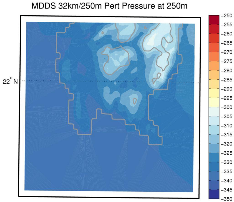
圖 3-26 MDDS 核三廠第三層巢狀網格(250 公尺解析度)壓力擾動場
