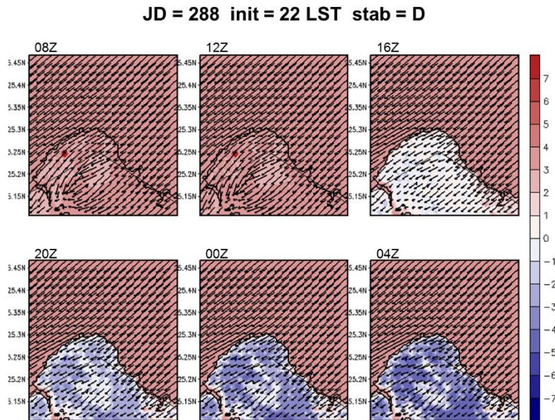
圖 5-91 A2Cflow 調校後之模擬(20m 高)風場，模擬日期太陽日為第 288 日，模擬初始時間為 20LST，中心位置為核一廠(第 3 層巢狀網格)，風向為 45^\circ ，風速為 8m/s，穩定度參數為 0.002(穩定度分類 D 級)，填色部分為溫度擾動，單位為 ^\circ\text{C} 。
