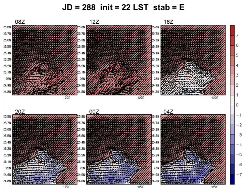
圖 5-62 A2Cflow 調校後之模擬(20m 高)風場，模擬日期太陽日為第 288 日，模擬初始時間為 22LST，中心位置為核一廠(第 2 層巢狀網格)，風向為 45^\circ ，風速為 5m/s，穩定度參數為 0.005(穩定度分類 E 級)，填色部分為溫度擾動，單位為 ^\circ\text{C} 。
