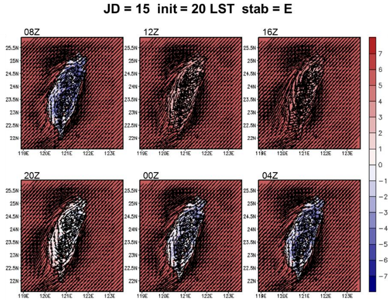
圖 5-37 A2Cflow 調校後之模擬(20m 高)風場，模擬日期太陽日為第 15 日，模擬初始時間為 20LST，中心位置為核一廠(第 1 層巢狀網格)，風向為 45^\circ ，風速為 5m/s，穩定度參數為 0.005(穩定度分類 E 級)，填色部分為溫度擾動，單位為 ^\circ\text{C} 。
