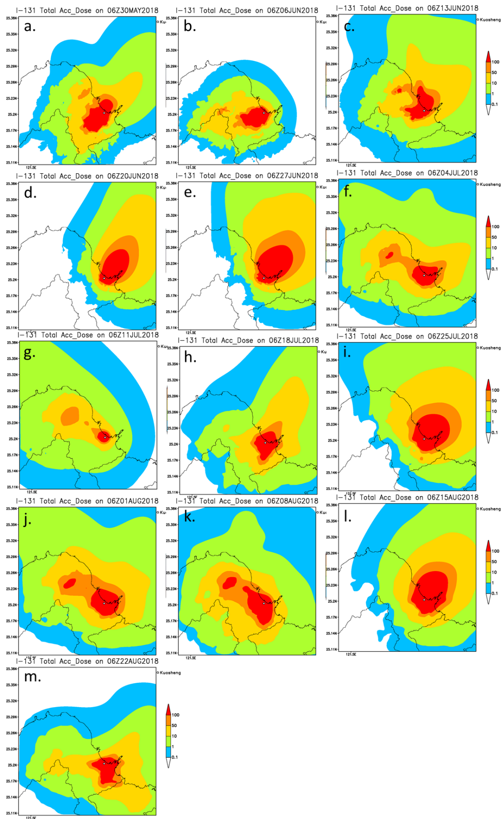
圖 4-22 核二廠夏季，自 2018 年 5 月 29 日至 2018 年 8 月 28 日 I-131 假想事故模擬之 7 日有效劑量累積圖(mSv)。
