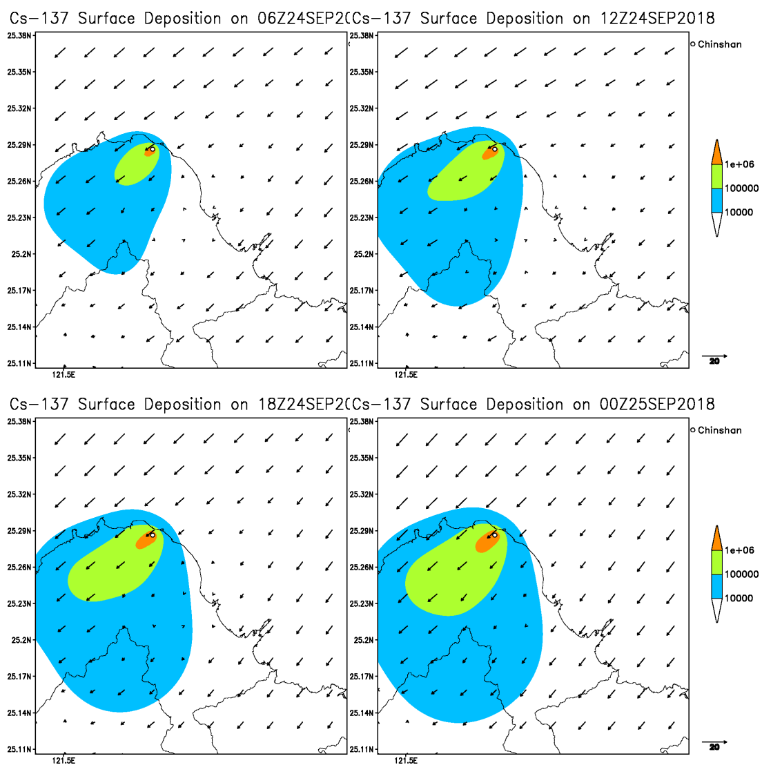
圖 3-33 2018 年 9 月 24 日僅有乾沉降過程之每六小時之地表沉降累積量( \text{Bq}/\text{m}^2 )分布。
