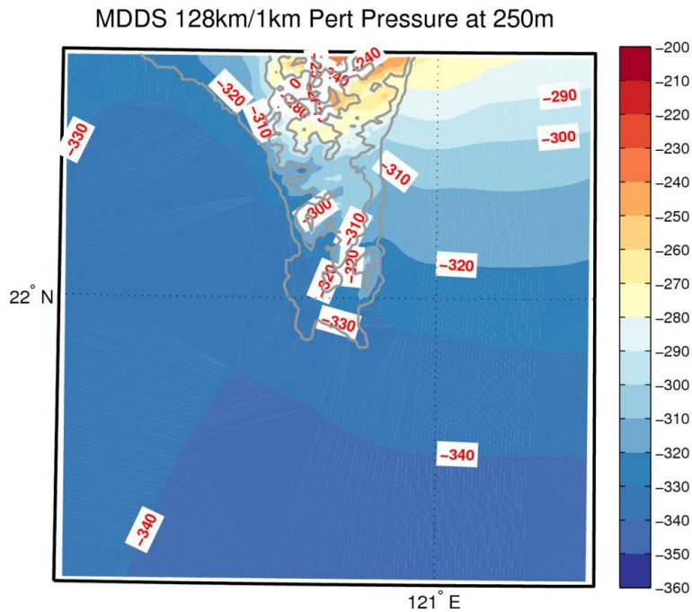
圖 3-24 MDDS 核三廠第一層巢狀網格(1 公里解析度)壓力擾動場。此時大氣環境中最主要受到冷高壓影響，壓力擾動場由北而南是由高到低且梯度較大，可以看到隨著解析度的增加，越能解析出壓力場在地形上面的變化。
