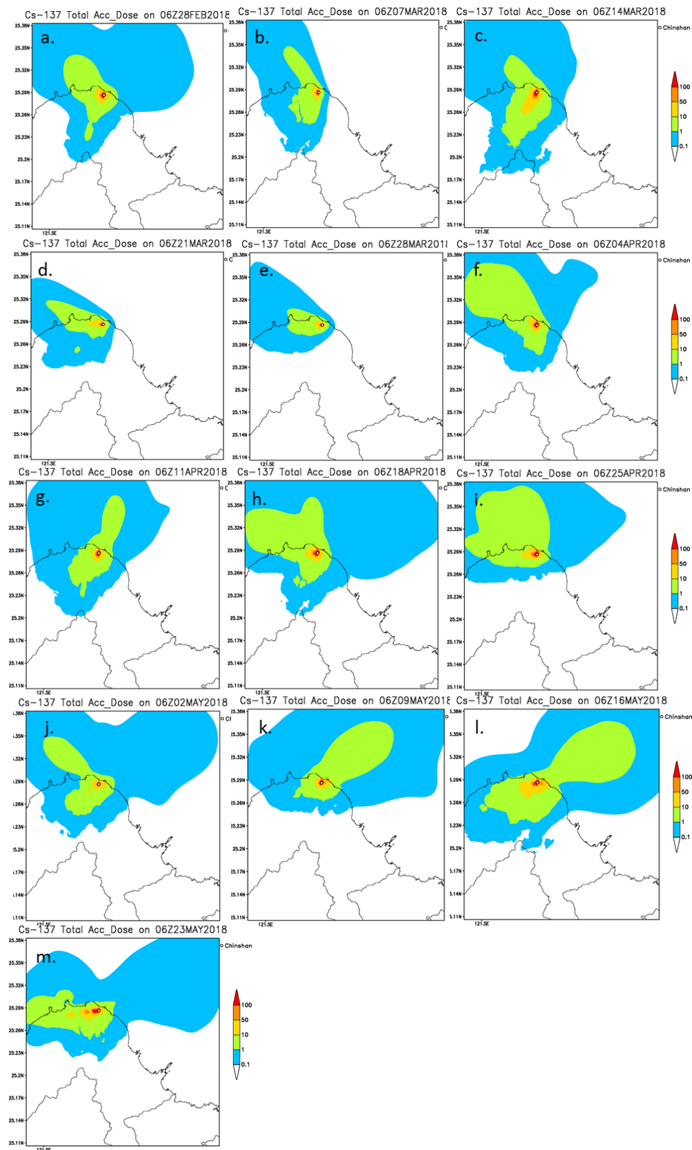
圖 4-12 核一廠春季，自 2018 年 2 月 28 日至 2018 年 5 月 23 日 Cs-137 假想事故模擬之 7 日有效劑量累積圖(mSv)。
