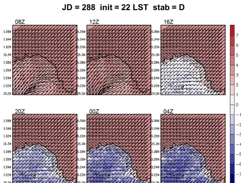
圖 5-60 A2Cflow 調校後之模擬(20m 高)風場，模擬日期太陽日為第 288 日，模擬初始時間為 22LST，中心位置為核一廠(第 4 層巢狀網格)，風向為 45^\circ ，風速為 5m/s，穩定度參數為 0.002(穩定度分類 D 級)，填色部分為溫度擾動，單位為 ^\circ\text{C} 。
