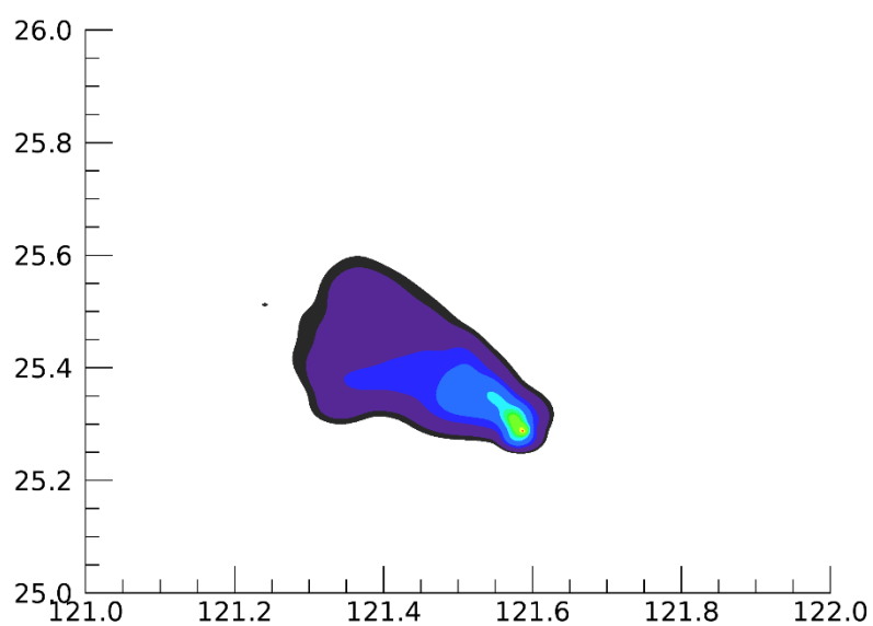
圖 3-4 核一廠案例不同劑量網格設定輸出結果 2
