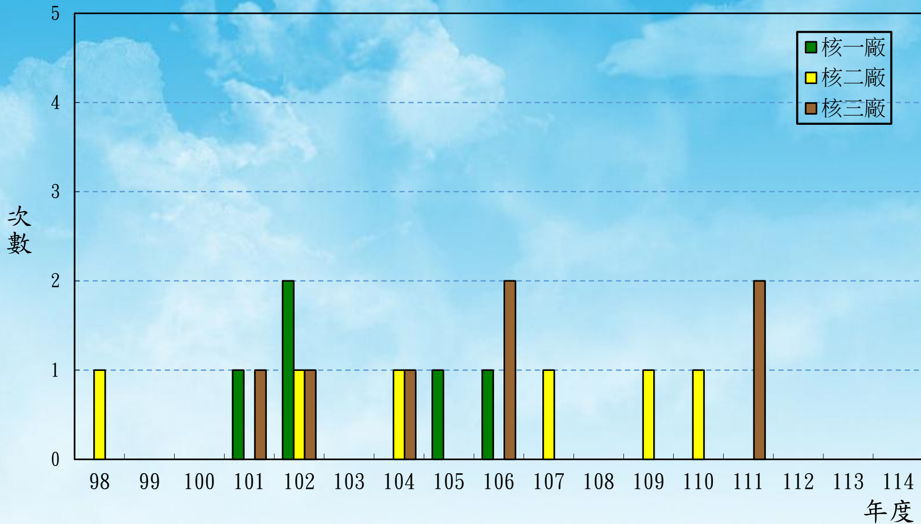
我國核能電廠自動急停次數統計圖
